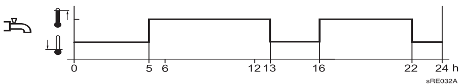
Abb 17: Freigabe nach Zeitschaltprogramm 4 (Beispiel)
