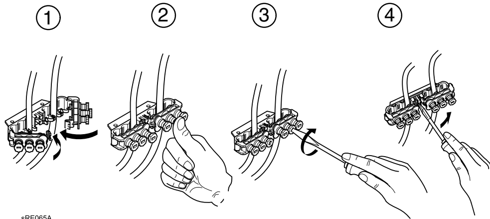
Abb 9: Zugentlastung
