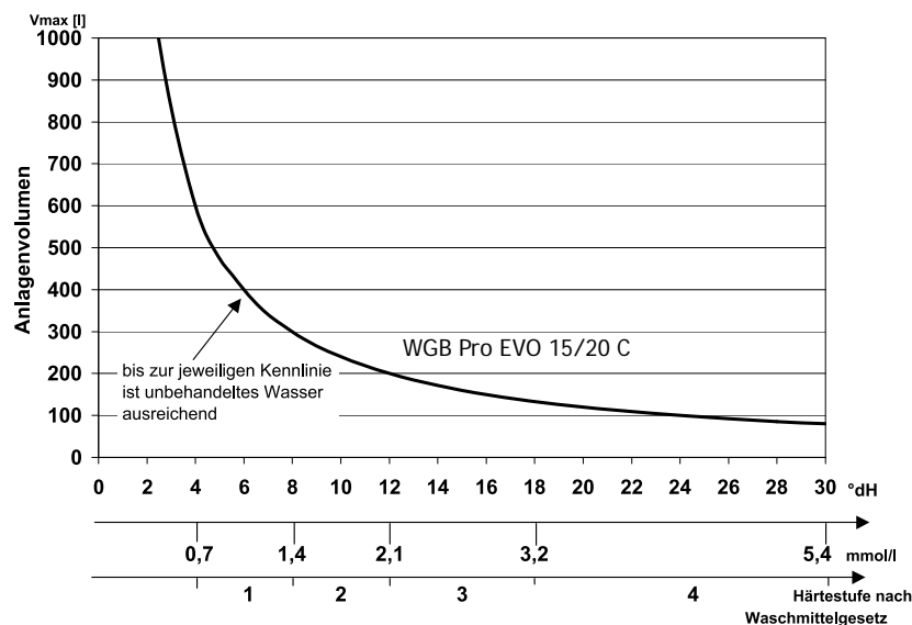
Abb 2: Diagramm Wasserhärte
