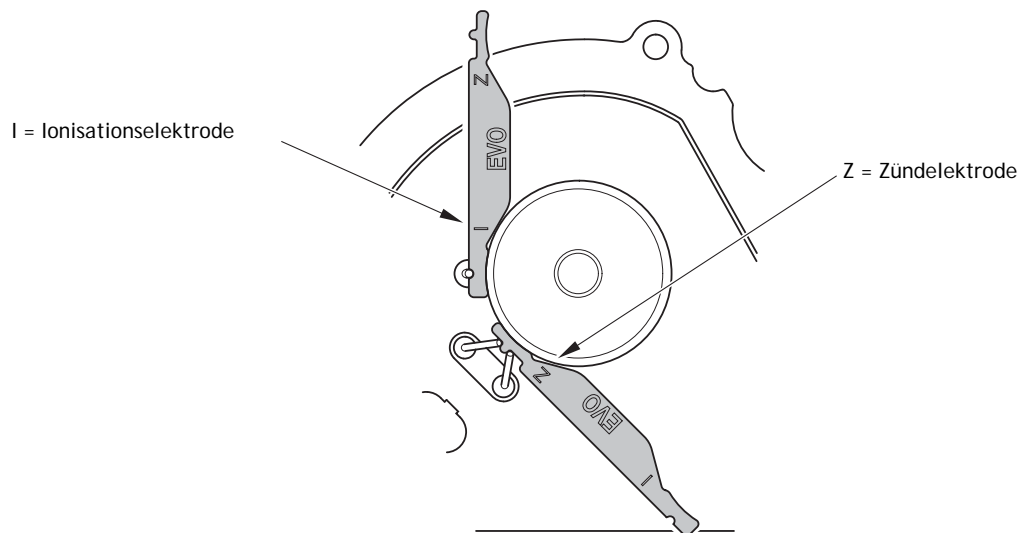
Abb 24: Prüfung der Elektrodenabstände
