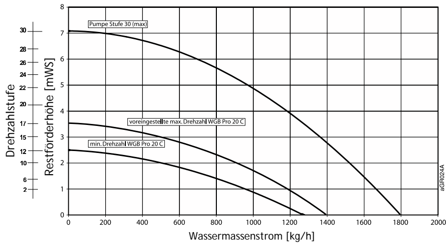
Abb 15: Restförderhöhe
