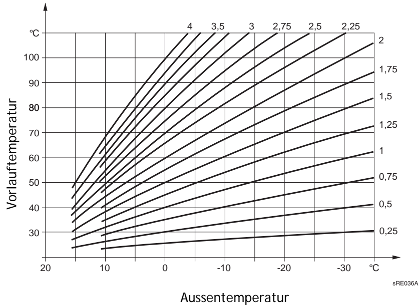
Abb 13: Heizkennlinien-Diagramm
