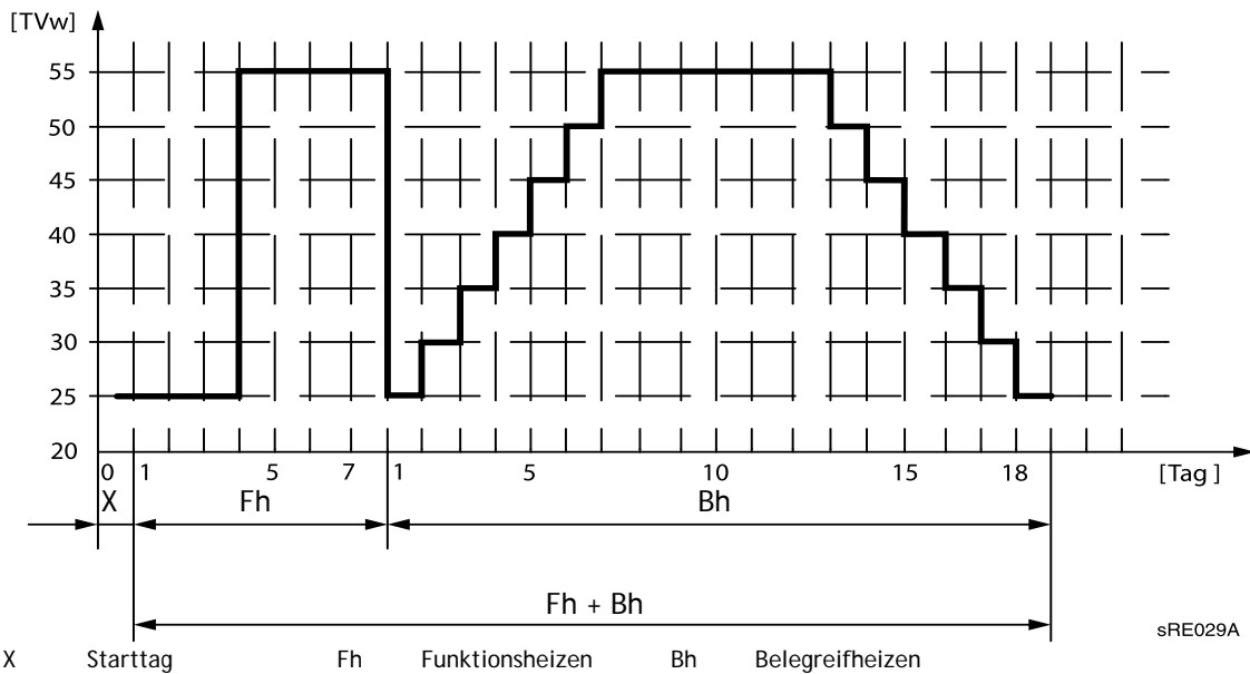
Abb 14: Temperaturprofil bei der Estrich-Austrocknungsfunktion
