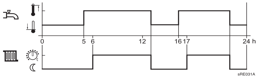
Abb 16: Freigabe in Abhängigkeit von den Zeitschaltprogrammen der Heizkreise (Beispiel)
