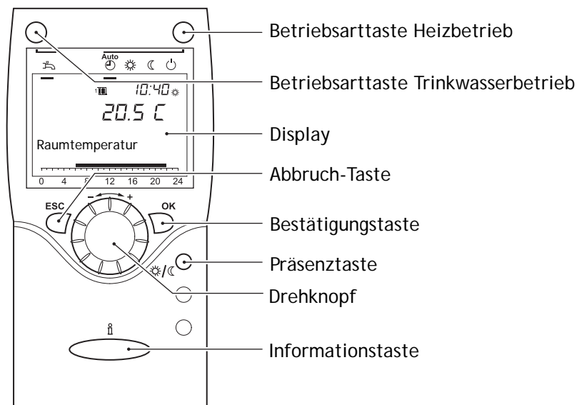
Abb. 20: Bedieneroberfläche der Raumgeräte RGT
