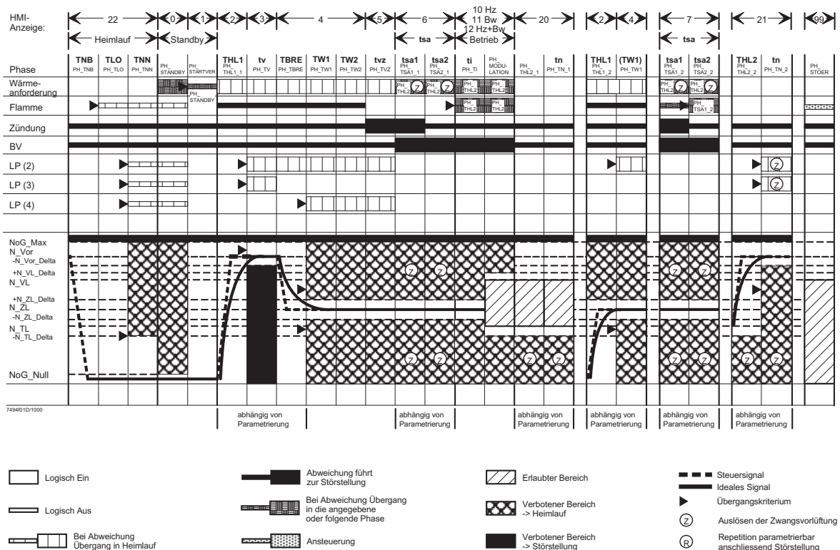
Abb 16: Programmablauf Steuer- und Regelzentrale BMU (Typ LMU 54/64.xxx)
