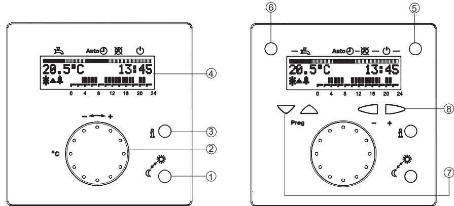
Abb 13: Raumregelgerät RRG (Zubehör)
