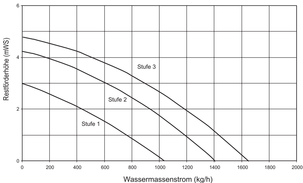
Abb 11: Restförderhöhe WBC 22/24
