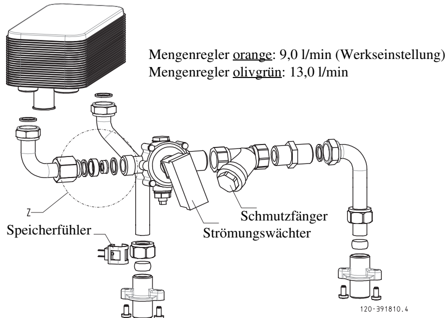
Abb 4: Austausch des Mengenreglers
