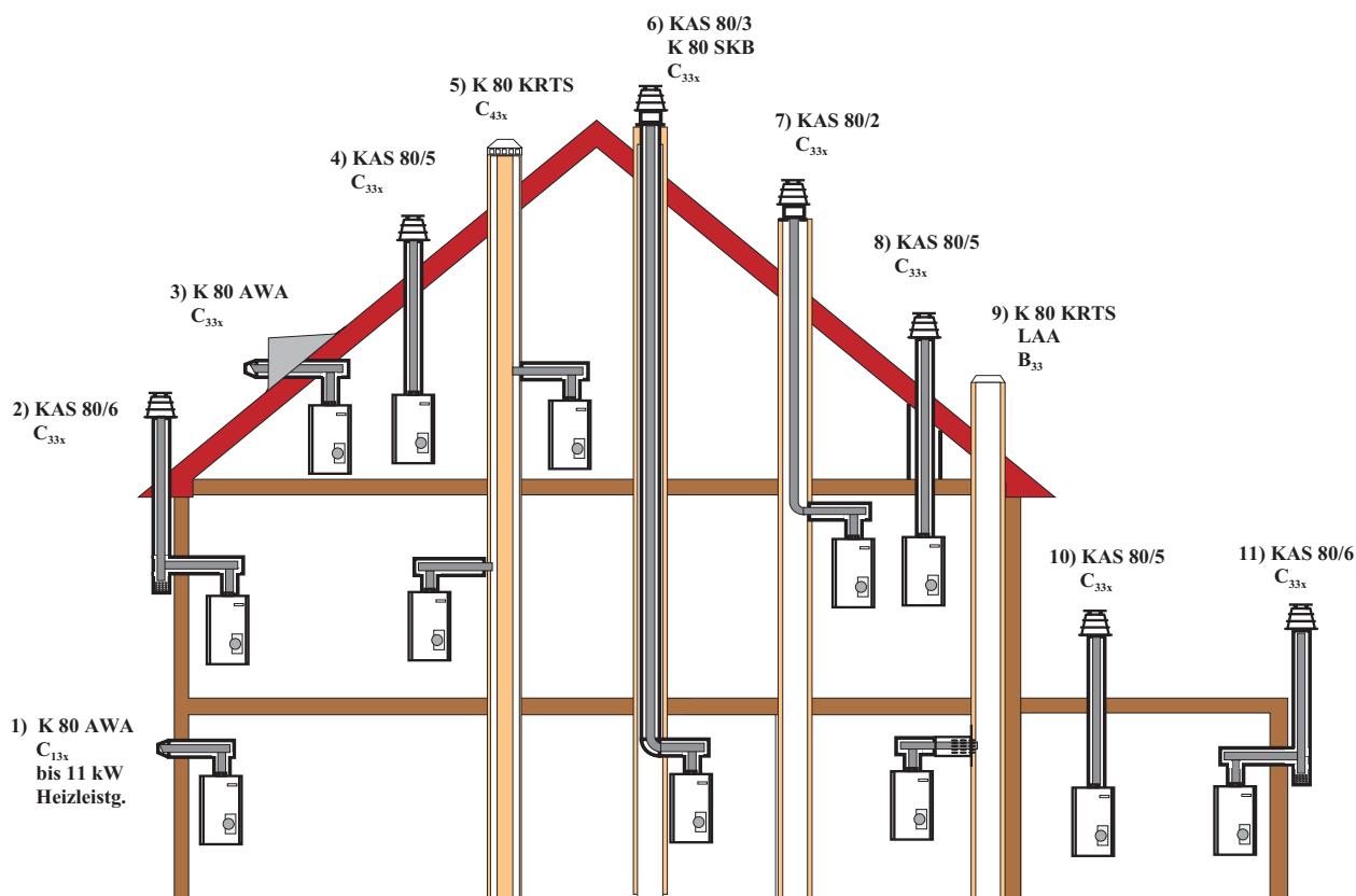
Abb 5: Anschlussmöglichkeiten mit KAS 80 (Zubehör)
