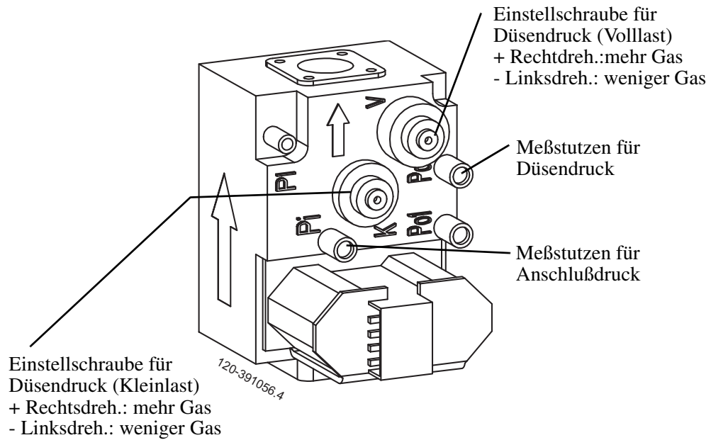
Abb 9: Gasarmatur (Einstellung der Düsendrücke mit Innensechskantschlüssel SW 2,5)
