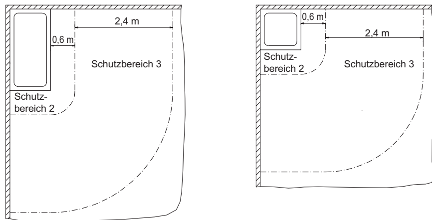
Abb 3: Abstände WBC in Bad- bzw. Duschräumen
