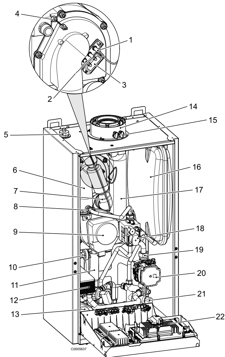
Abb. 27: Kesselansicht WBC (dargestellt ohne Vorderwand und Abdeckung der Regelung)
