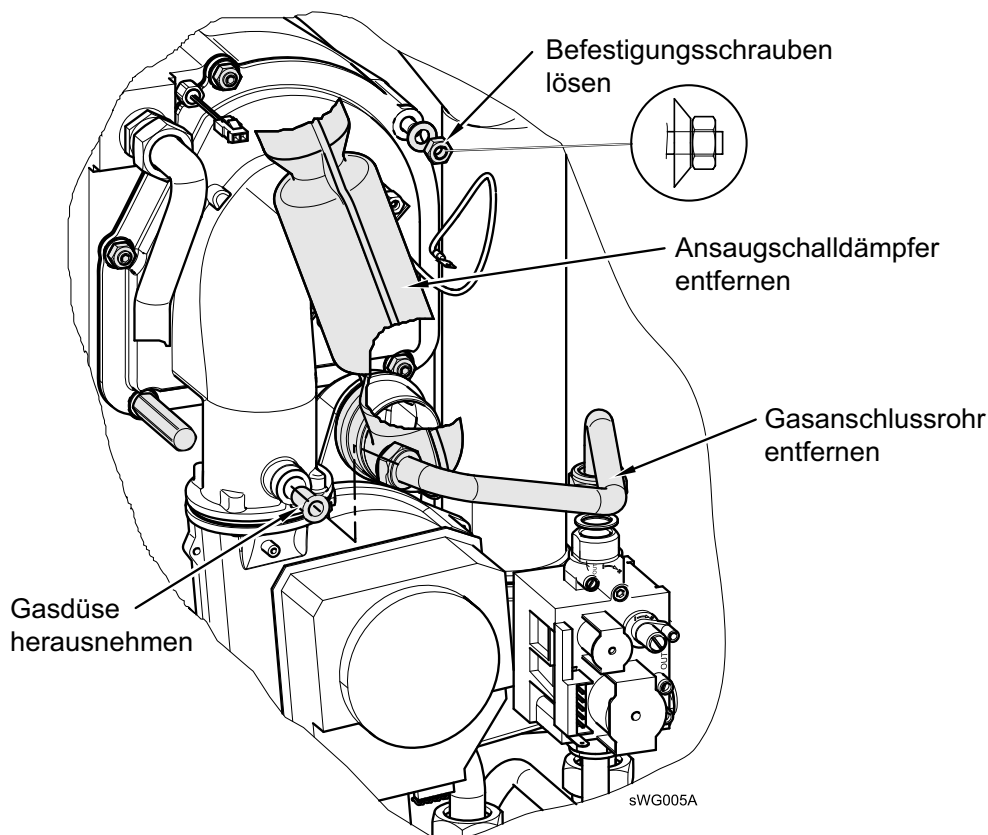
Abb. 26: Gasbrenner ausbauen
