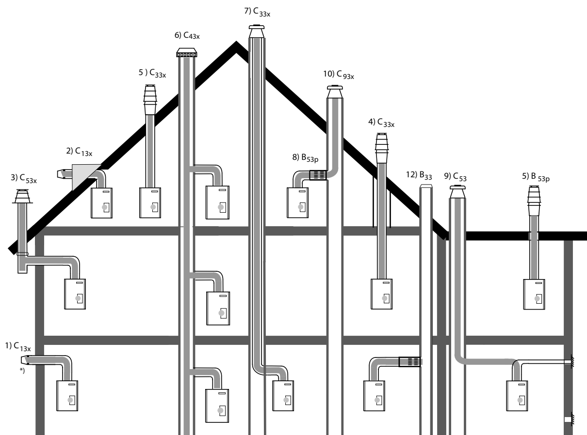
Abb. 7: Anschlussmöglichkeiten mit KAS (Zubehör)
