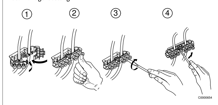
Abb. 11: Zugentlastung
