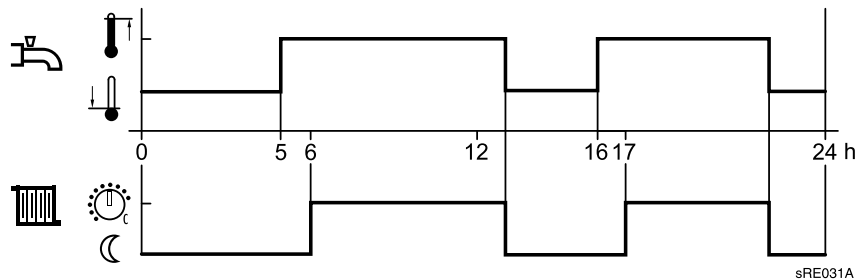
Abb. 22: Freigabe in Abhängigkeit von den Zeitschaltprogrammen der Heizkreise (Beispiel)
