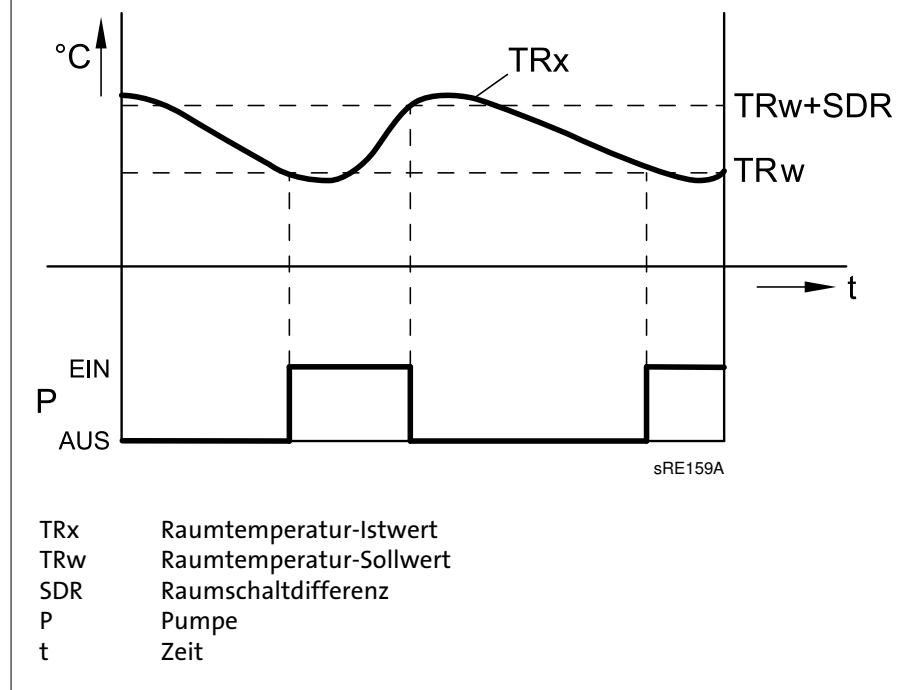
Abb. 16: Raumtemperaturbegrenzung
