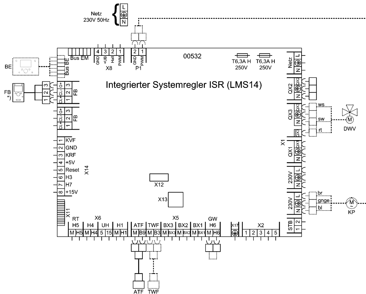
Abb. 5: Anschlussplan
