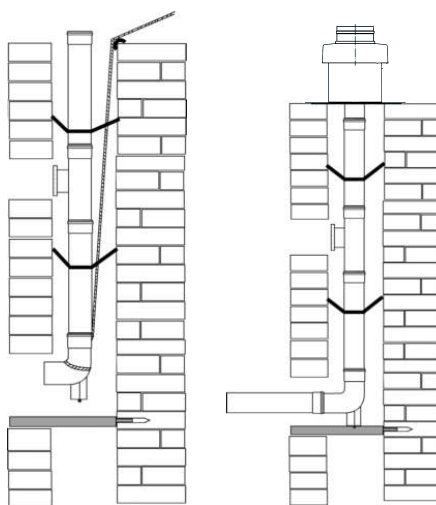
Abb. 9: Einführen in einen Schacht
