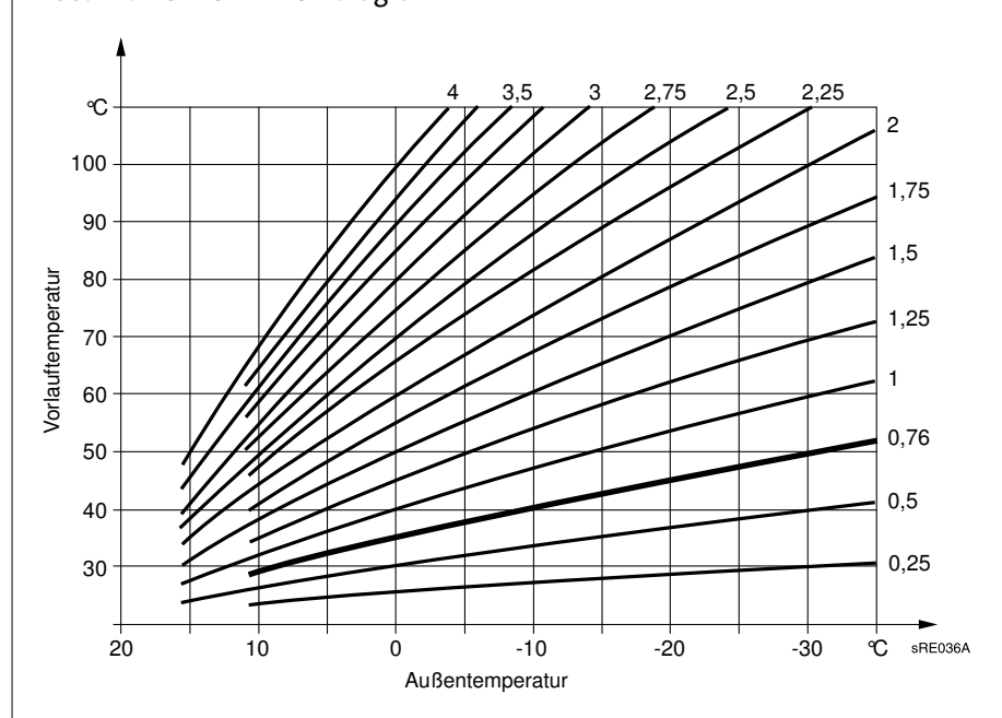
Abb. 14: Heizkennlinien-Diagramm
