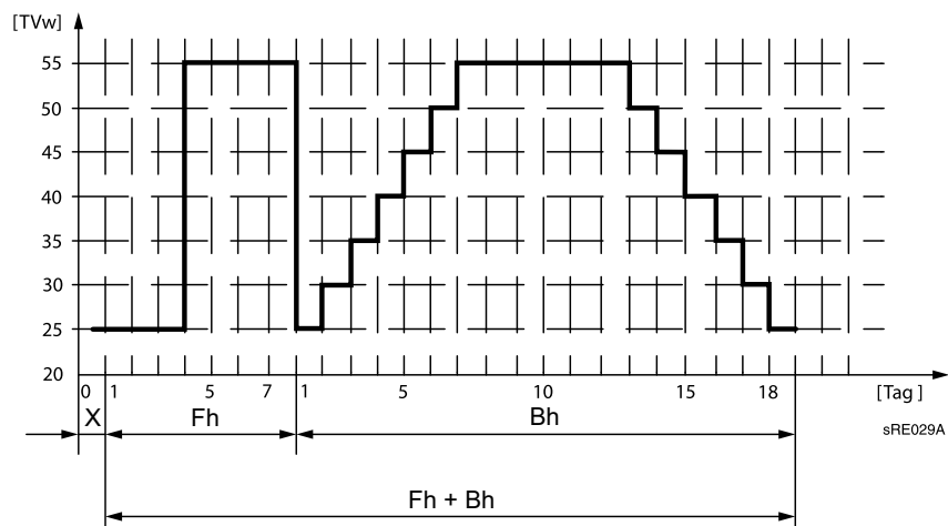
Abb. 20: Temperaturprofil bei der Estrich-Austrocknungsfunktion
