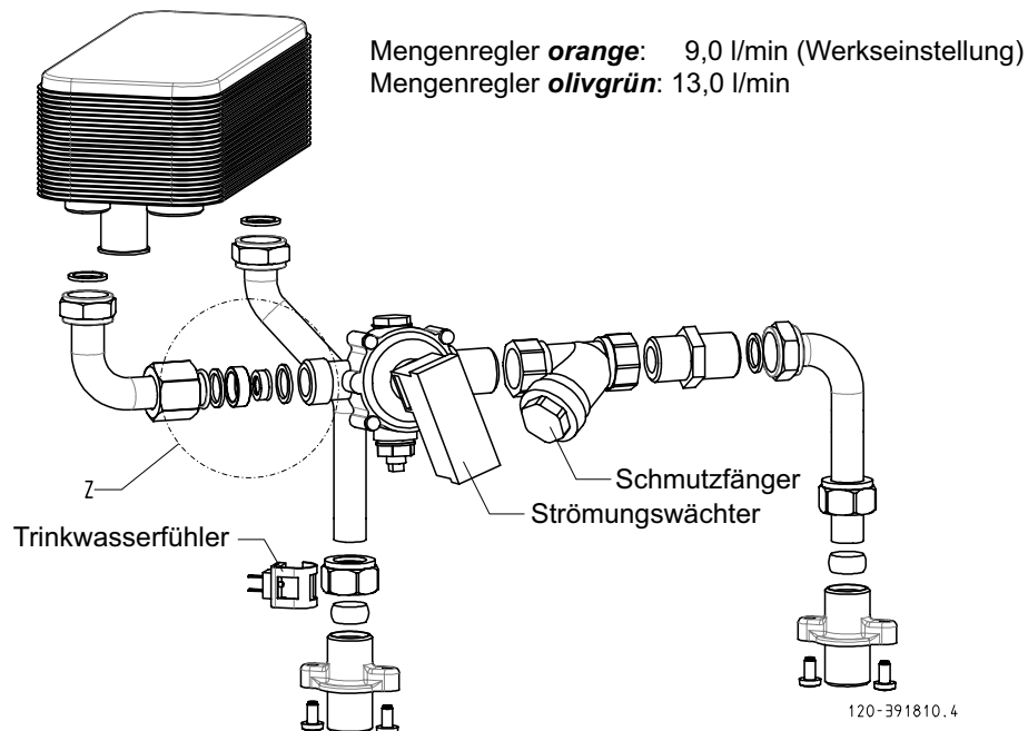
Abb. 6: Austausch des Mengenreglers
