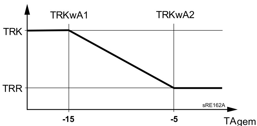
Abb. 19: Reduziert-Anhebung
