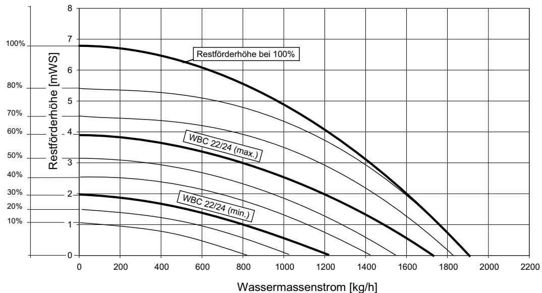
Abb. 21: Restförderhöhe WBC 22/24 F
