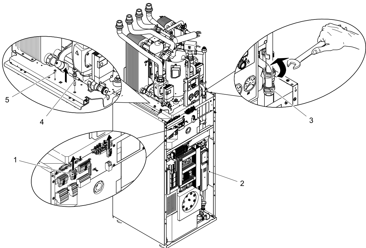
Abb. 25: Vorbereitung zum Transport des Geräteoberteils
