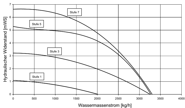
Abb. 5: Restförderhöhe Verdampferseite BSW-K/-KC 6
