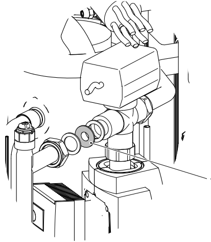
Abb. 28: Warmwasserblende ausbauen
