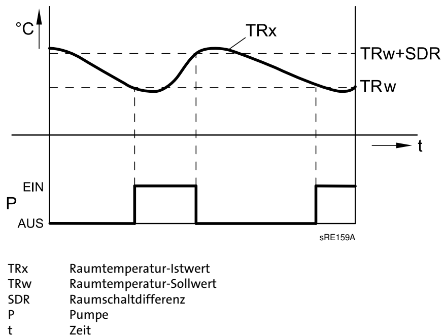
Abb. 36: Raumtemperaturbegrenzung
