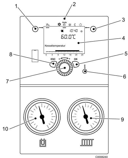
Abb. 32: Bedienelemente
