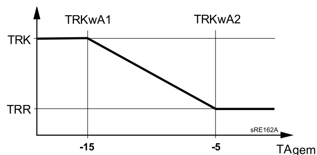
Abb. 39: Reduziert-Anhebung
