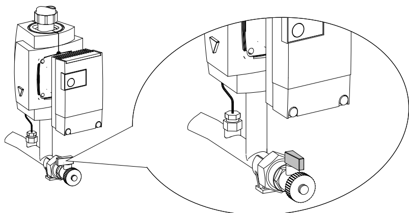
Abb. 48: Heizkreispumpe ausbauen
