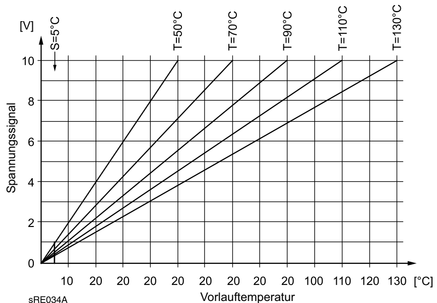
Abb. 46: Wärmeanforderung (Beispiele)
