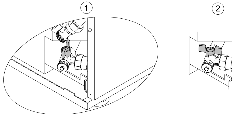
Abb. 29: Entleerungshahn Trinkwasser-Speicher
