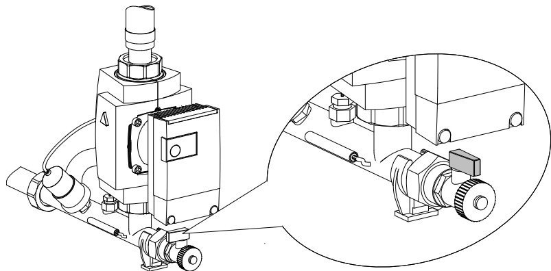
Abb. 47: Solepumpe ausbauen
