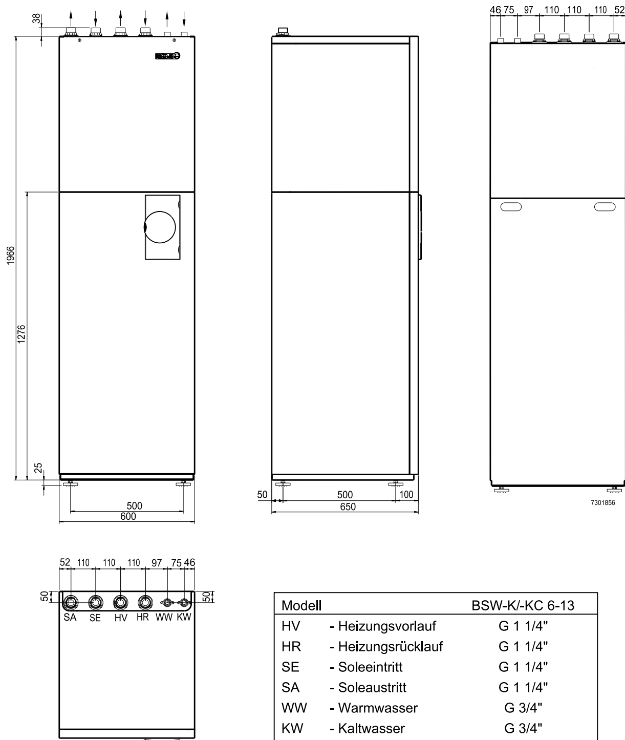
Abb. 1: Abmessungen und Anschlüsse BSW-K/-KC 6-13
