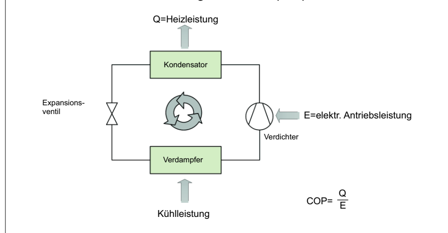
Abb. 14: Schematische Darstellung einer Wärmepumpe
