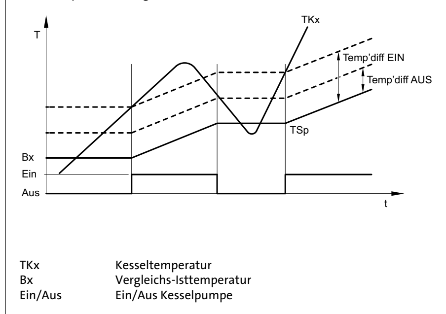
Abb. 44: Speicherladung
