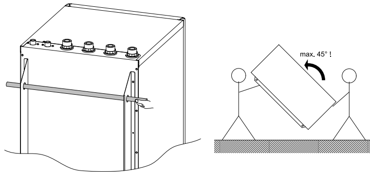
Abb. 13: Transporthilfe
