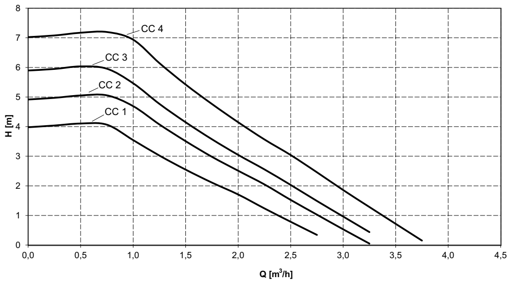
Abb. 17: Diagramm BOB 32/40 B mit integriertem Heizkreispumpen-Set HPS BOB 32/40
