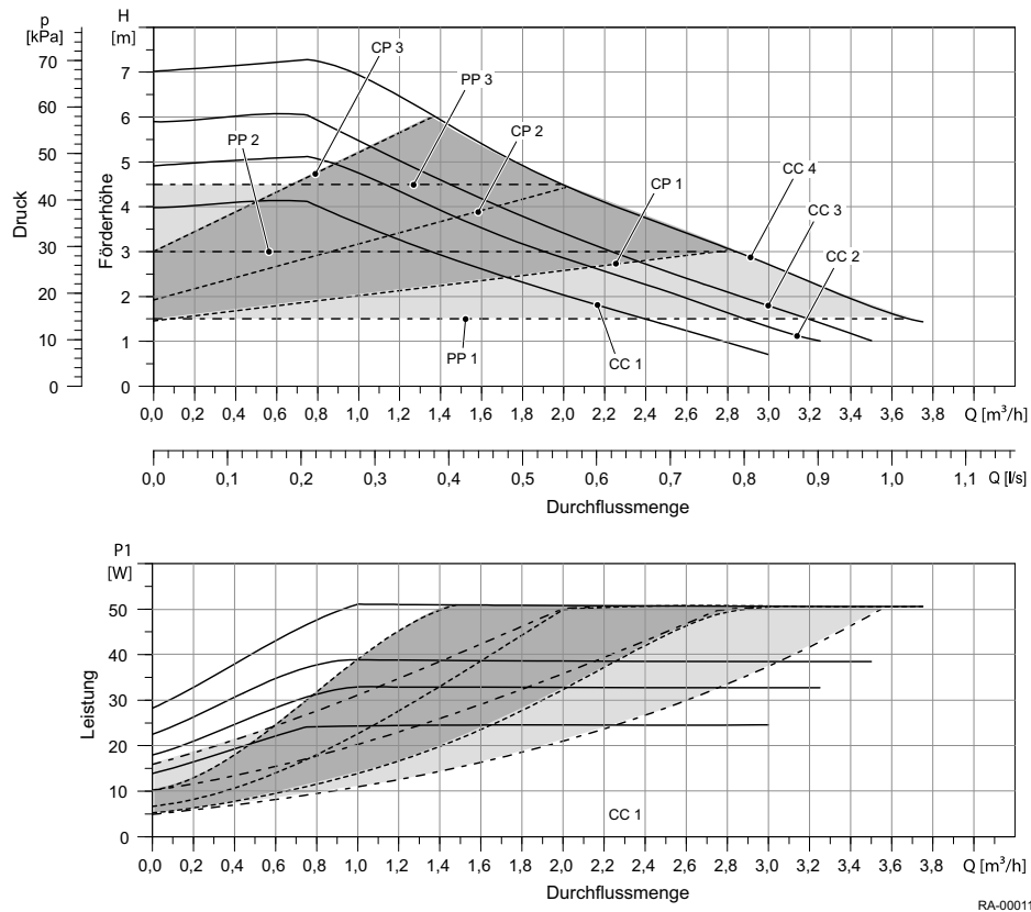
Abb. 23: Pumpenkennlinien Grundfos UPM3 (PSG B /PSMG B )
