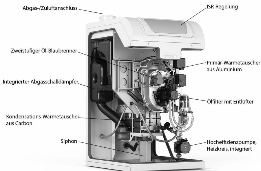
Abb. 3: Aufbau und Funktion BOB 20/25 B
