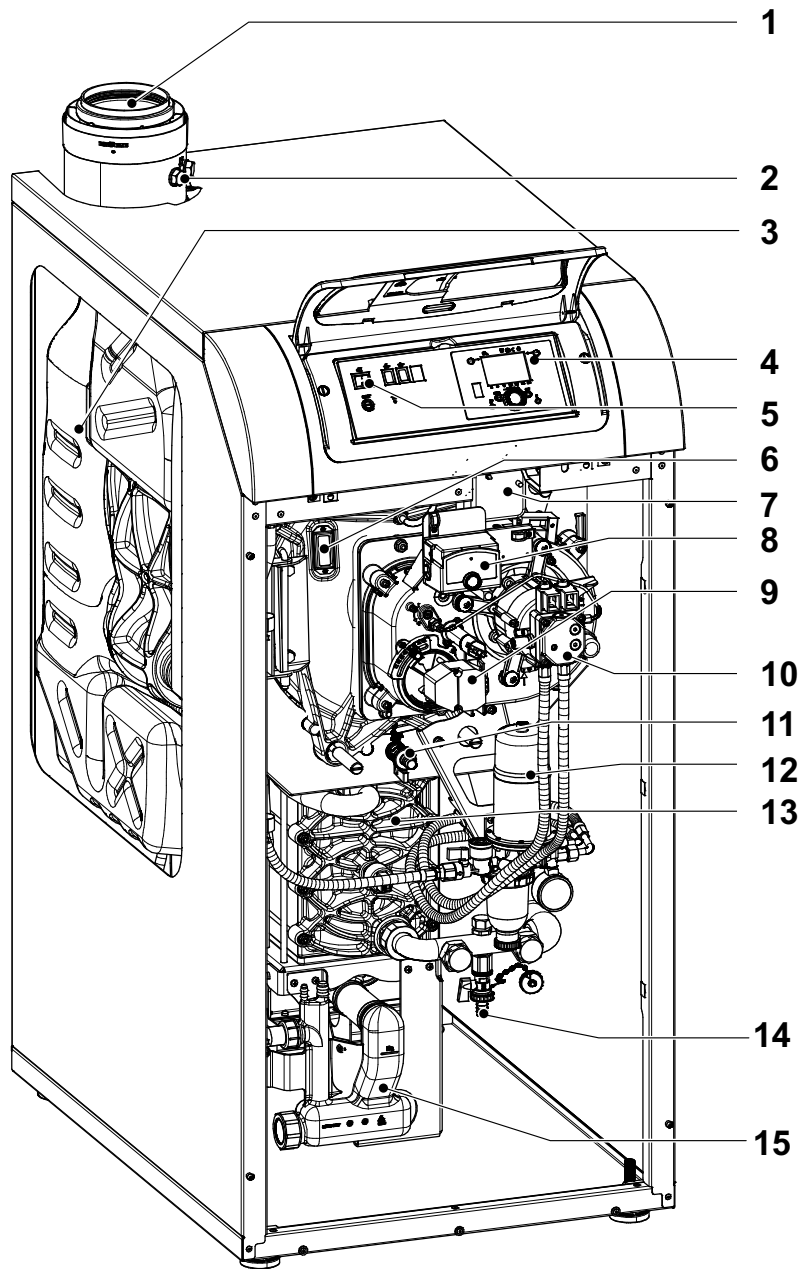
Abb. 2: BOB 32–40 B (dargestellt ohne Frontverkleidung)
