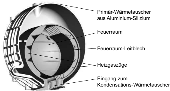
Abb. 4: Primär-Wärmetauscher
