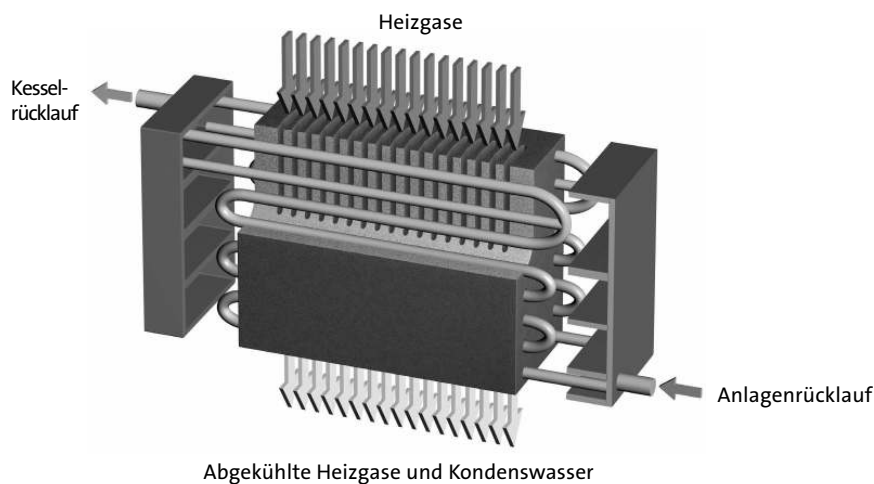
Abb. 7: Effektive Wärmeübertragung im Kreuzstrom-Prinzip
