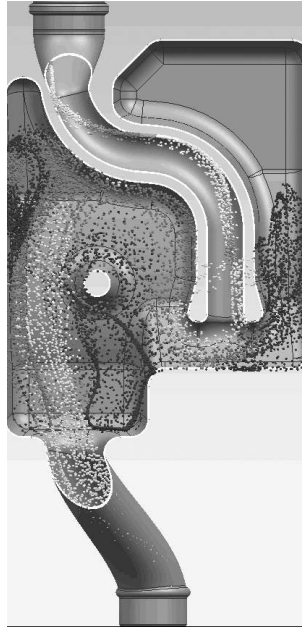
Abb. 8: Strömungssimulation Schalldämpfer
