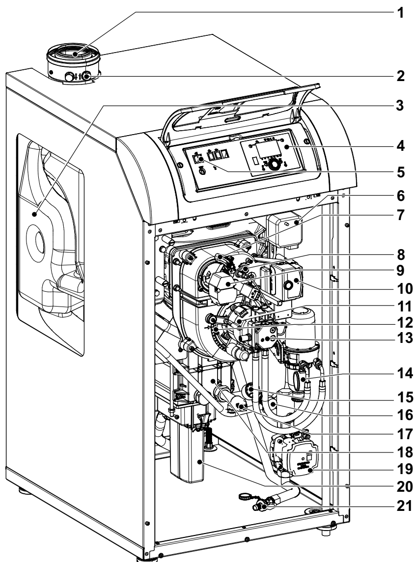
Abb. 1: BOB 20–25 B (dargestellt ohne Frontverkleidung)
