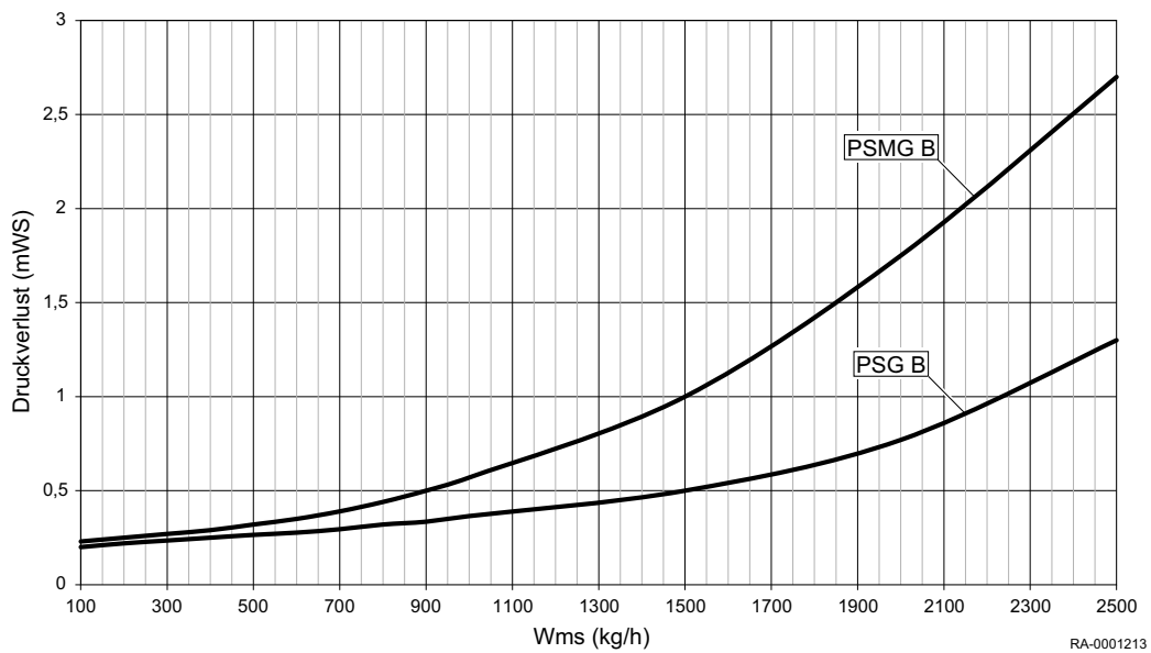
Abb. 24: Druckverlustkurven PSG B /PSMG B
