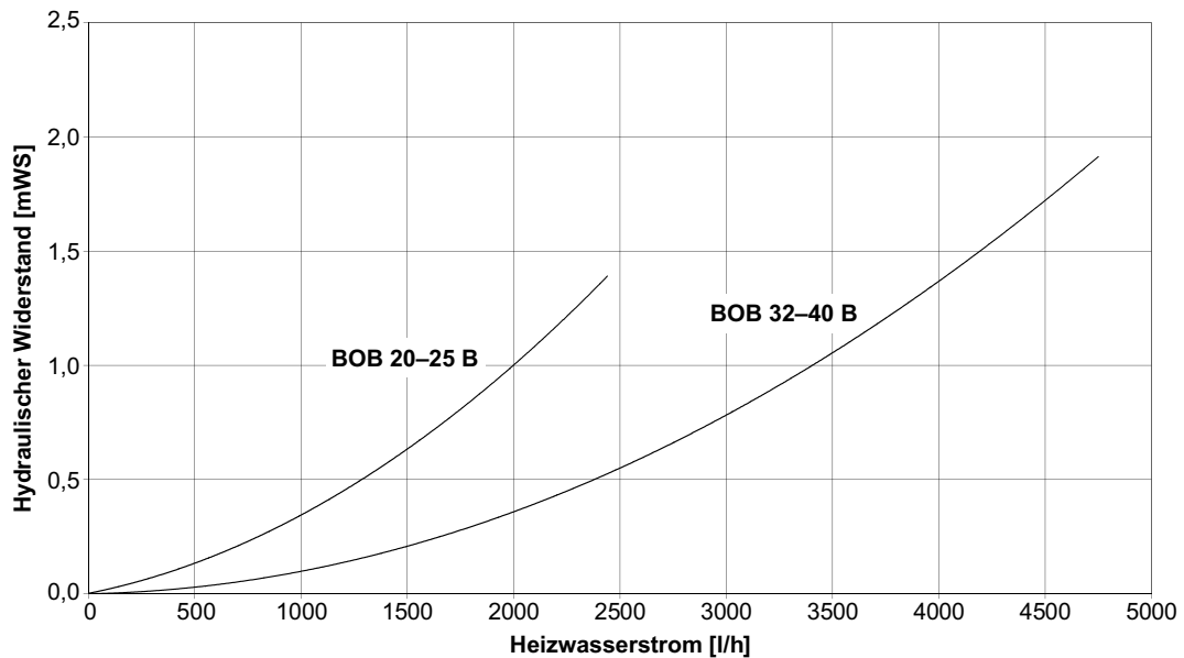
Abb. 18: Diagramm BOB 20–40 B (ohne Schwerkraftbremse)
