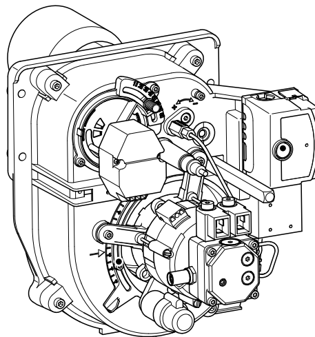
Abb. 9: Zweistufiger Öl-Blaubrenner
