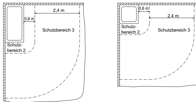
Abb. 3: Abstände in Bad- bzw. Duschräumen
