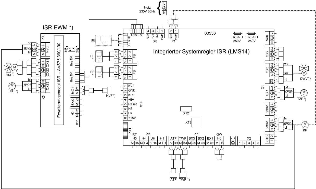
Abb. 7: Anschlussplan
