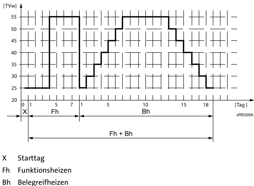
Abb. 24: Temperaturprofil bei der Estrich-Austrocknungsfunktion
