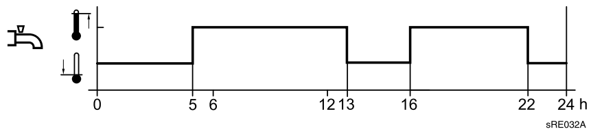
Abb. 27: Freigabe nach Zeitschaltprogramm 4 (Beispiel)
