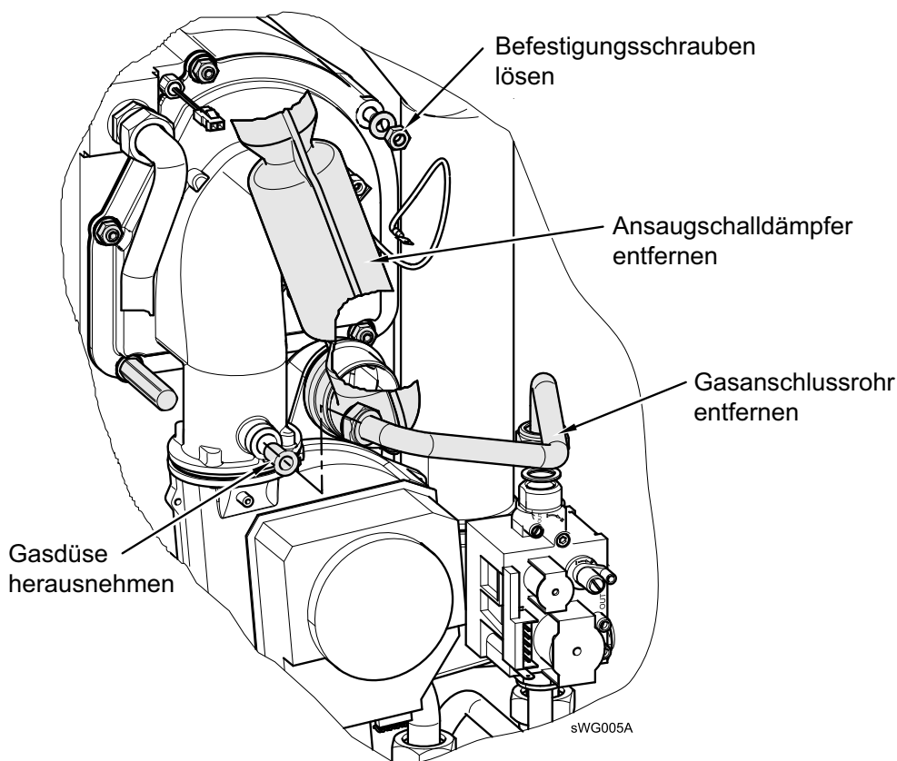
Abb. 31: Gasbrenner ausbauen
