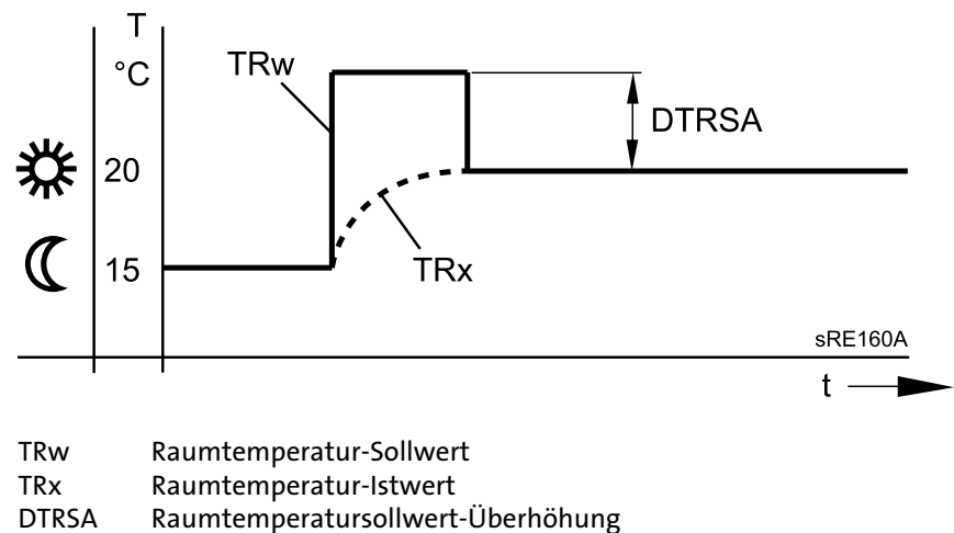
Abb. 21: Schnellaufheizung
