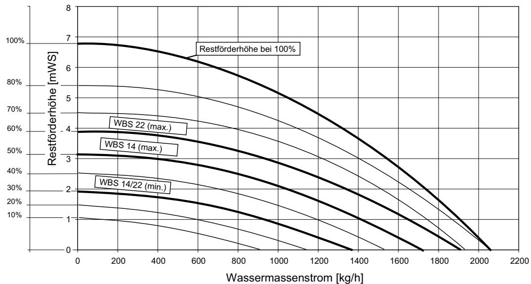
Abb. 25: Restförderhöhe WBS 14/22 F
