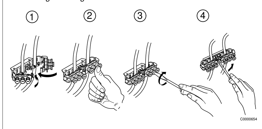
Abb. 15: Zugentlastung
