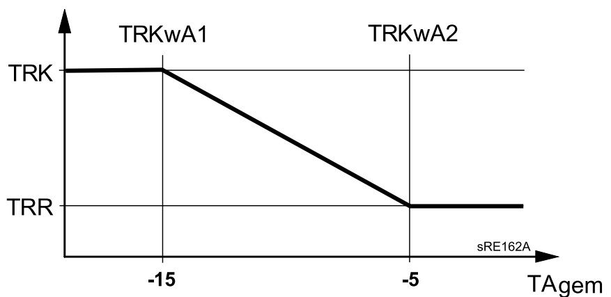
Abb. 23: Reduziert-Anhebung
