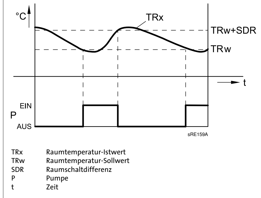
Abb. 20: Raumtemperaturbegrenzung
