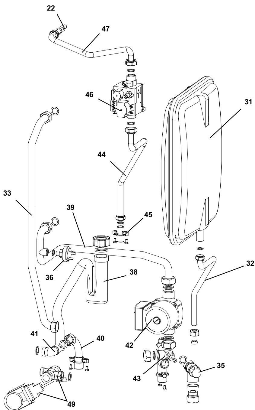
Abb. 36: Verrohrungsbauteile
