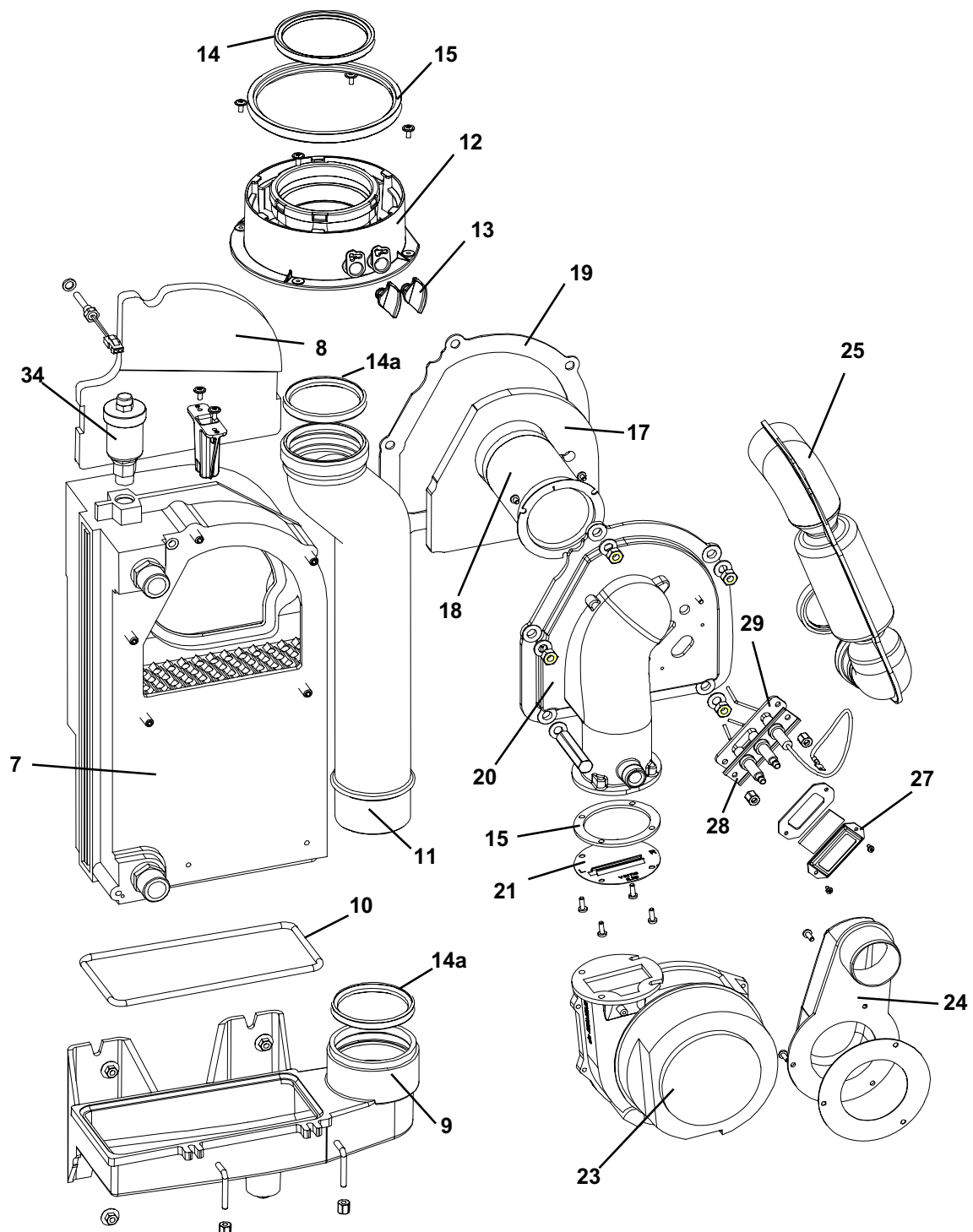
Abb. 35: Brennerbauteile
