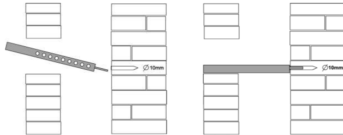
Abb. 11: Montage der Stützschiene
