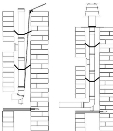
Abb. 12: Einführen in einen Schacht
