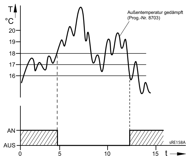
Abb. 19: Sommer-/Winterheizgrenze
