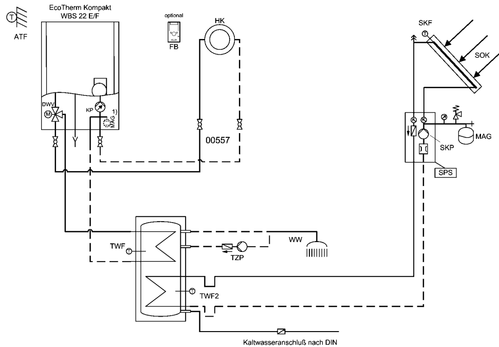
Abb. 8: Anwendungsbeispiel: Ein Pumpenheizkreis mit Raumgerät und Solarspeicher
