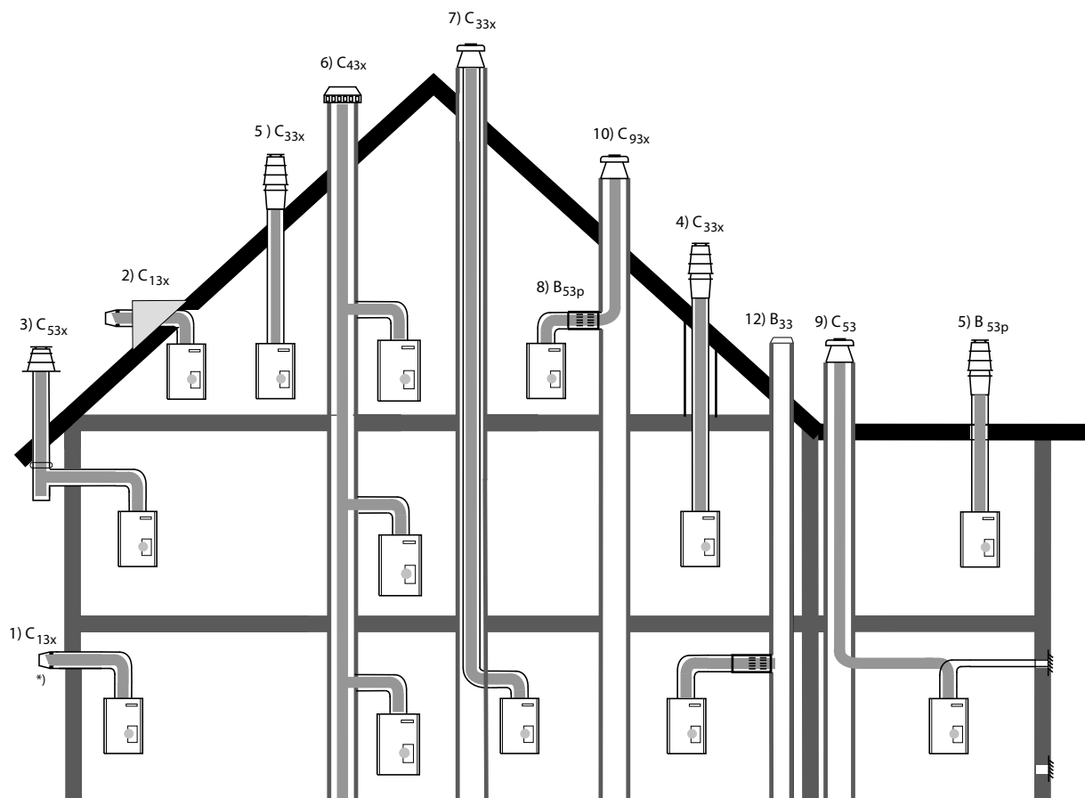
Abb. 7: Anschlussmöglichkeiten mit KAS (Zubehör)
