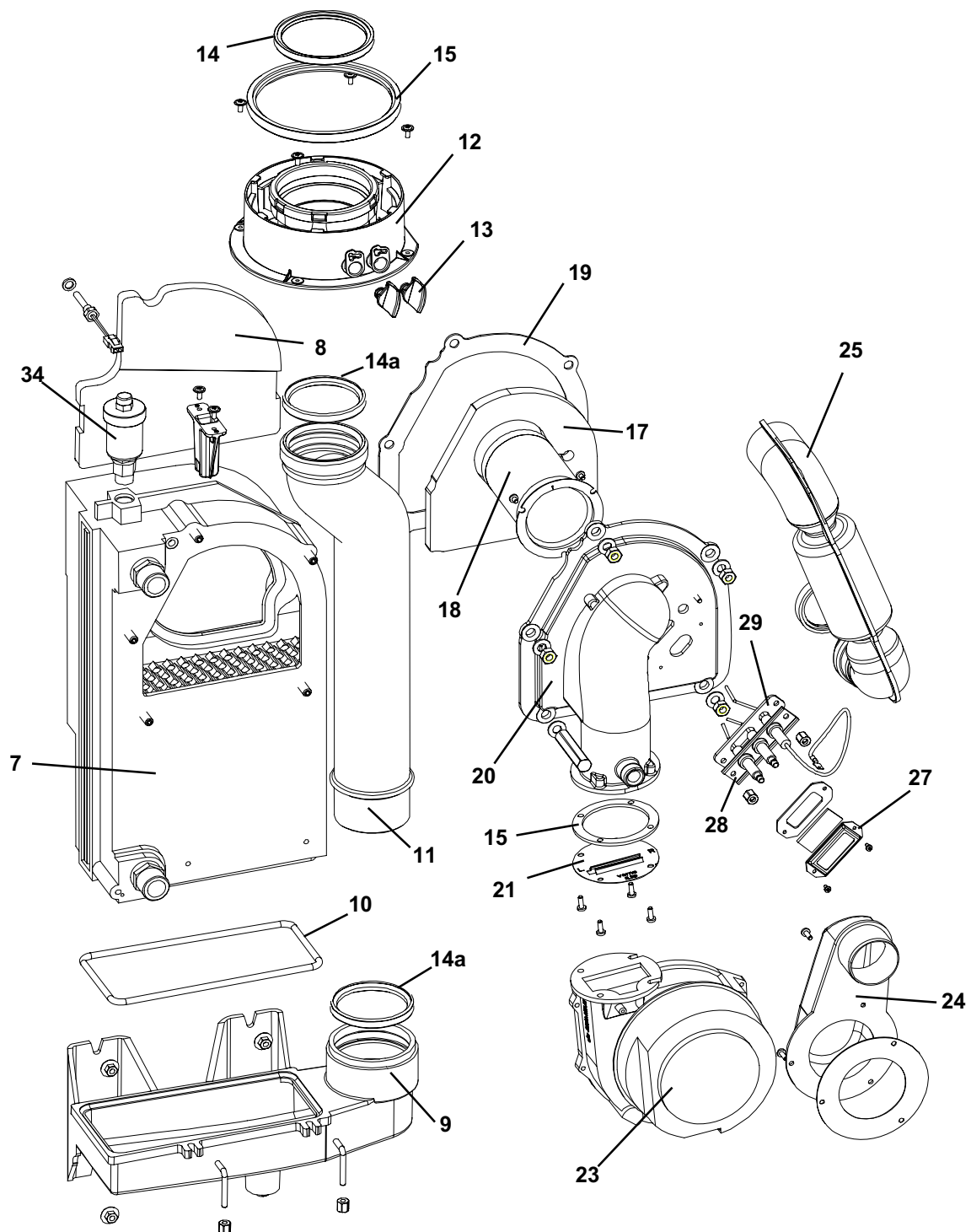
Abb. 30: Brennerbauteile
