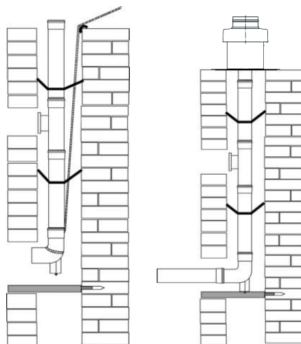
Abb. 9: Einführen in einen Schacht
