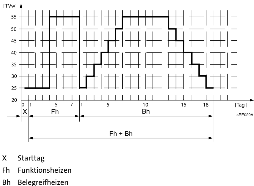
Abb. 20: Temperaturprofil bei der Estrich-Austrocknungsfunktion
