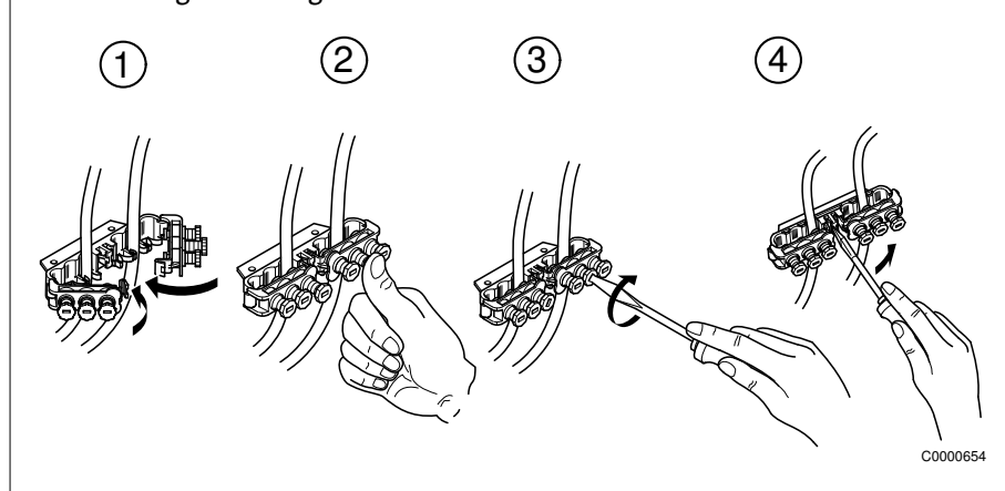
Abb. 12: Zugentlastung
