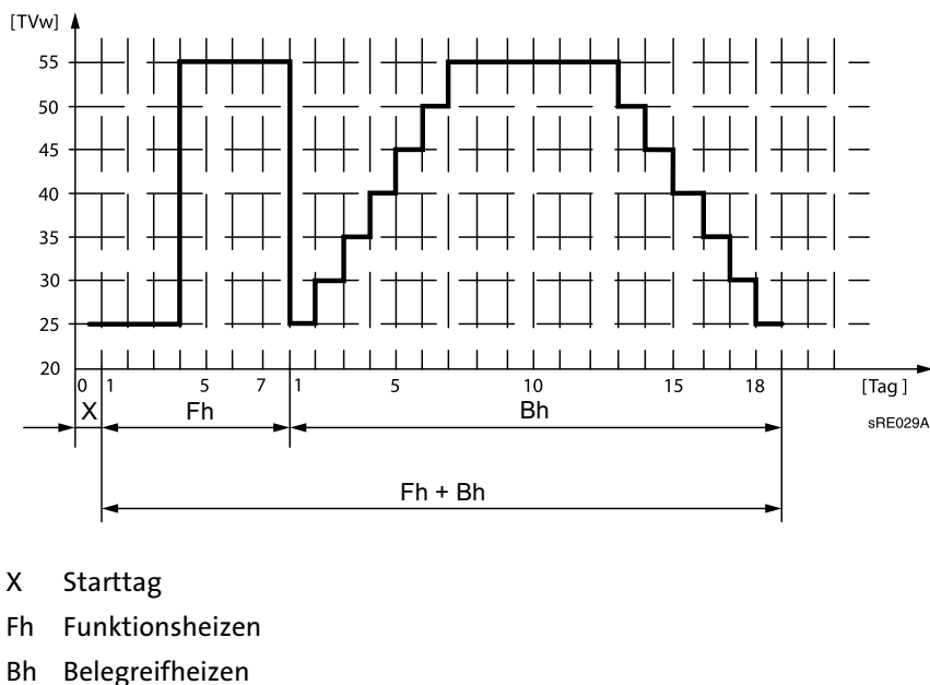
Abb. 21: Temperaturprofil bei der Estrich-Austrocknungsfunktion
