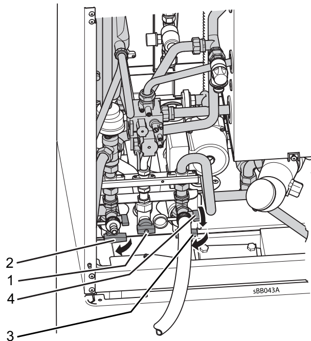
Abb. 6: Absperrventile und Gasabsperrhahn schliessen
