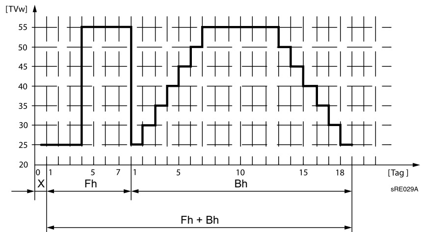
Abb. 22: Temperaturprofil bei der Estrich-Austrocknungsfunktion
