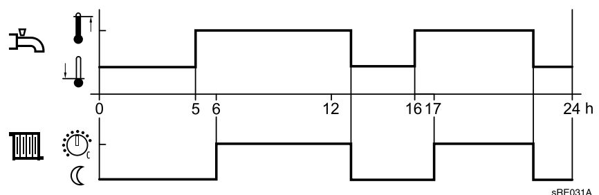
Abb. 24: Freigabe in Abhängigkeit von den Zeitschaltprogrammen der Heizkreise (Beispiel)
