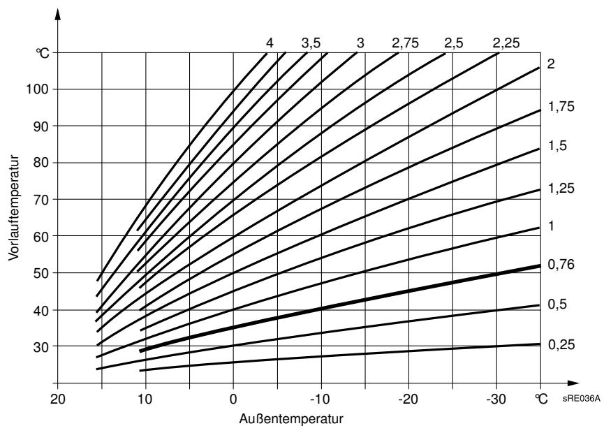
Abb. 16: Heizkennlinien-Diagramm
