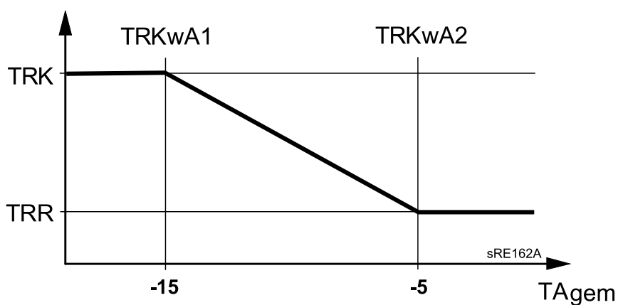
Abb. 21: Reduziert-Anhebung
