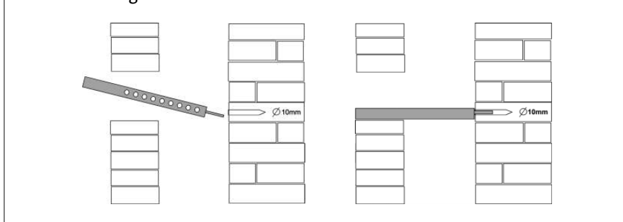
Abb. 8: Montage der Stützschiene
