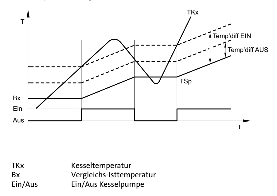
Abb. 28: Speicherladung
