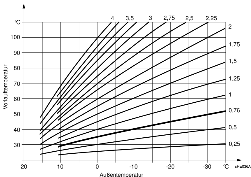
Abb. 14: Heizkennlinien-Diagramm
