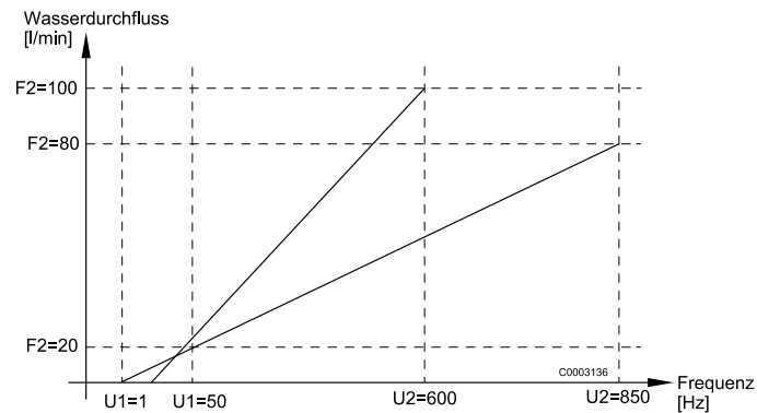
Abb. 30: Beispiel für zwei unterschiedliche Fühlerkennlinien
