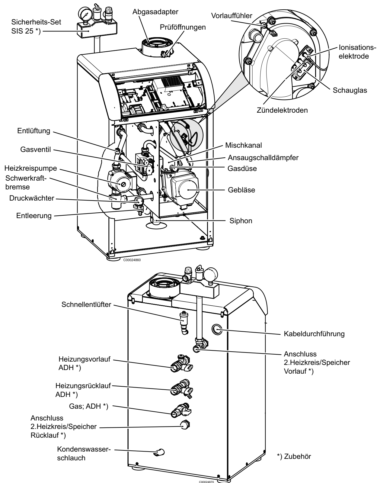
Abb. 35: Kesselansicht BGB (dargestellt ohne Vorderwand und Abdeckung der Regelung)
