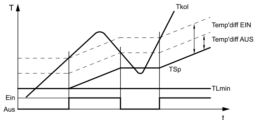
Abb. 27: Laderegelung /schematisch)
