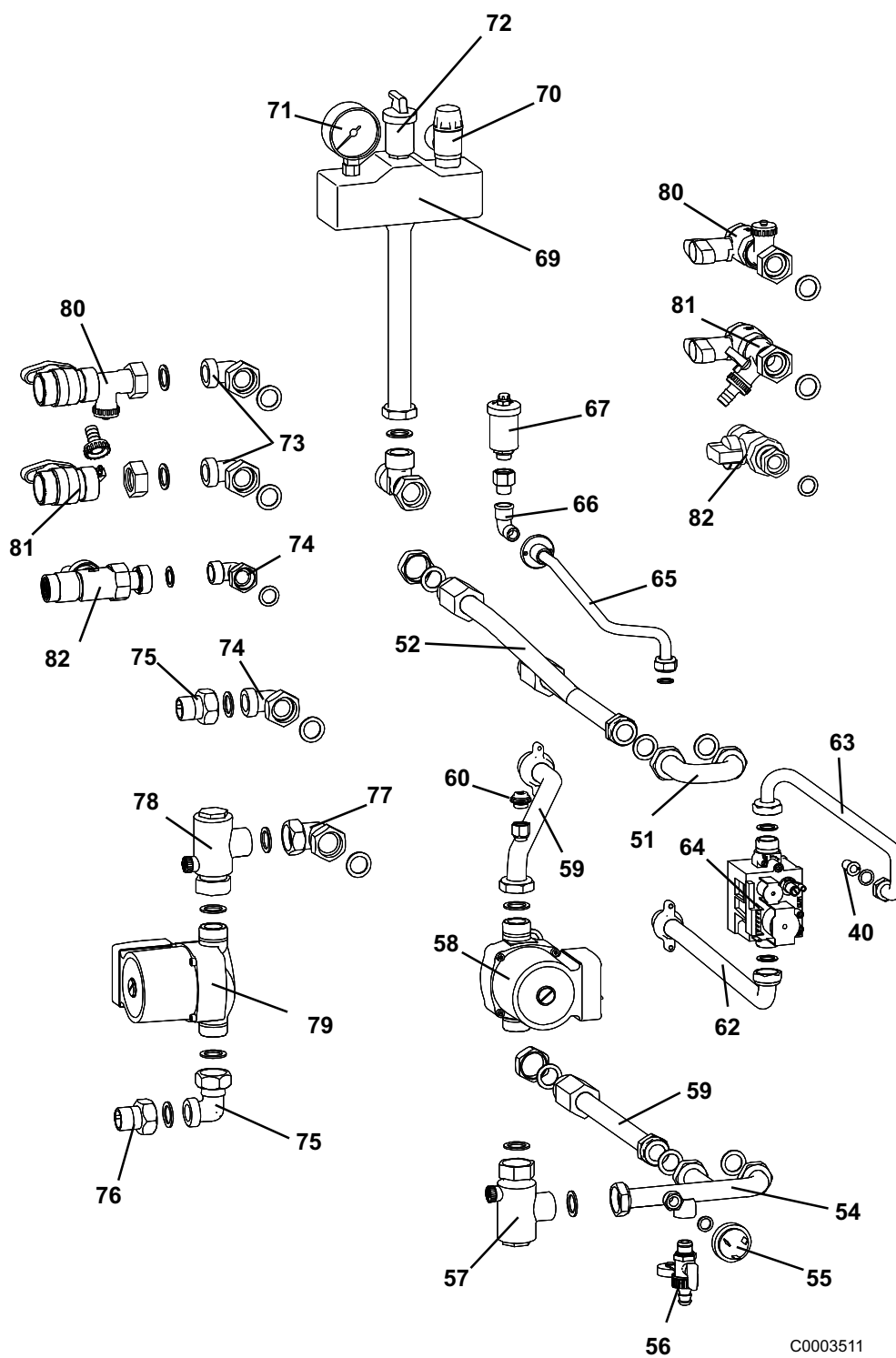
Abb. 39: Verrohrungsbauteile
