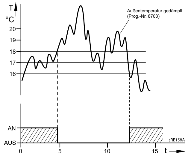
Abb. 17: Sommer-/Winterheizgrenze
