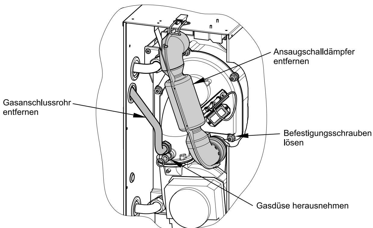
Abb. 33: Gasbrenner ausbauen
