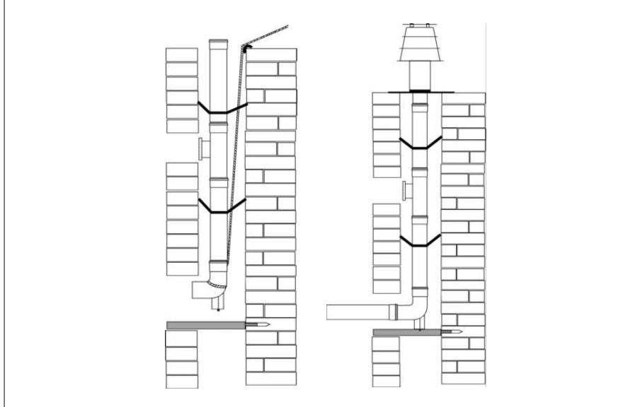
Abb. 9: Einführen in einen Schacht
