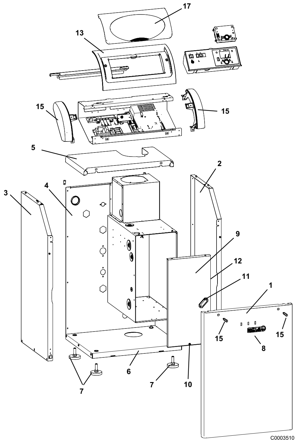
Abb. 37: Verkleidungsbauteile
