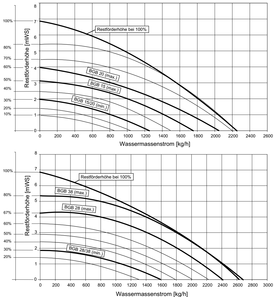
Abb. 23: Restförderhöhe BGB 15-38 E
