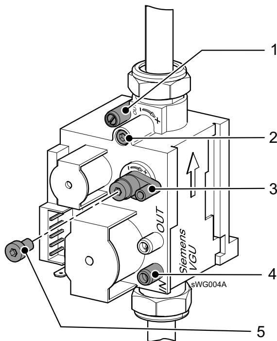
Abb. 11: Gasarmatur (Einstellung der Düsendrücke mit Torx T15)
