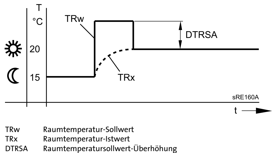
Abb. 19: Schnellaufheizung
