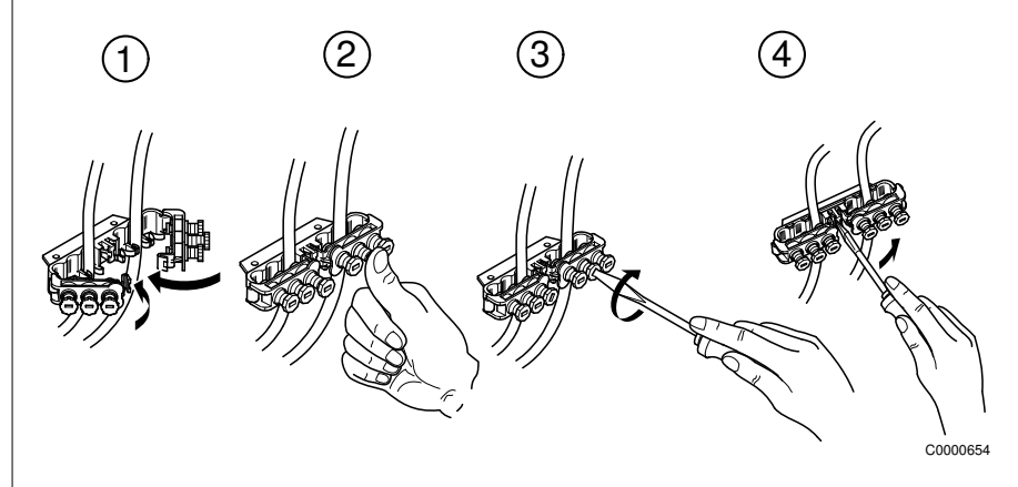
Abb. 12: Zugentlastung
