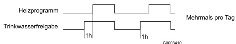
Abb. 27: Ladevorverlegung
