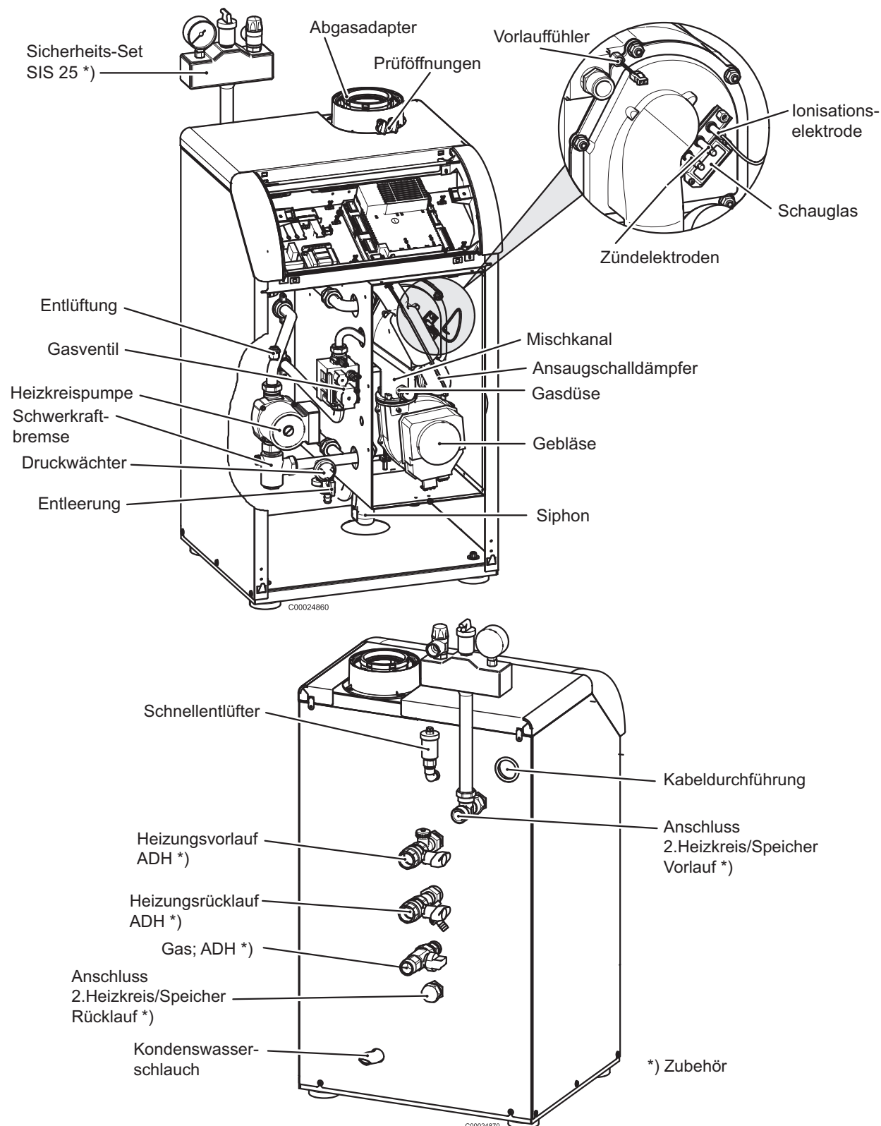
Abb. 33: Kesselansicht BGB (dargestellt ohne Vorderwand und Abdeckung der Regelung)
