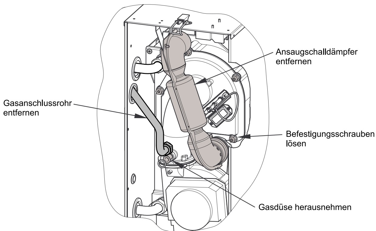
Abb. 31: Gasbrenner ausbauen
