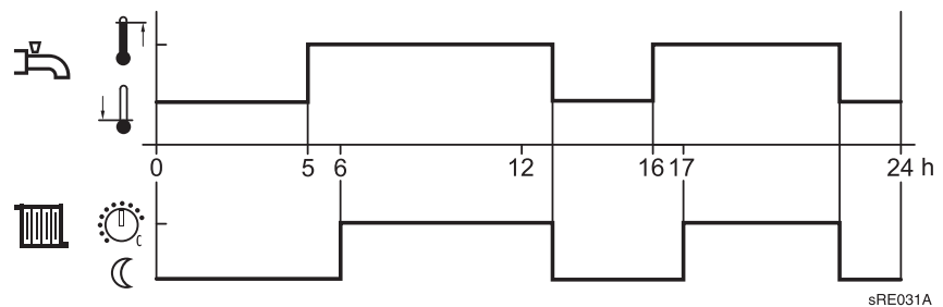
Abb. 22: Freigabe in Abhängigkeit von den Zeitschaltprogrammen der Heizkreise (Beispiel)
