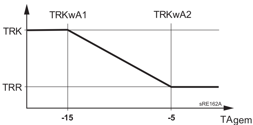
Abb. 20: Reduziert-Anhebung
