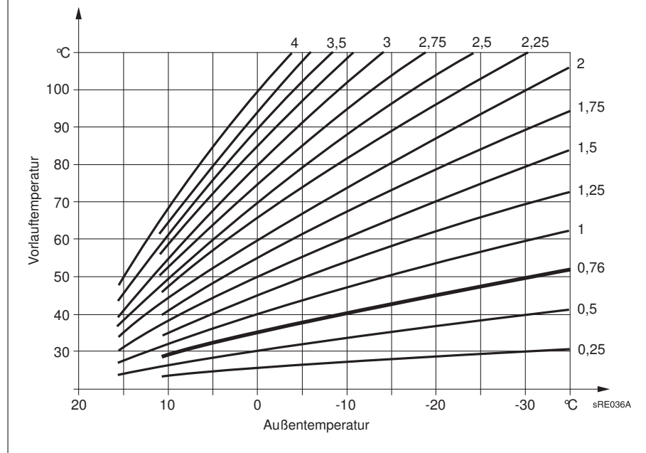
Abb. 15: Heizkennlinien-Diagramm
