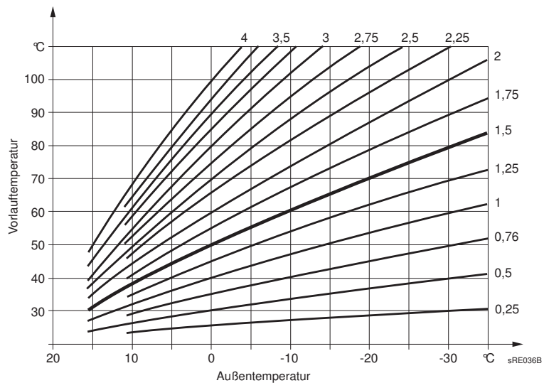
Abb. 4: Heizkennlinie
