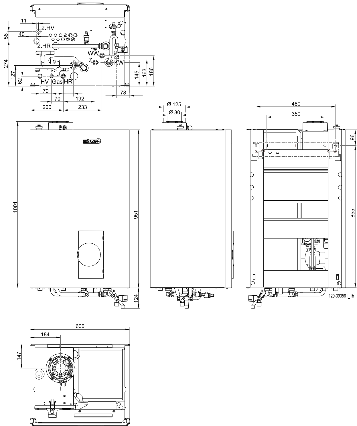
Abb. 1: Abmessungen und Anschlüsse WGB-K
