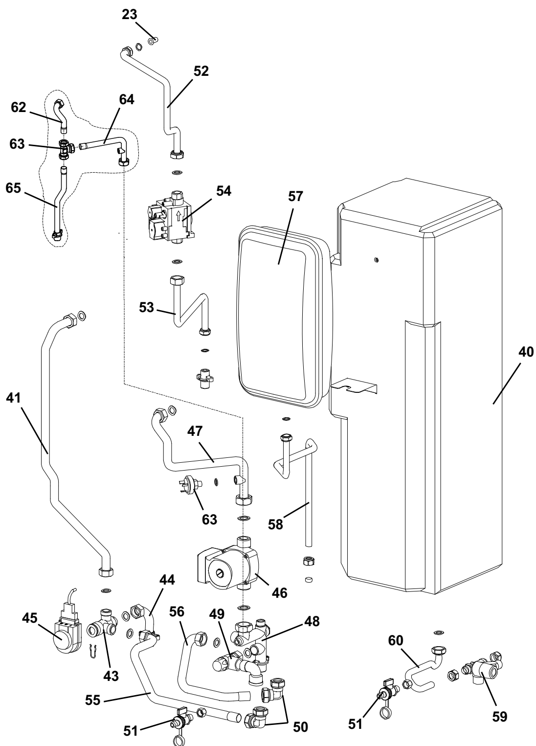
Abb. 37: Verrohrungsbauteile
