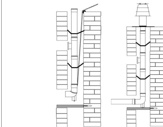
Abb. 12: Einführen in einen Schacht
