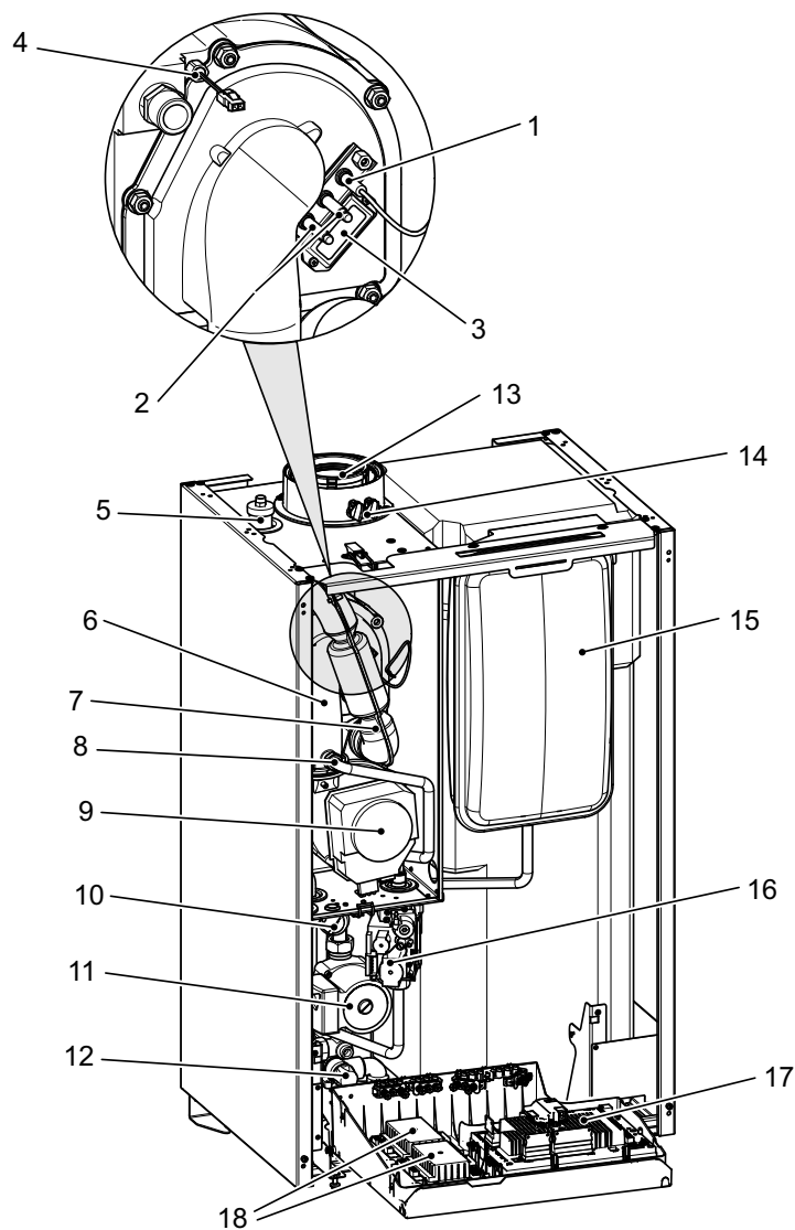
Abb. 33: Kesselansicht WGB-K (dargestellt ohne Vorderwand und Abdeckung der Regelung)
