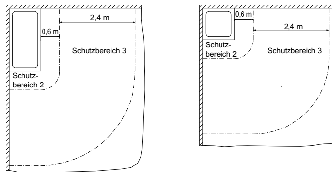
Abb. 4: Abstände in Bad- bzw. Duschräumen
