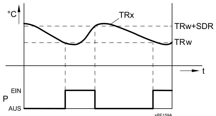
Abb. 20: Raumtemperaturbegrenzung
