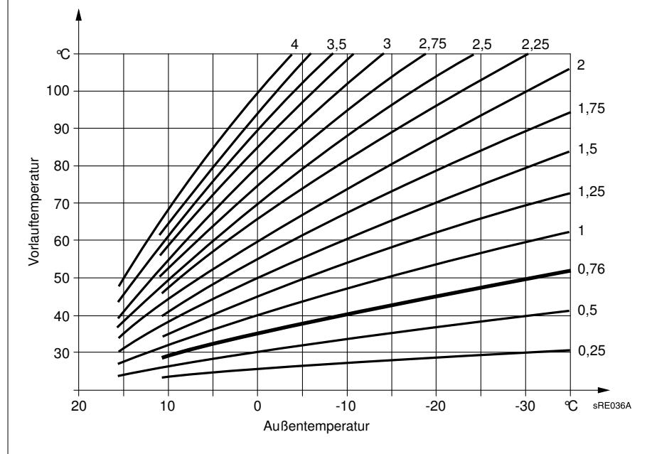
Abb. 18: Heizkennlinien-Diagramm
