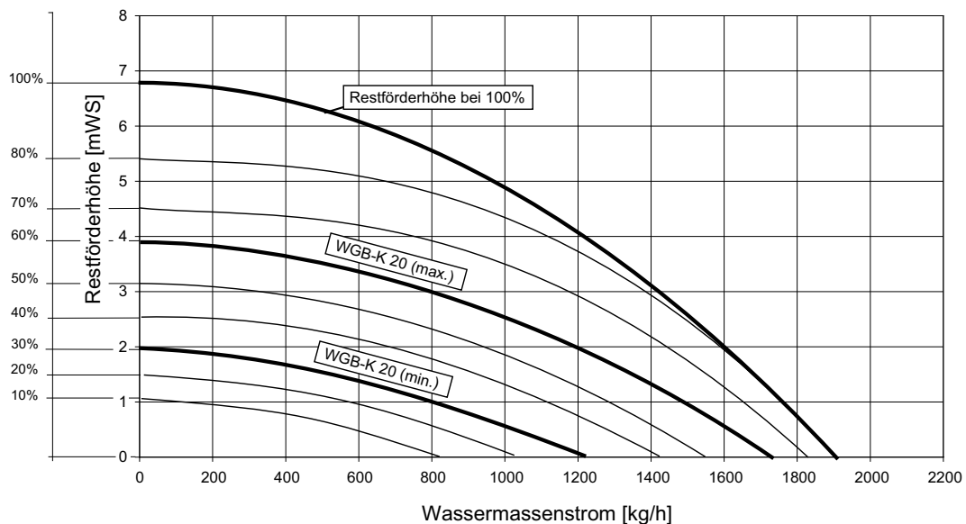
Abb. 25: Restförderhöhe WGB-K 20 E
