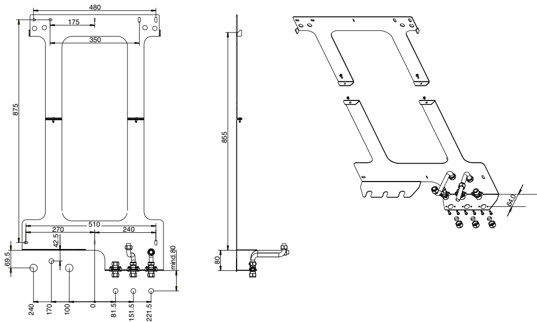
Abb. 2: SMR-KC Schnellmontagerahmen*) für WGB-K
