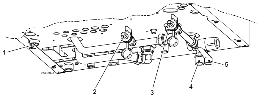
Abb. 9: Unterseite WGB-K
