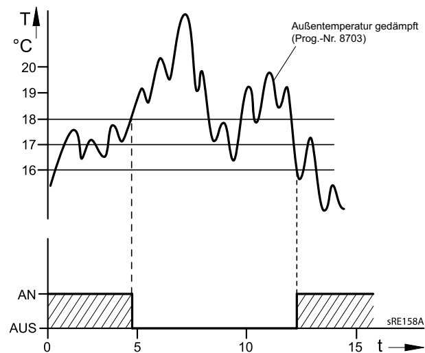
Abb. 19: Sommer-/Winterheizgrenze
