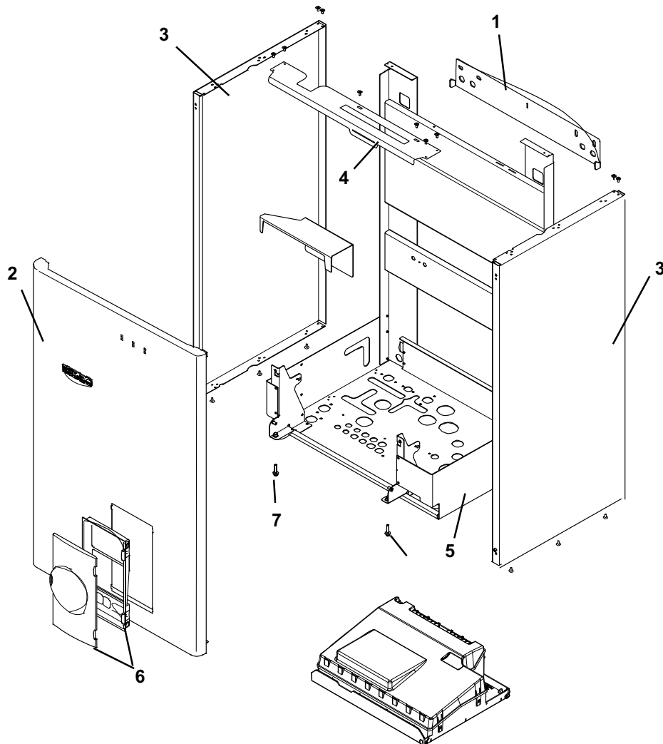
Abb. 35: Verkleidungsbauteile
