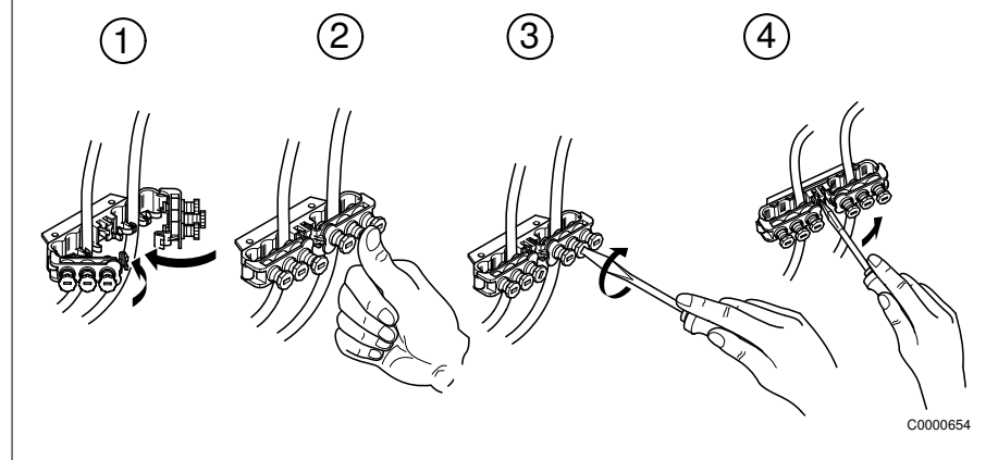
Abb. 15: Zugentlastung
