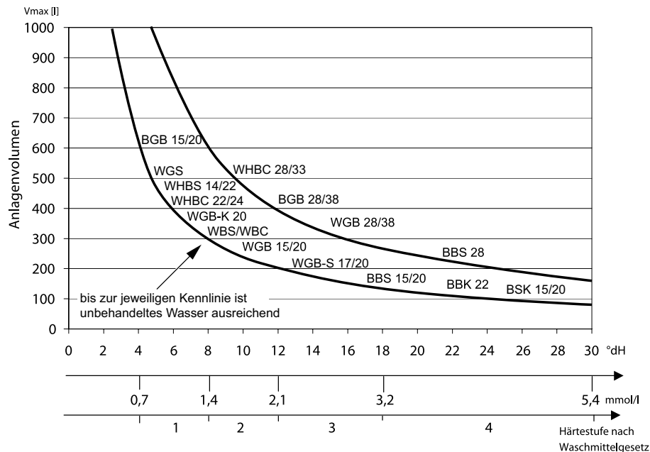
Abb. 3: Diagramm Wasserhärte
