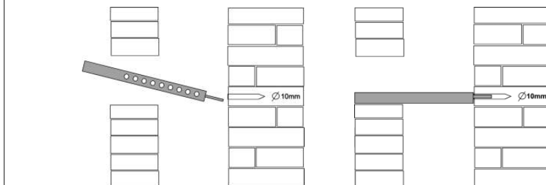
Abb. 11: Montage der Stützschiene
