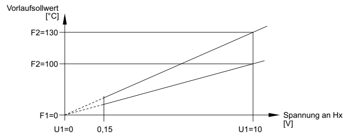
Abb. 30: Beispiel für Wärmeanforderung 10 V und Kälteanforderung 10 V
