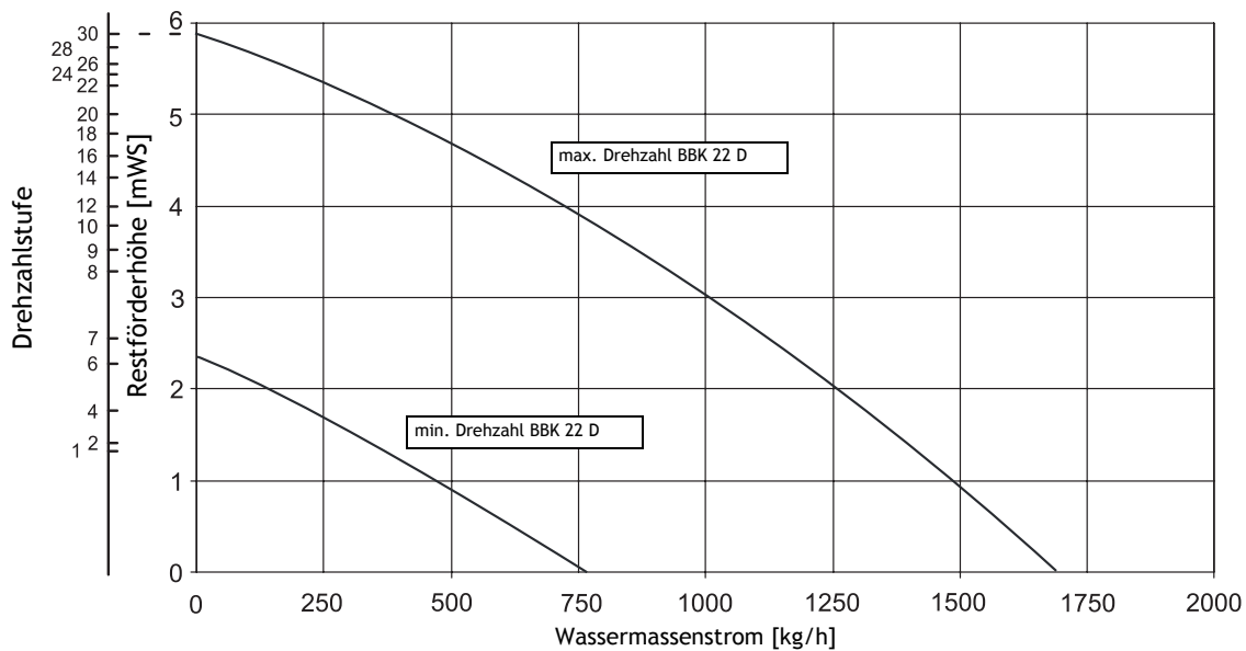
Abb. 16: Restförderhöhe
