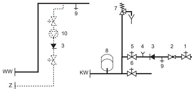
Abb. 4: Installationsbeispiel nach DIN 1988
