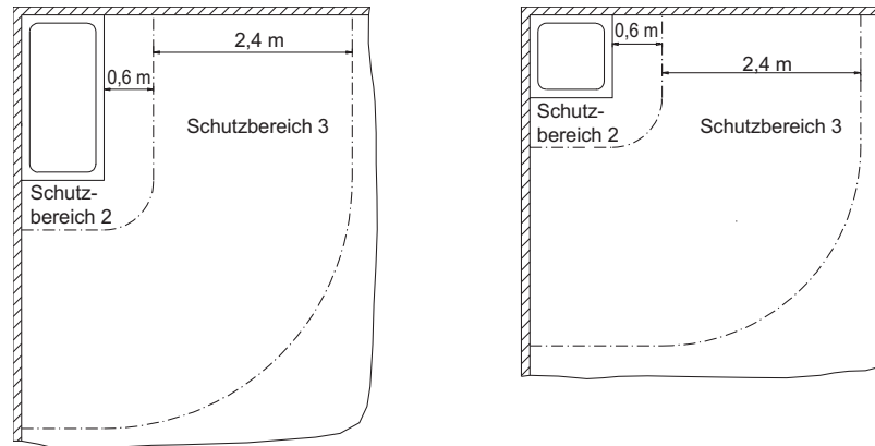
Abb. 3: Abstände BBK in Bad- bzw. Duschräumen
