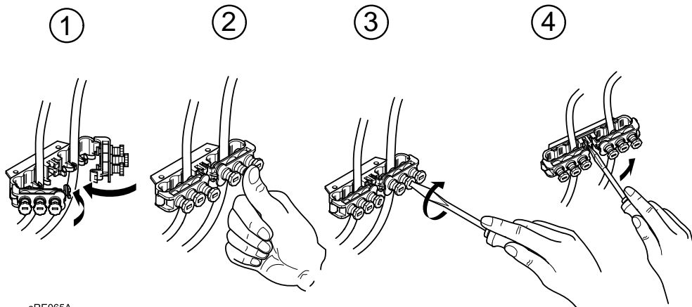
Abb. 10: Zulentlastung
