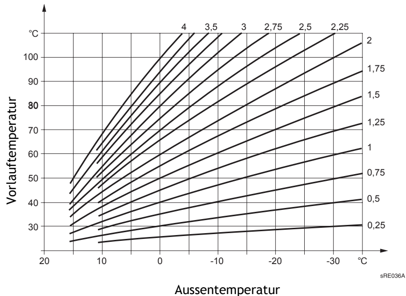
Abb. 14: Heizkennlinien-Diagramm
