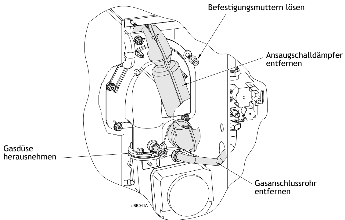
Abb. 20: Gasbrenner ausbauen
