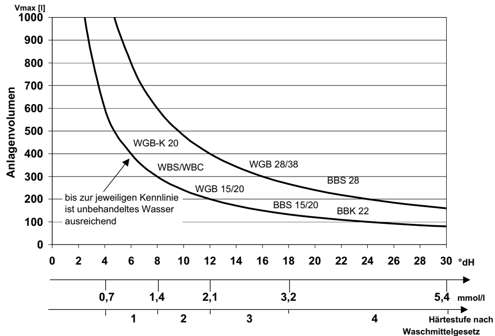
Abb. 2: Diagramm Wasserhärte
