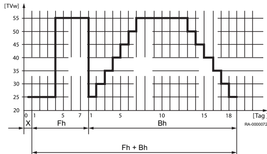
Abb.32 Temperaturprofil bei der Estrich-Austrocknungsfunktion
