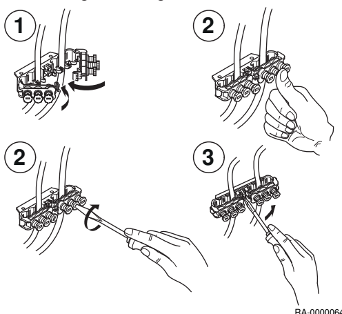
Abb. 19 Zugentlastungen
