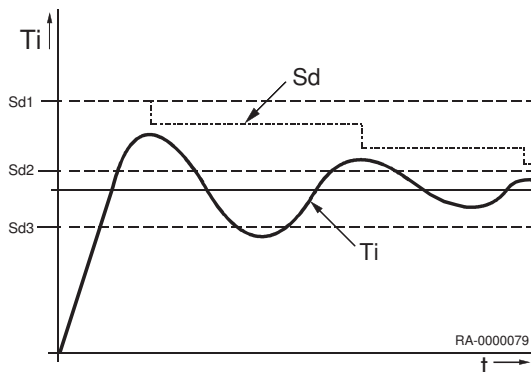
Abb.35 Schaltdifferenz
