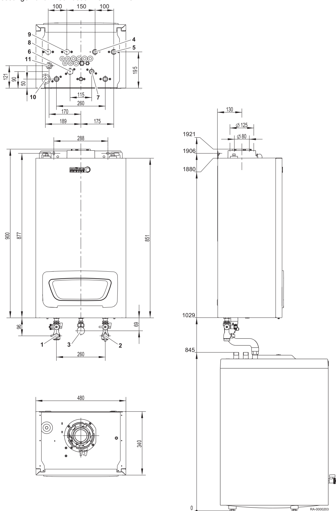
Abb.3 Abmessungen und Anschlüsse WGB-M EVO
