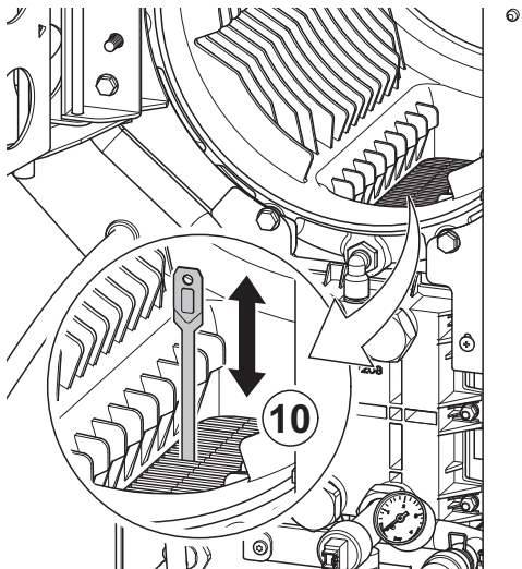
Abb.52 Reinigen des Wärmetauschers
