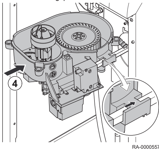
Abb.42 Demontage der Mischeinrichtung/des Lüfterrads
