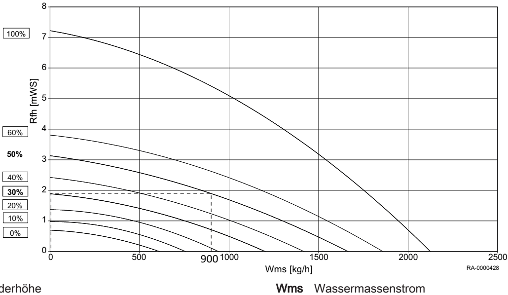
Abb.25 Beispiel für Restförderhöhe
