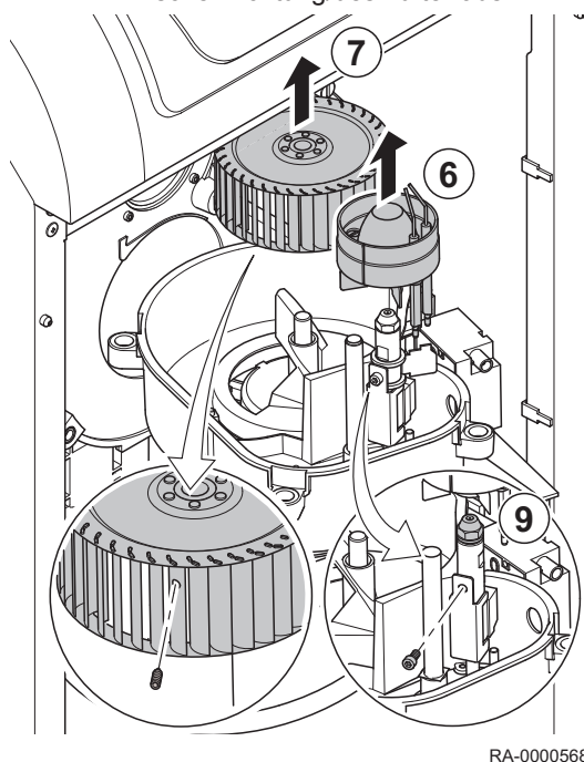
Abb.42 Demontage der Mischeinrichtung/des Lüfterrads
