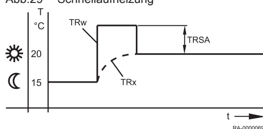
Abb.29 Schnellaufheizung
