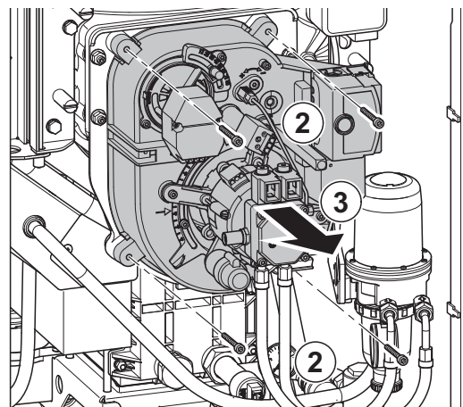
Abb.40 Entfernen des Brenneroberteils
