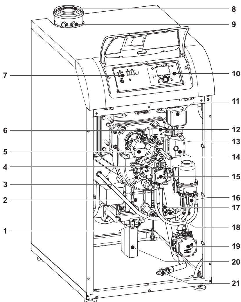
Abb.5 Kesselansicht BOB 20/25 B
