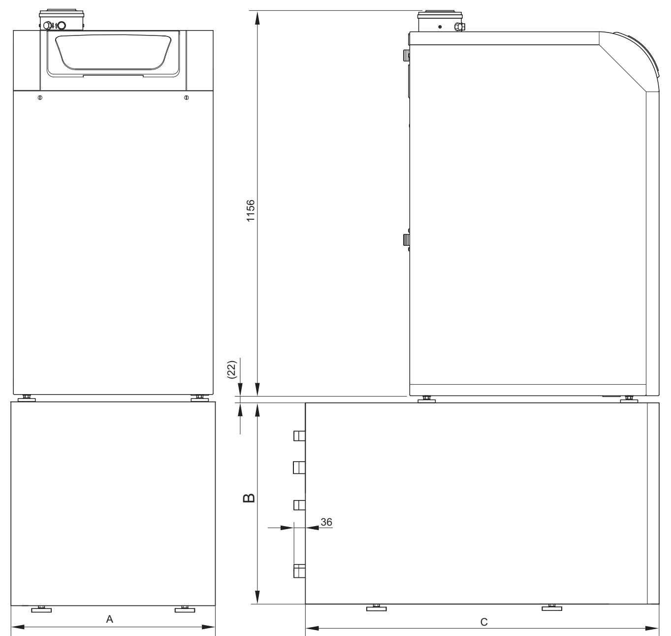
Abb.3 Abmessungen BOB mit Tiefspeicher EAS-T 150 - 200 C
