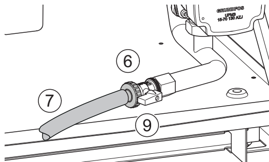
Abb.65 KFE-Hahn mit Schlauchtülle
