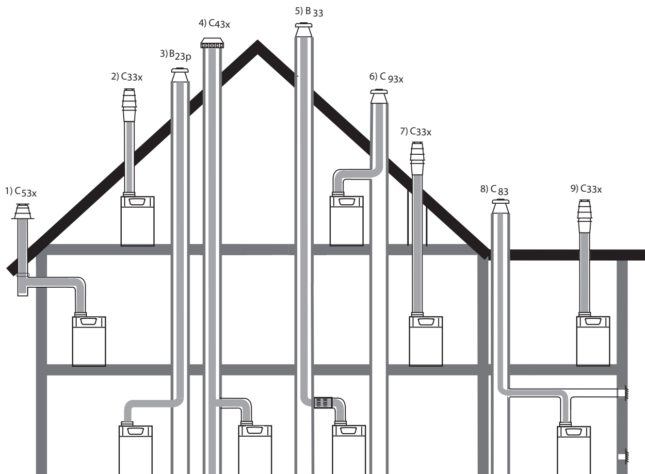
Abb.18 Anschlussmöglichkeiten mit KAS 80 (Zubehör)
