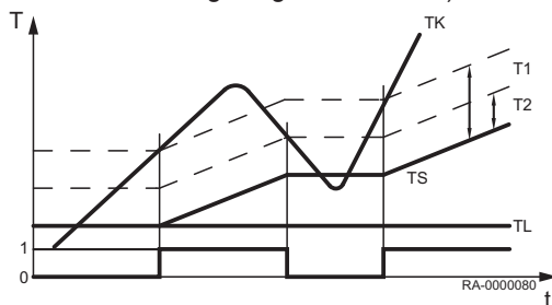
Abb.35 Laderegelung /schematisch)
