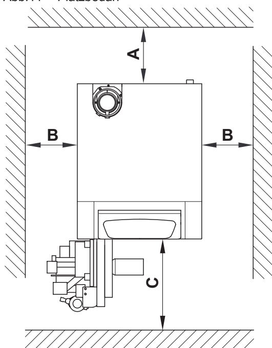
Abb.11 Platzbedarf
