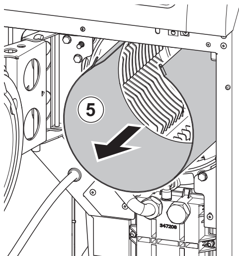
Abb.50 Entfernen des Feuerraumblechs
