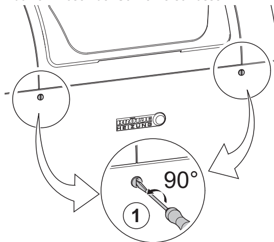
Abb. 15 Lösen der Schnellverschlüsse
