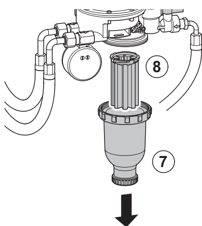
Abb.57 Wechseln des Filtereinsatzes
