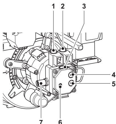
Abb.7 Bedienelemente und Anschlüsse
