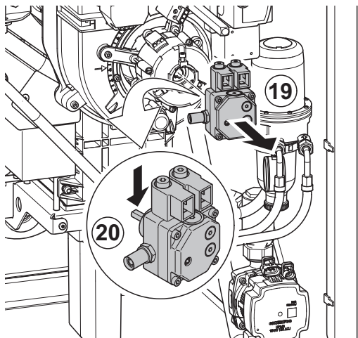
Abb.46 Ausbau der Ölpumpe
