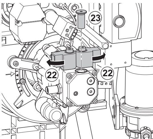
Abb.47 Ausbau des Ölfilters
