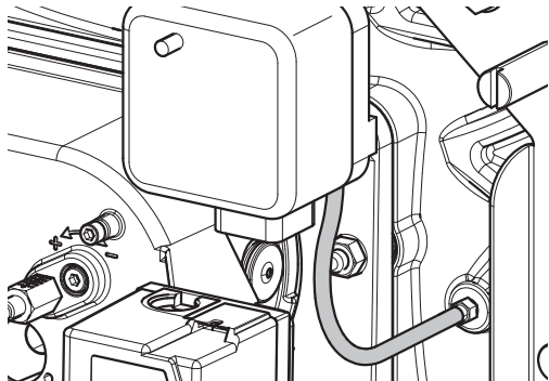
Abb.1 Schlauchverbindung Gasdruckwächter-Brennerraum
