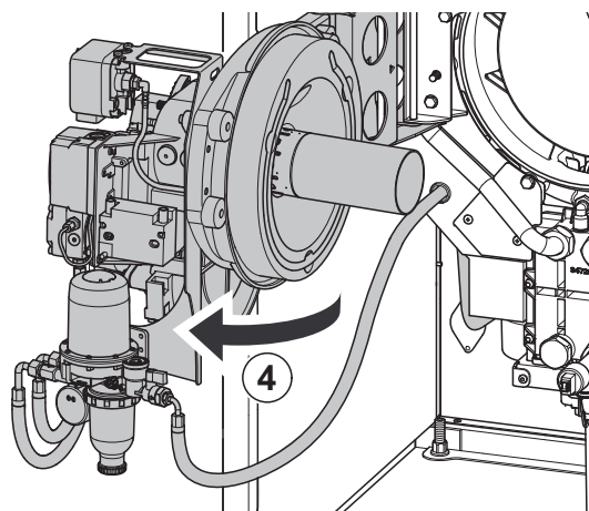
Abb.49 Herausschwenken der Brennergür
