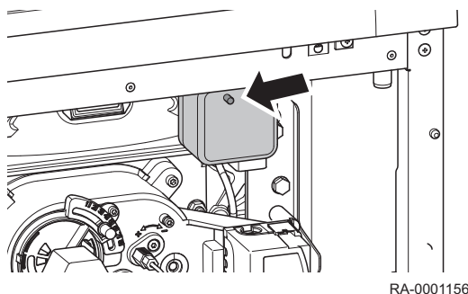
Abb.63 Entriegelungsknopf Luftdruckschalter
