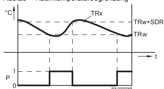
Abb.28 Raumtemperaturbegrenzung
