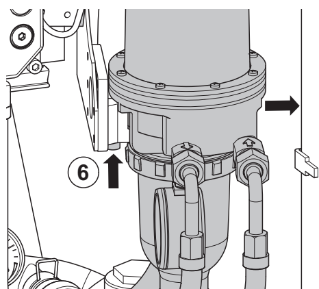
Abb.56 Ausbau des Ölfilter
