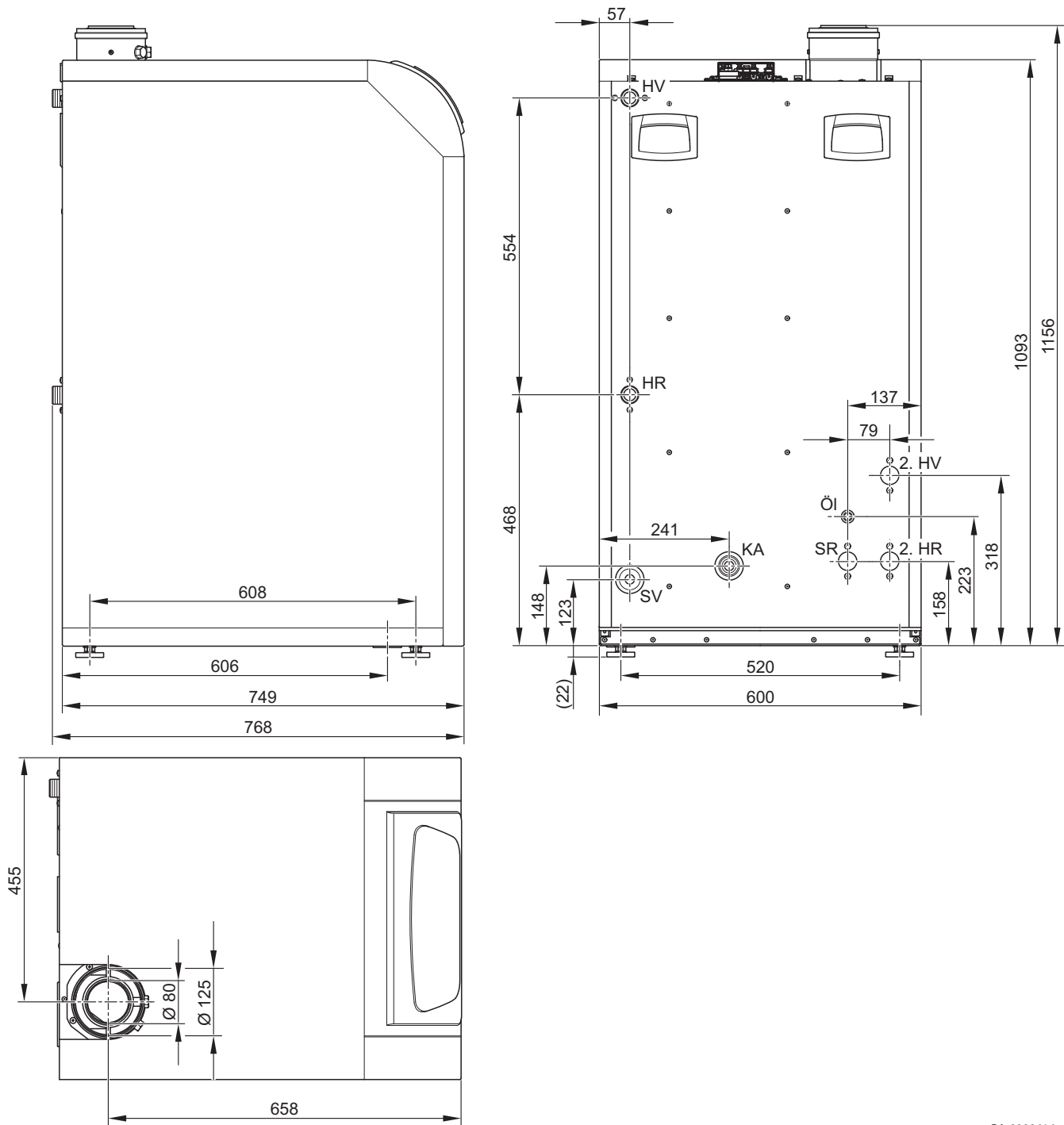
Abb.2 Abmessungen und Anschlüsse BOB
