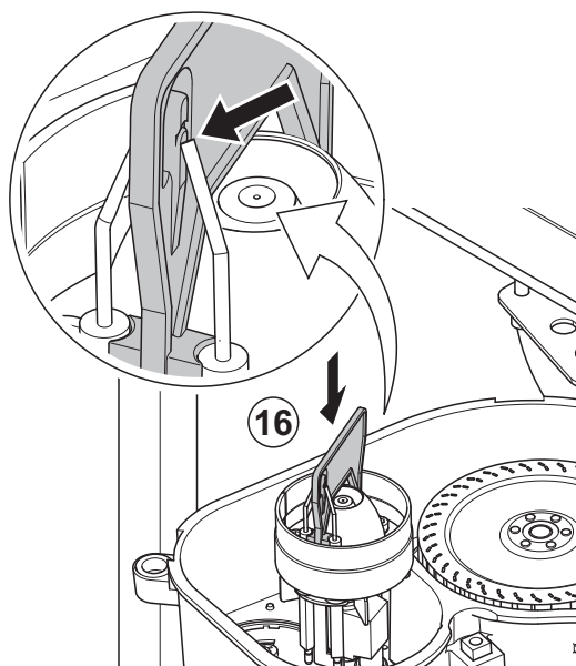
Abb.45 Prüfen des Elektrodenabstandes
