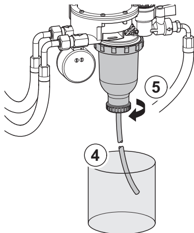
Abb.56 Ausbau des Ölfilter
