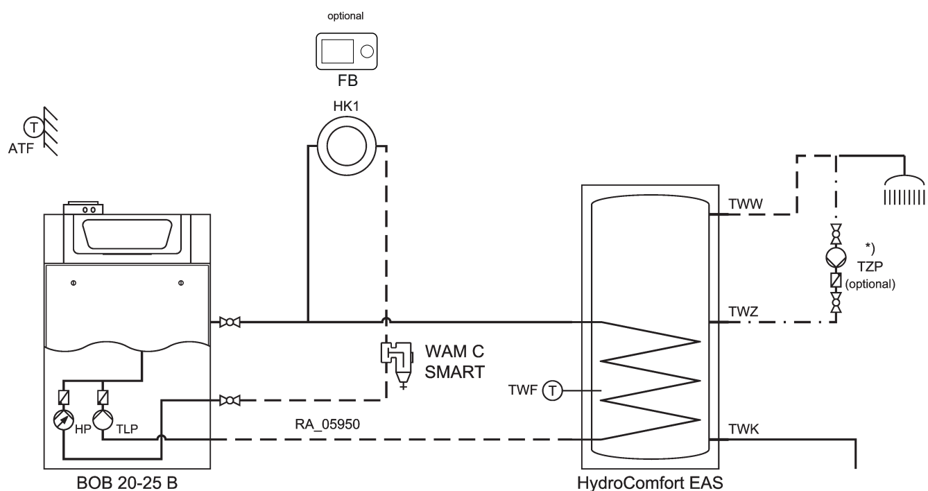
Abb.13 Hydraulikplan - BOB, ein Pumpenheizkreis mit Raumgerät, inkl. Speichertemperaturregelung
