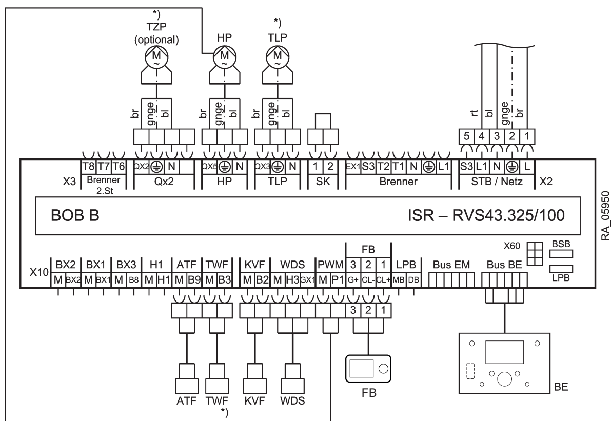
Abb.14 Anschlussplan - BOB, ein Pumpenheizkreis mit Raumgerät, inkl. Speichertemperaturregelung
