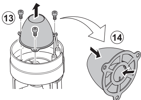
Abb.43 Entfernen und Reinigung der Luftdüse
