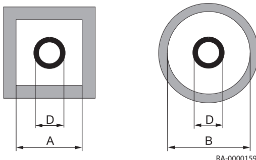
Abb.19 Mindestmaße des Schachtes
