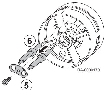
Abb.58 Entfernen der Zündelektroden
