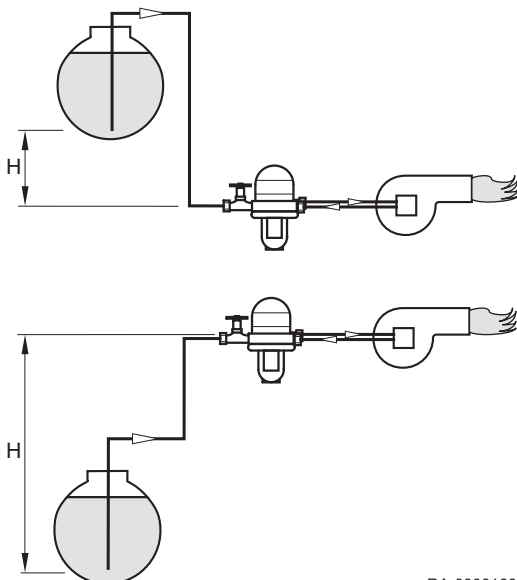
Abb.17 1-Strang-System mit Ölfiter
