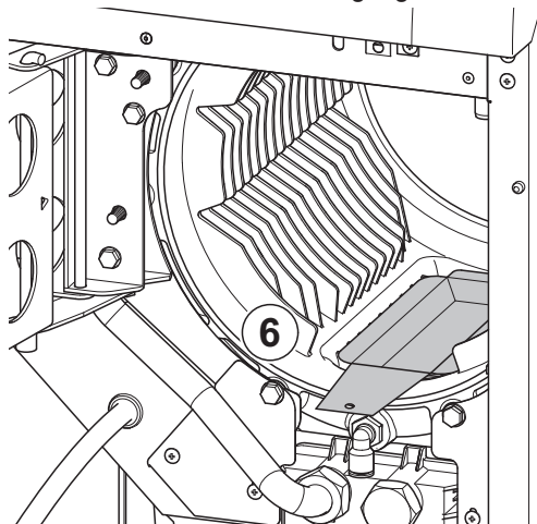
Abb.51 Einsetzen der Reinigungsschale
