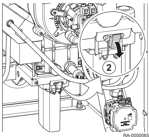
Abb.39 Entfernen des Siphons
