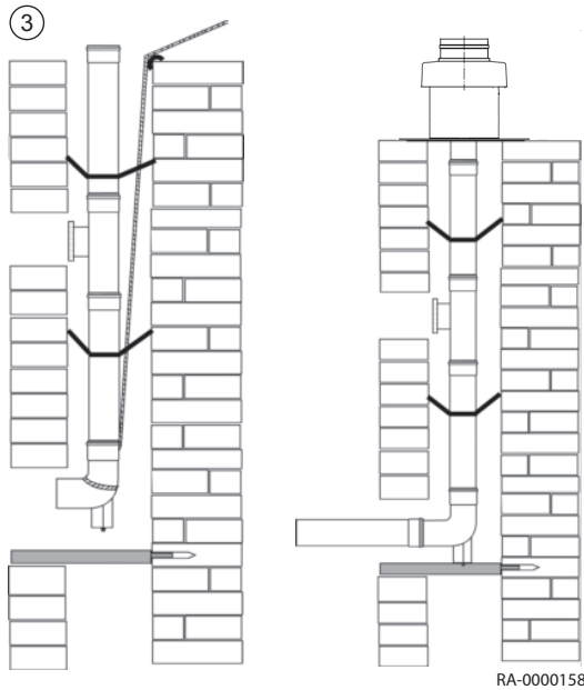
Abb.21 Einführen in den Schacht
