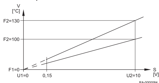
Abb.38 Beispiel für Wärmeanforderung 10 V
