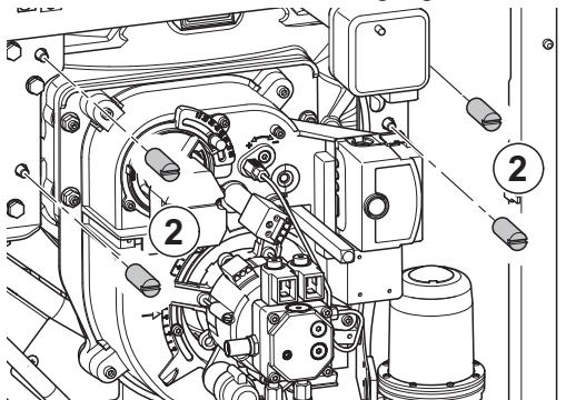
Abb.48 Entfernen der Befestigungsmuttern
