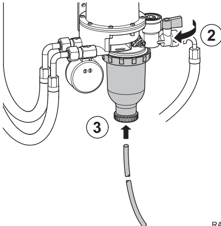
Abb.54 Anbringen des Ablassschlauchs
