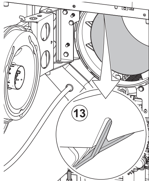
Abb.53 Einsetzen des Feuerraumblechs
