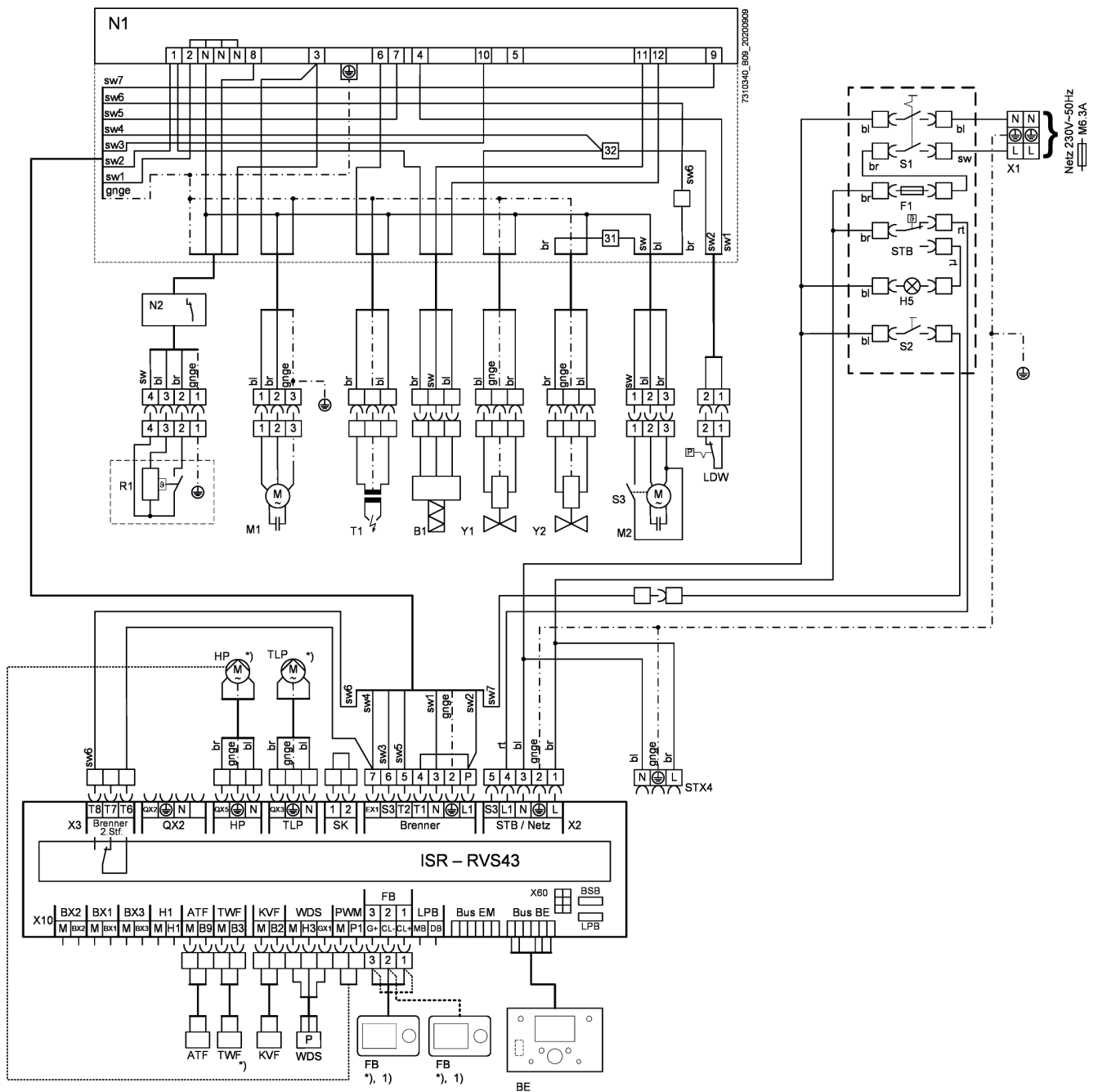
Abb.4 Schaltplan
