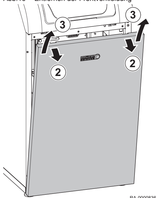
Abb.16 Entfernen der Frontverkleidung
