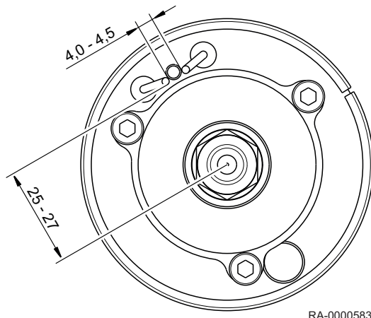
Abb.59 Einstellmaße
