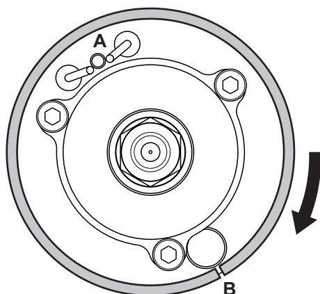
Abb.44 Position des Rezirkulationsrings
