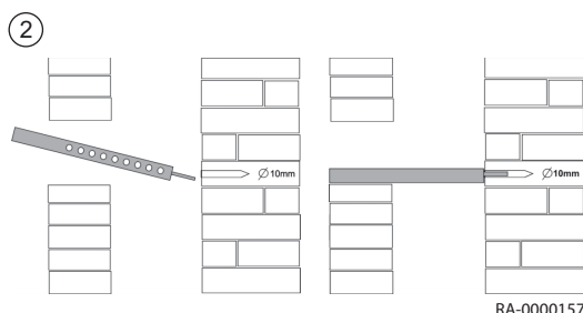
Abb.20 Montage der Stützschiene
