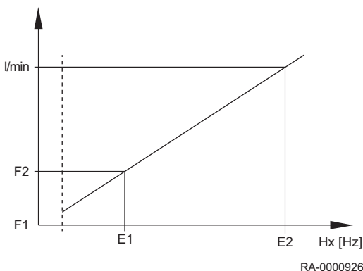
Abb.29 Beispiel für zwei unterschiedliche Fühlerkennlinien
