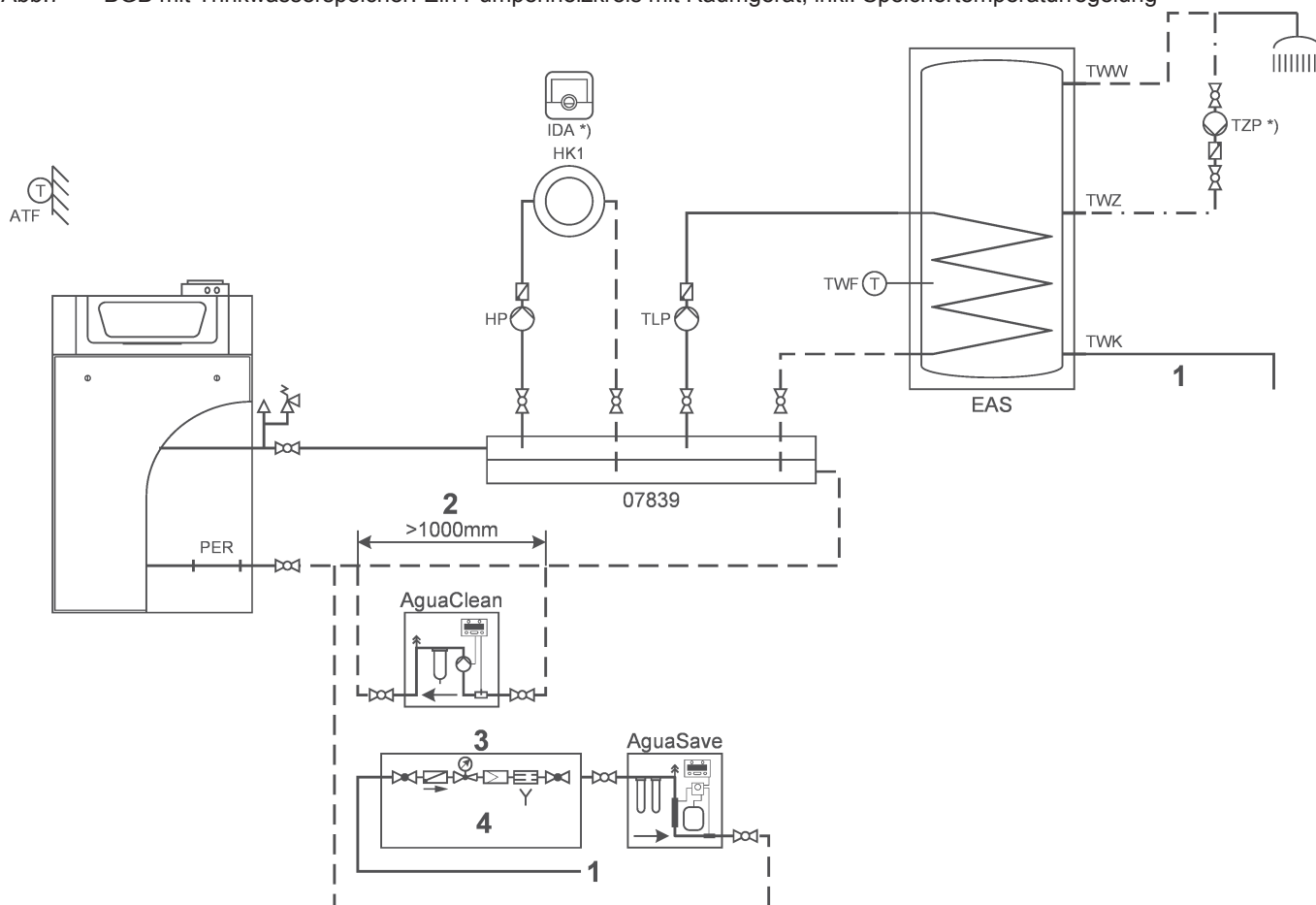
Abb.7 BGB mit Trinkwasserspeicher: Ein Pumpenheizkreis mit Raumgerät, inkl. Speichertemperaturregelung
