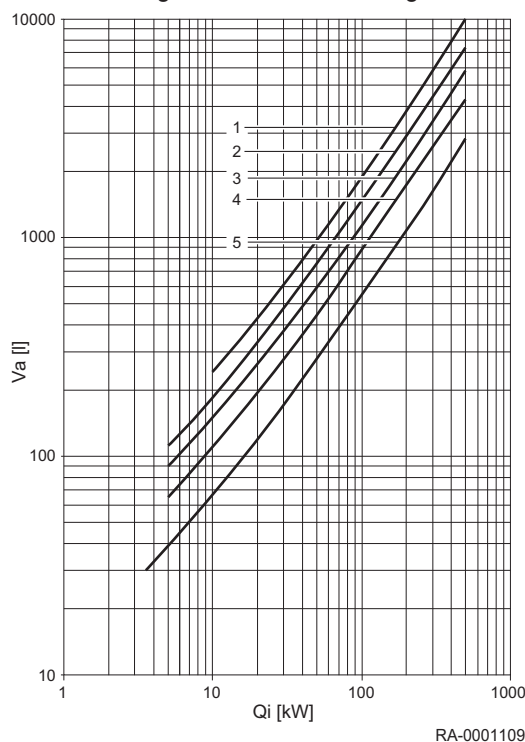
Abb.6 Anlagenvolumenbestimmung
