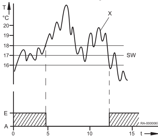
Abb.17 Sommer-/Winterheizgrenze
