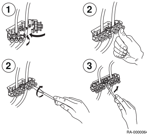
Abb.14 Zugentlastungen
