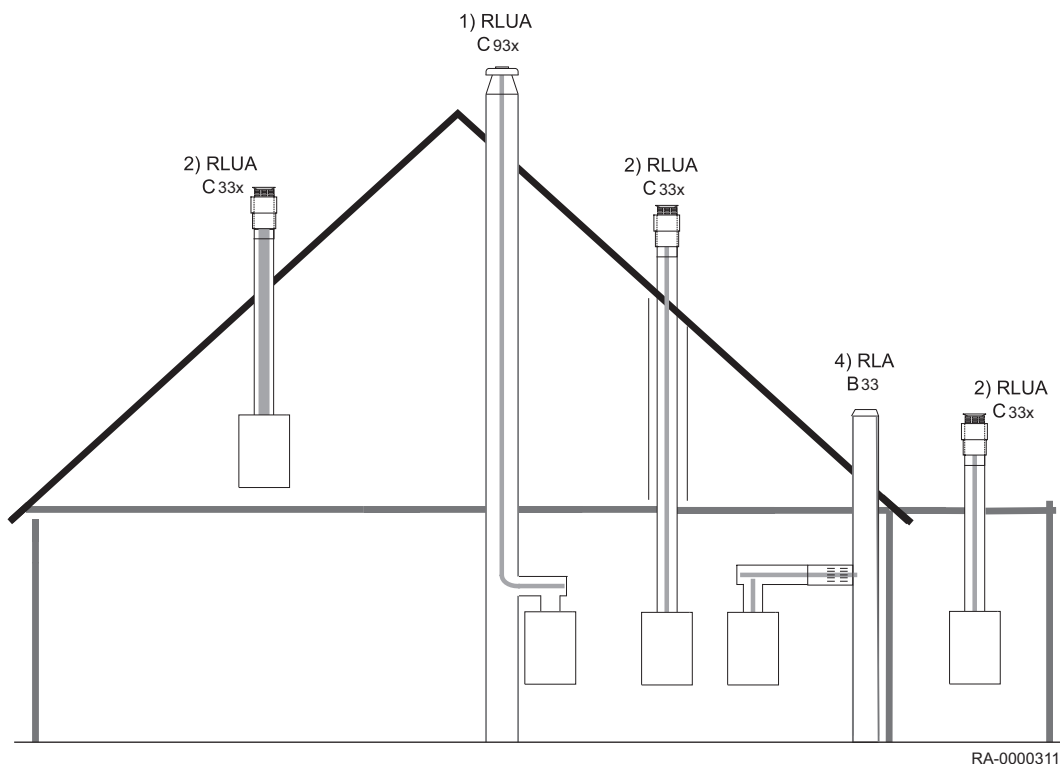
Abb.10 Anschlussmöglichkeiten mit KAS (Zubehör)
