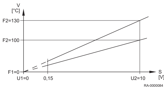
Abb.30 Beispiel für Wärmeanforderung 10 V
