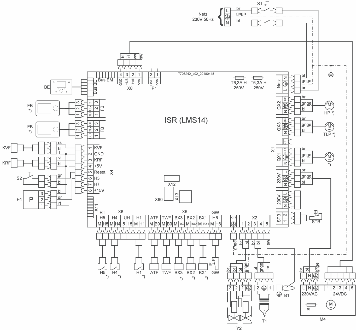
Abb.3 Schaltplan BGB 70 - 110
