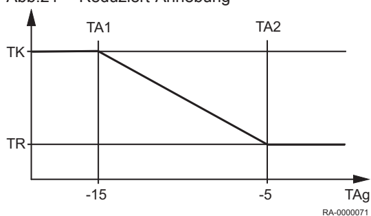
Abb.21 Reduziert-Anhebung
