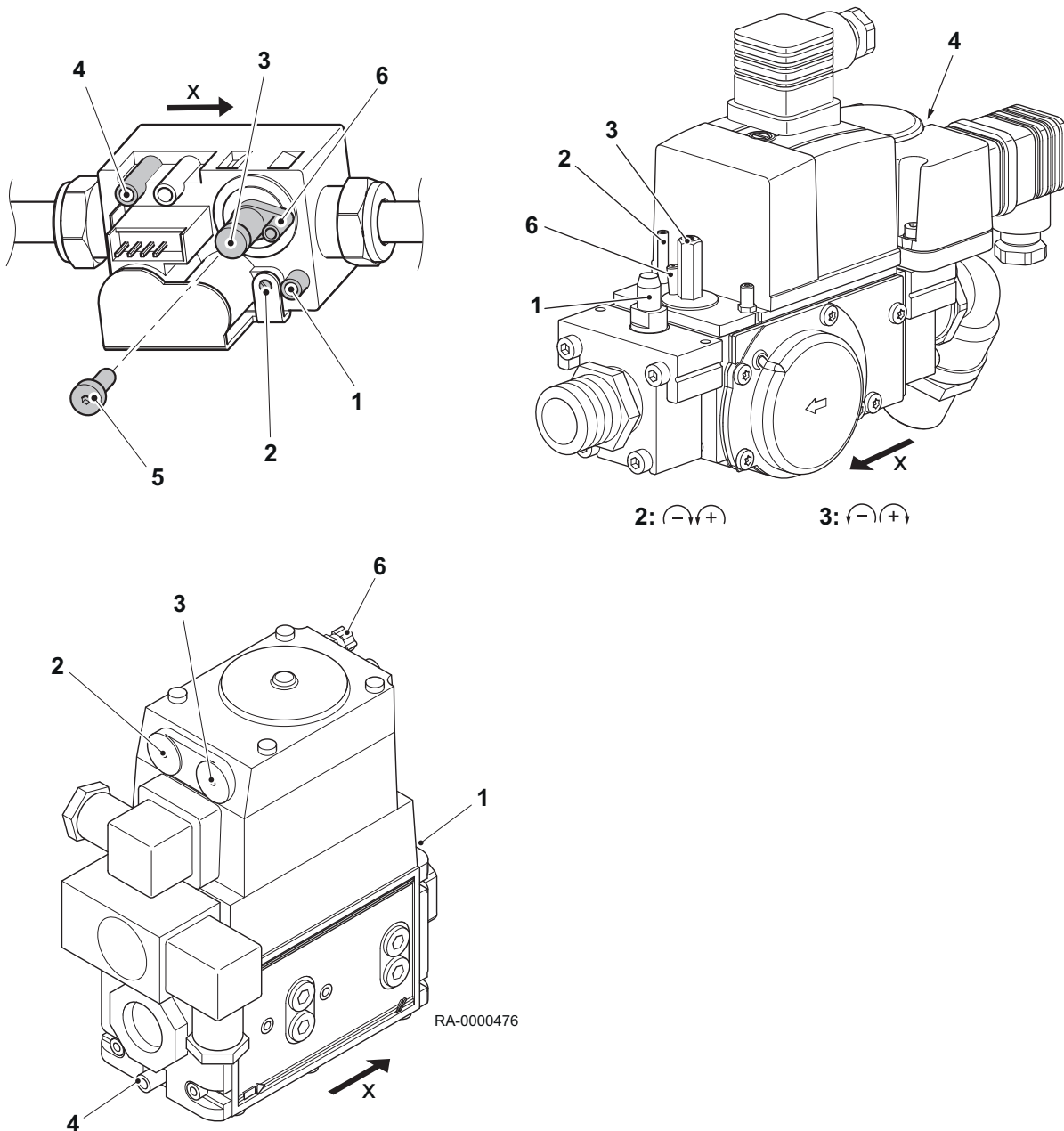
Abb.15 Gasventil
