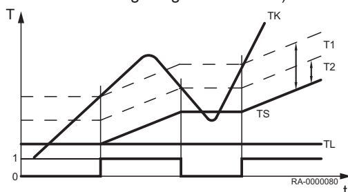
Abb.26 Laderegelung /schematisch)
