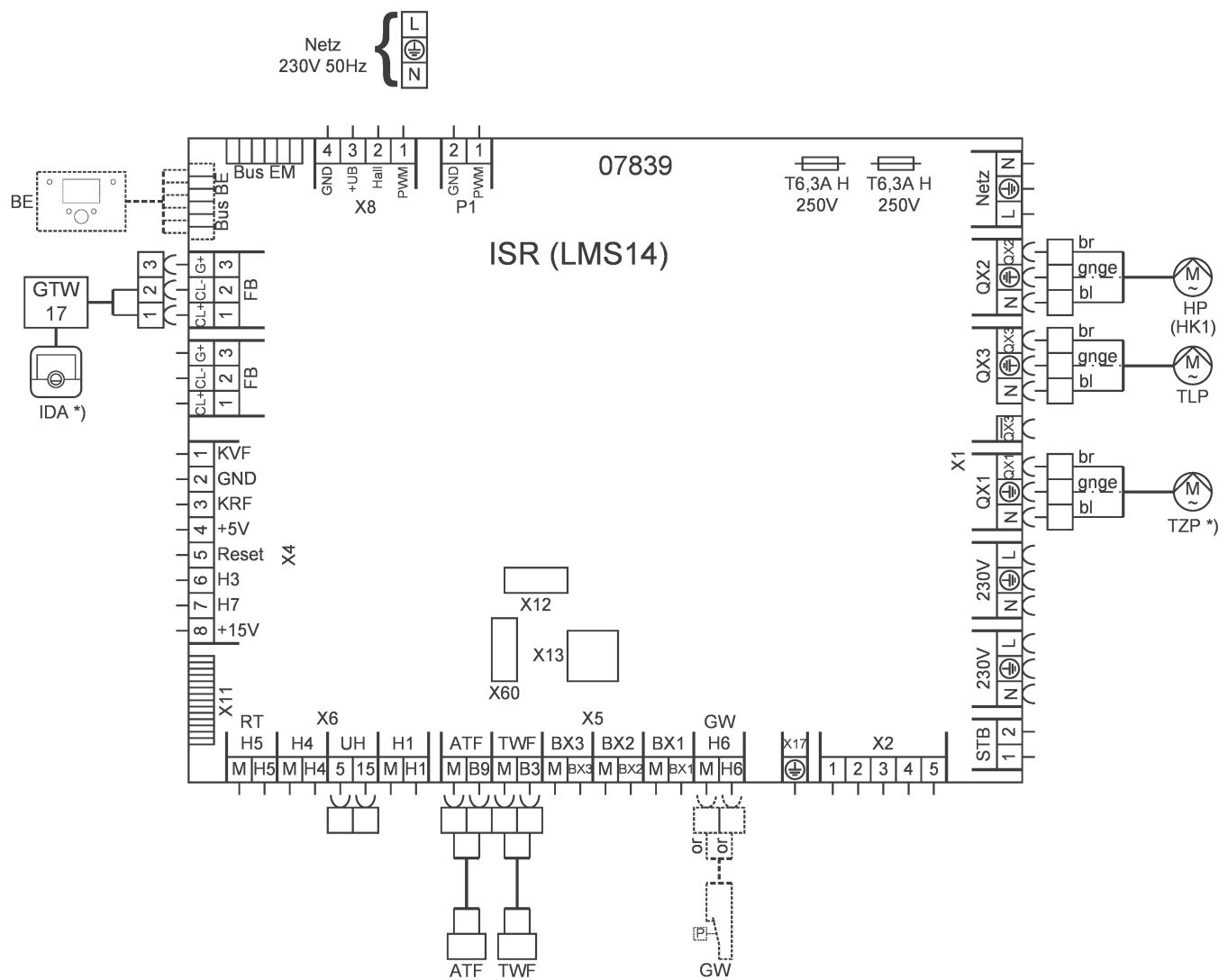
Abb.8 Anschlussplan
