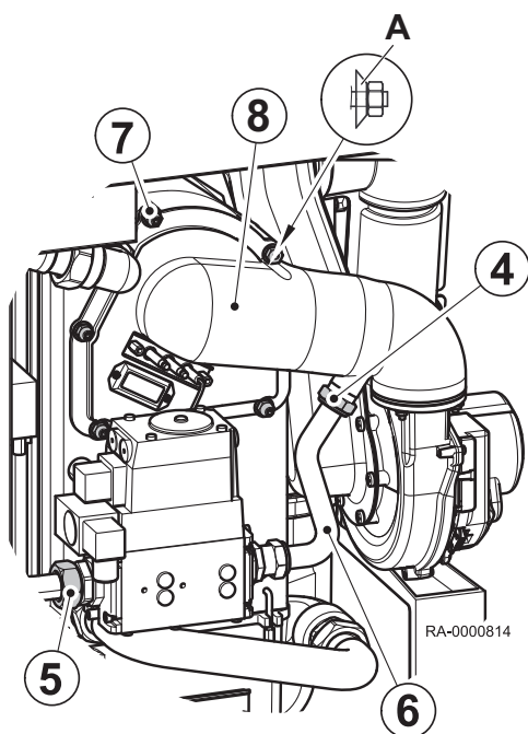
Abb.32 Gasbrenner ausbauen
