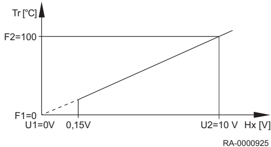
Abb.28 Spannungswert/Funktionswert
