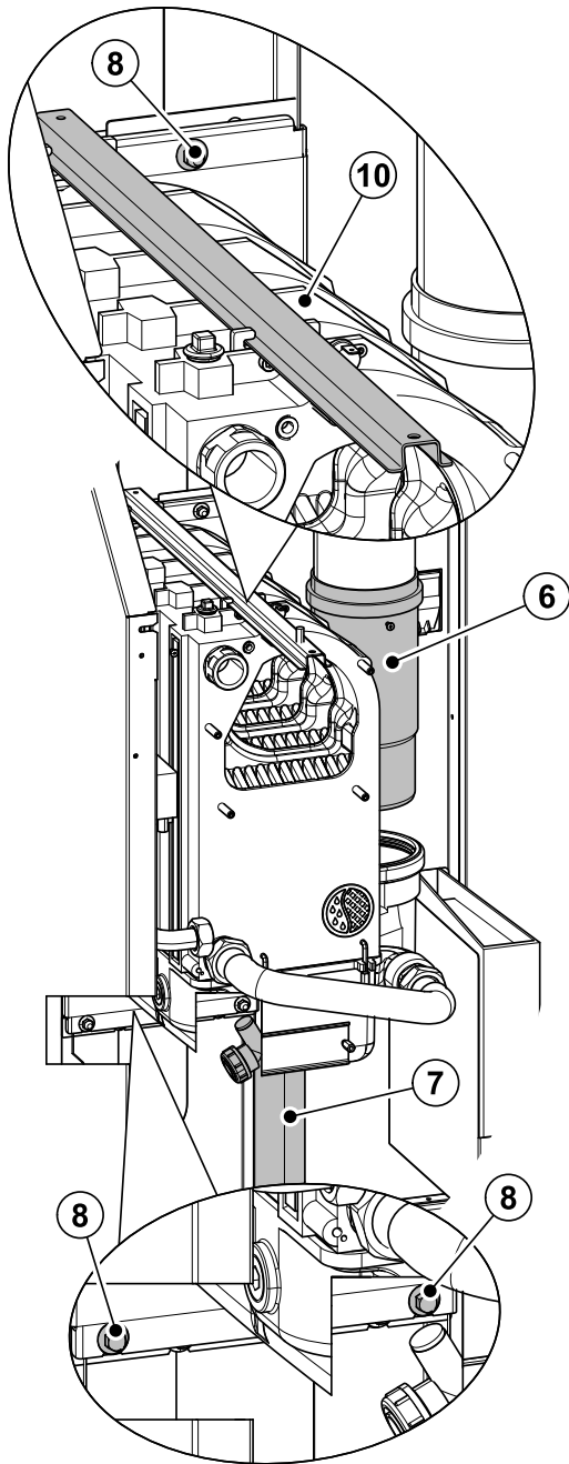
Abb.33 Wärmetauscher ausbauen
