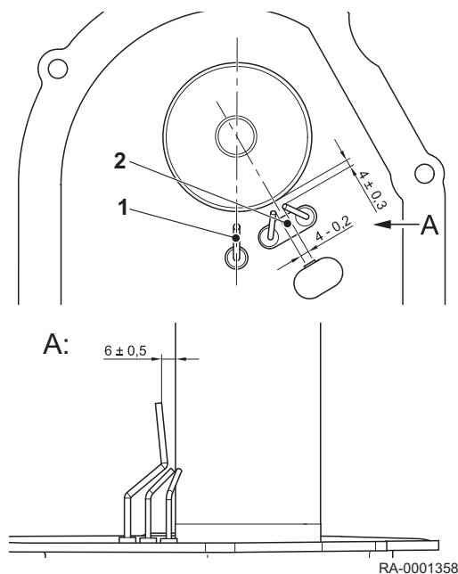
Abb.31 Elektroden
