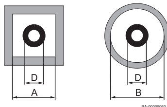
Abb.13 Mindestmaße des Schachtes
