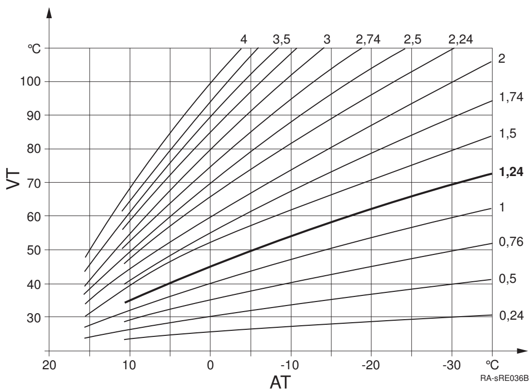
Abb.16 Heizkennlinien-Diagramm
