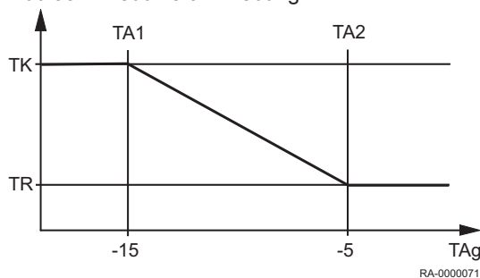
Abb.30 Reduziert-Anhebung
