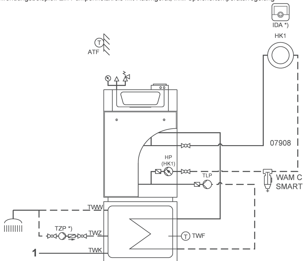
Abb.10 Anwendungsbeispiel: Ein Pumpenheizkreis mit Raumgerät, inkl. Speichertemperaturregelung
