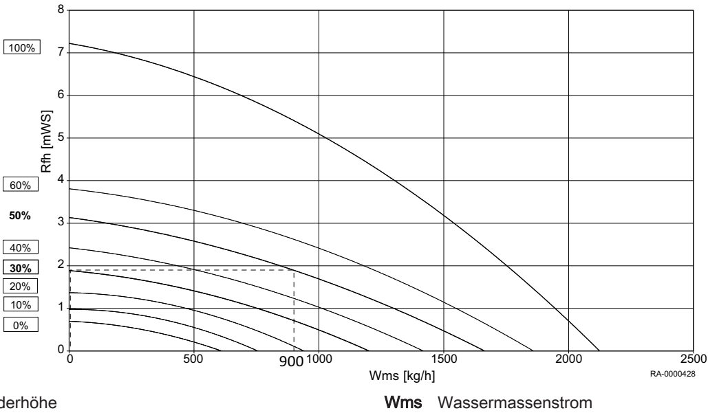
Abb.24 Beispiel für Restförderhöhe
