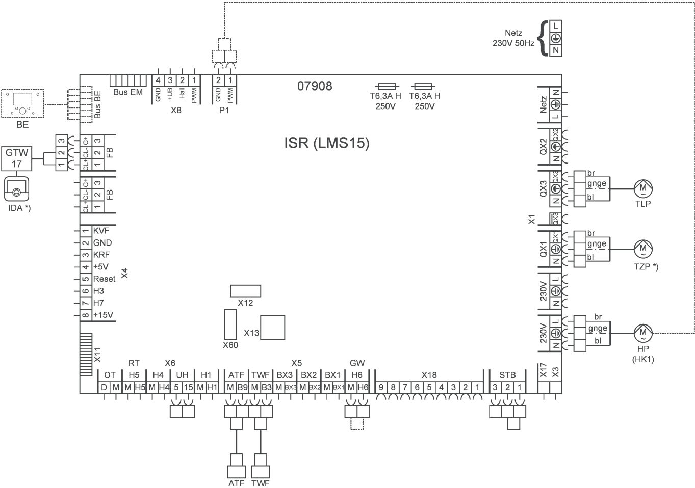
Abb.11 Anschlussplan
