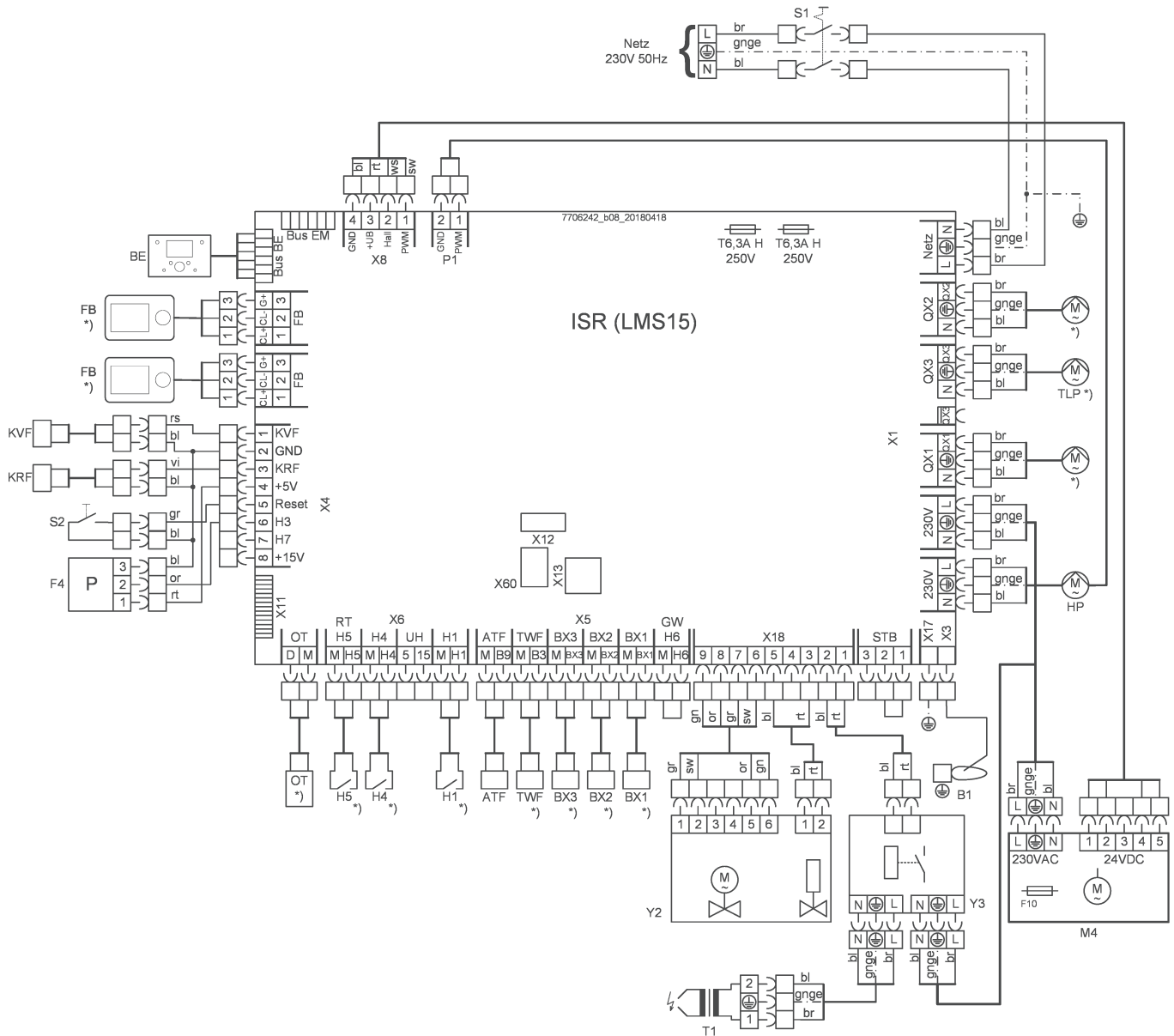
Abb.6 Schaltplan BGB EVO 38
