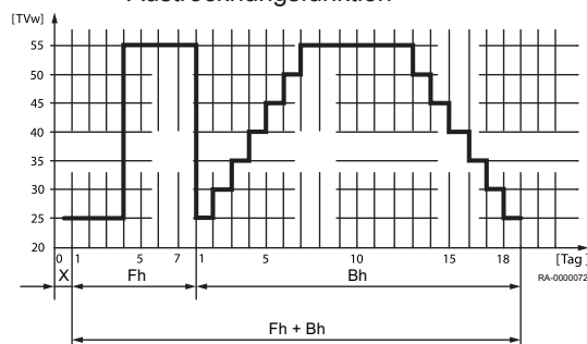
Abb.31 Temperaturprofil bei der Estrich-Austrocknungsfunktion
