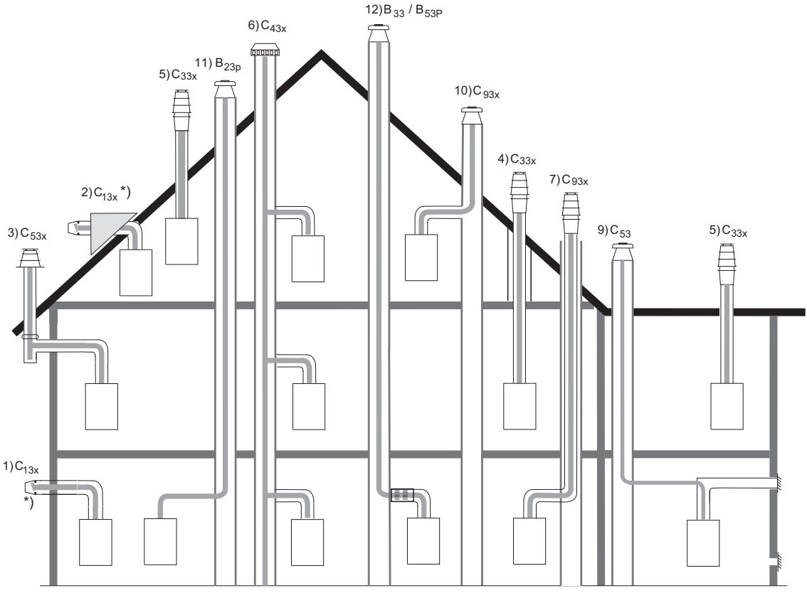
Abb.13 Anschlussmöglichkeiten mit KAS (Zubehör)
