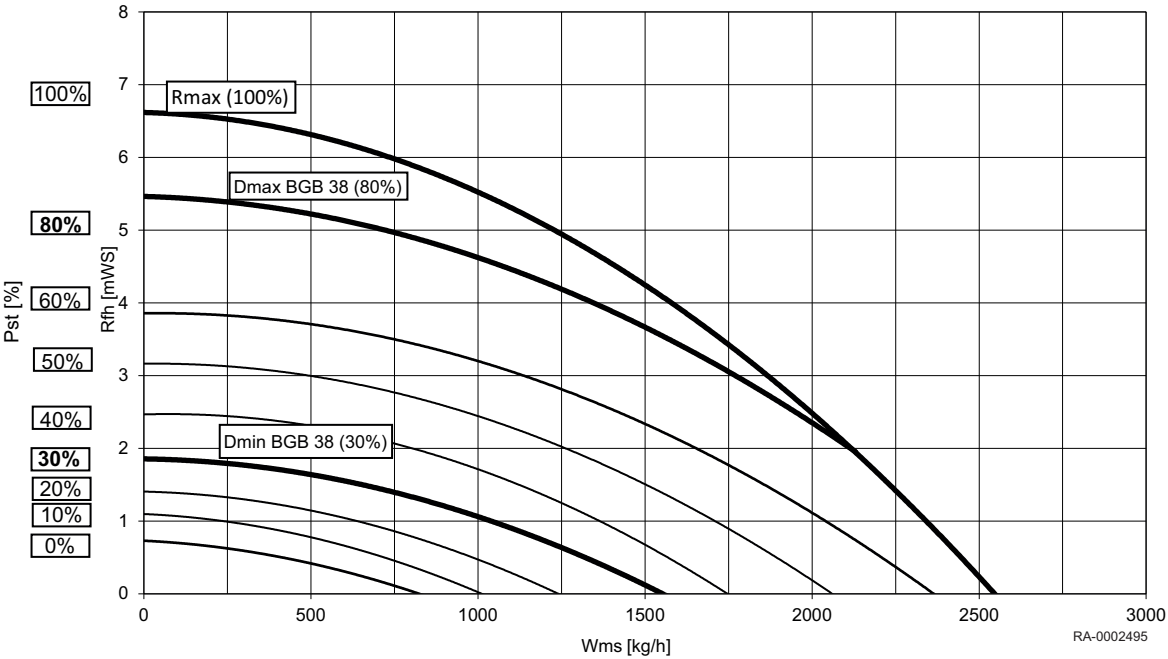
Abb.3 Restförderhöhe BGB EVO 38
