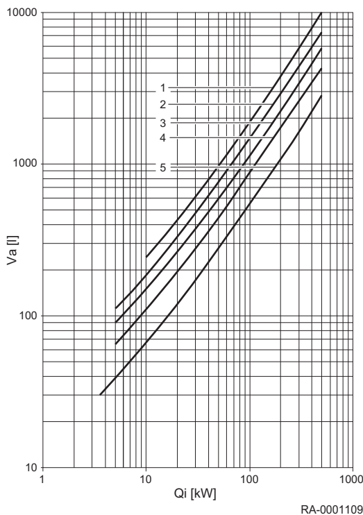
Abb.9 Anlagenvolumenbestimmung
