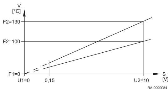
Abb.39 Beispiel für Wärmeanforderung 10 V
