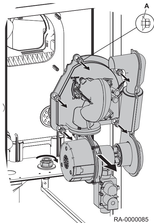
Abb.42 Gasbrenner ausbauen
