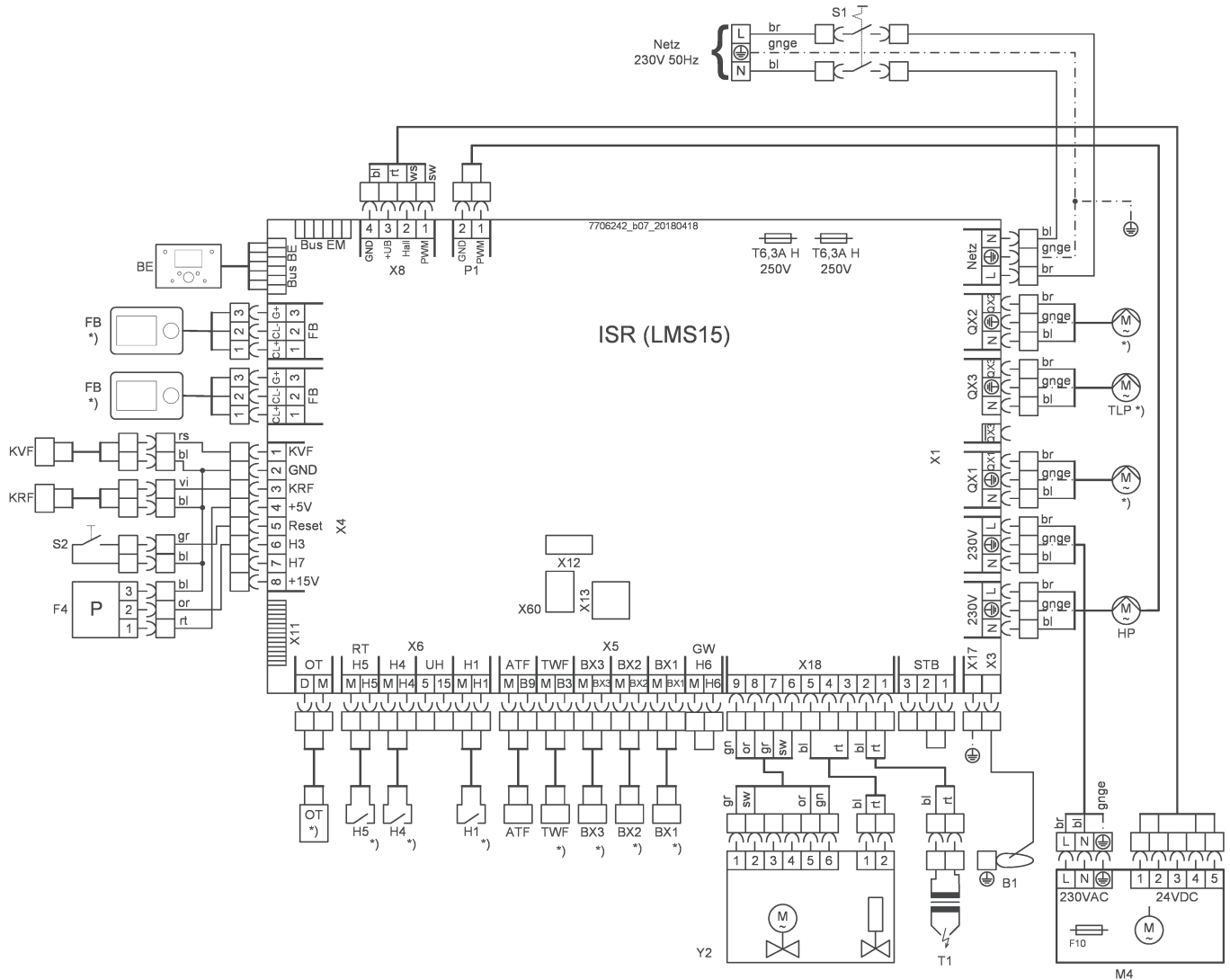
Abb.5 Schaltplan BGB EVO 15 - 28
