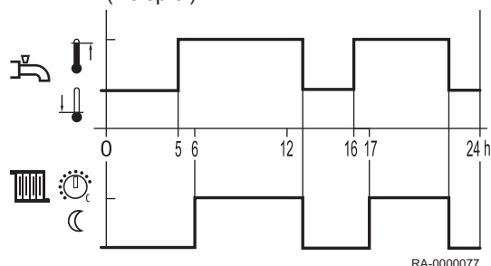
Abb.32 Freigabe in Abhängigkeit von den Zeitprogrammen der Heizkreise (Beispiel)
