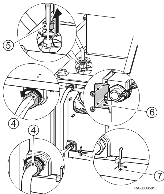
Abb.43 Wärmetauscher ausbauen
