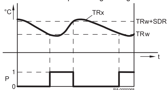
Abb.27 Raumtemperaturbegrenzung
