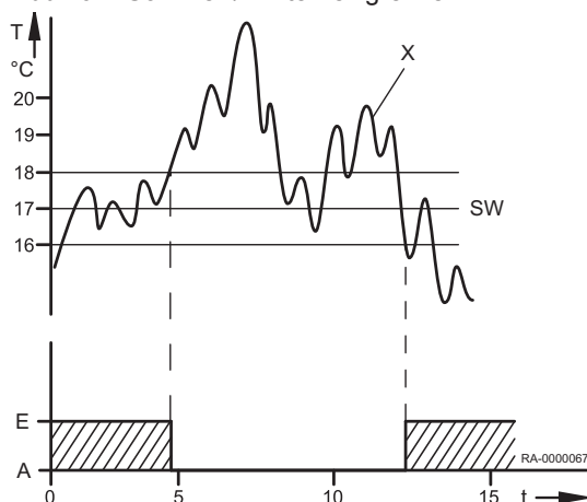
Abb.26 Sommer-/Winterheizgrenze
