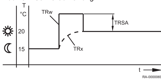
Abb.28 Schnellaufheizung
