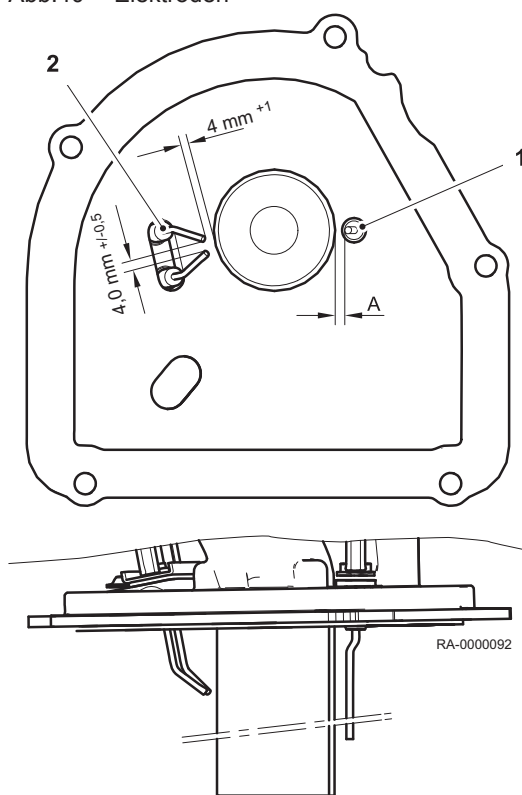
Abb.40 Elektroden
