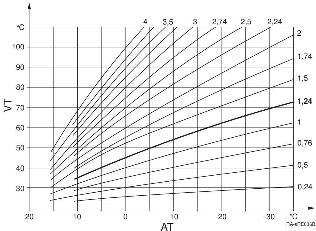
Abb.25 Heizkennlinien-Diagramm
