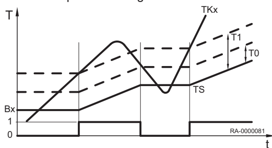
Abb.36 Speicherladung
