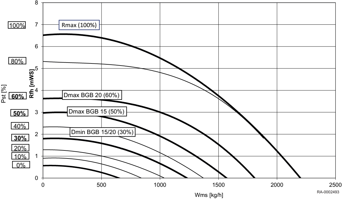
Abb.1 Restförderhöhe BGB EVO 15 - 20
