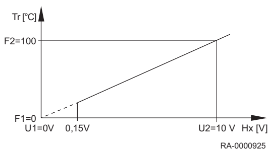
Abb.37 Spannungswert/Funktionswert
