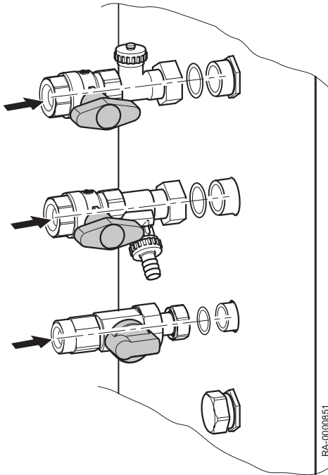
Abb.12 Einbau Absperrventile
