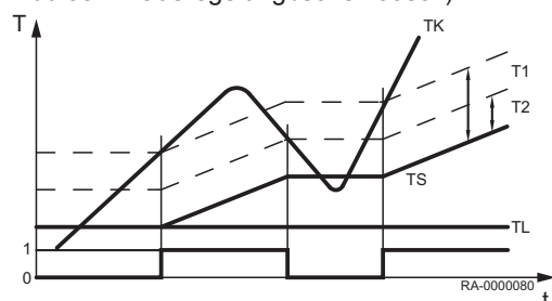
Abb.35 Laderegelung /schematisch)
