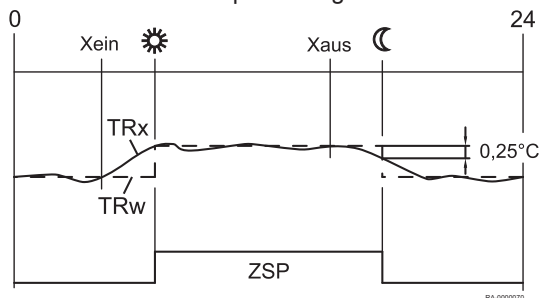
Abb.29 Einschalt- und Ausschaltoptimierung
