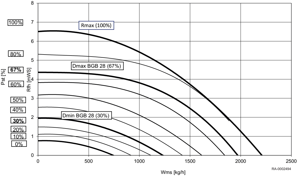
Abb.2 Restförderhöhe BGB EVO 28
