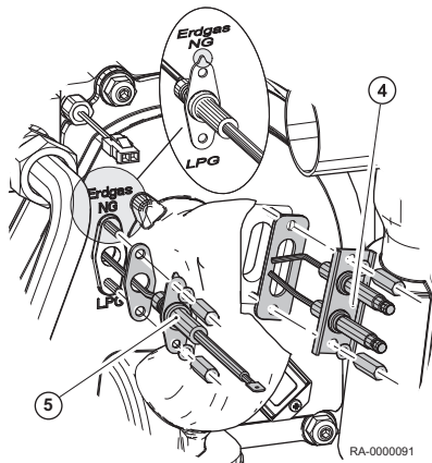
Abb.41 Zünd- und Ionisationselektrode ausbauen
