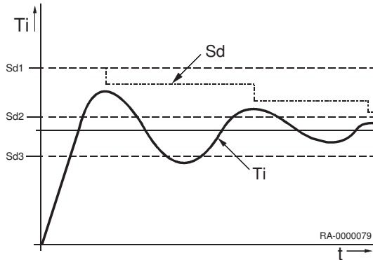
Abb.41 Schaltdifferenz
