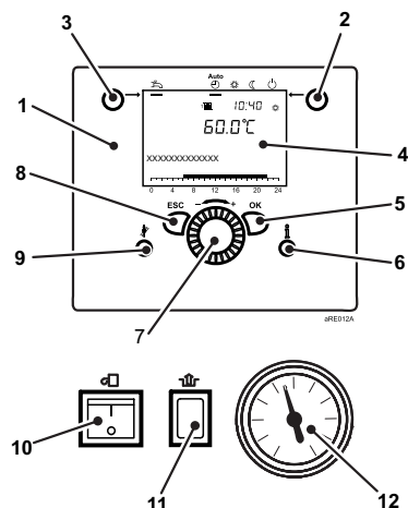
Abb.6 Bedienelemente
