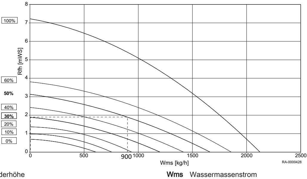
Abb.31 Beispiel für Restförderhöhe
