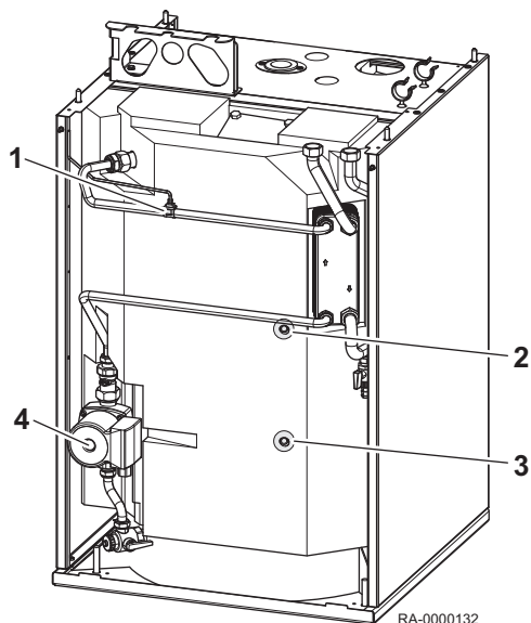
Abb.27 Schichtenspeicher SSP
