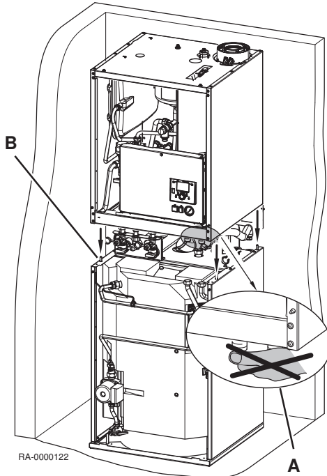
Abb.16 Montage Kesselteil
