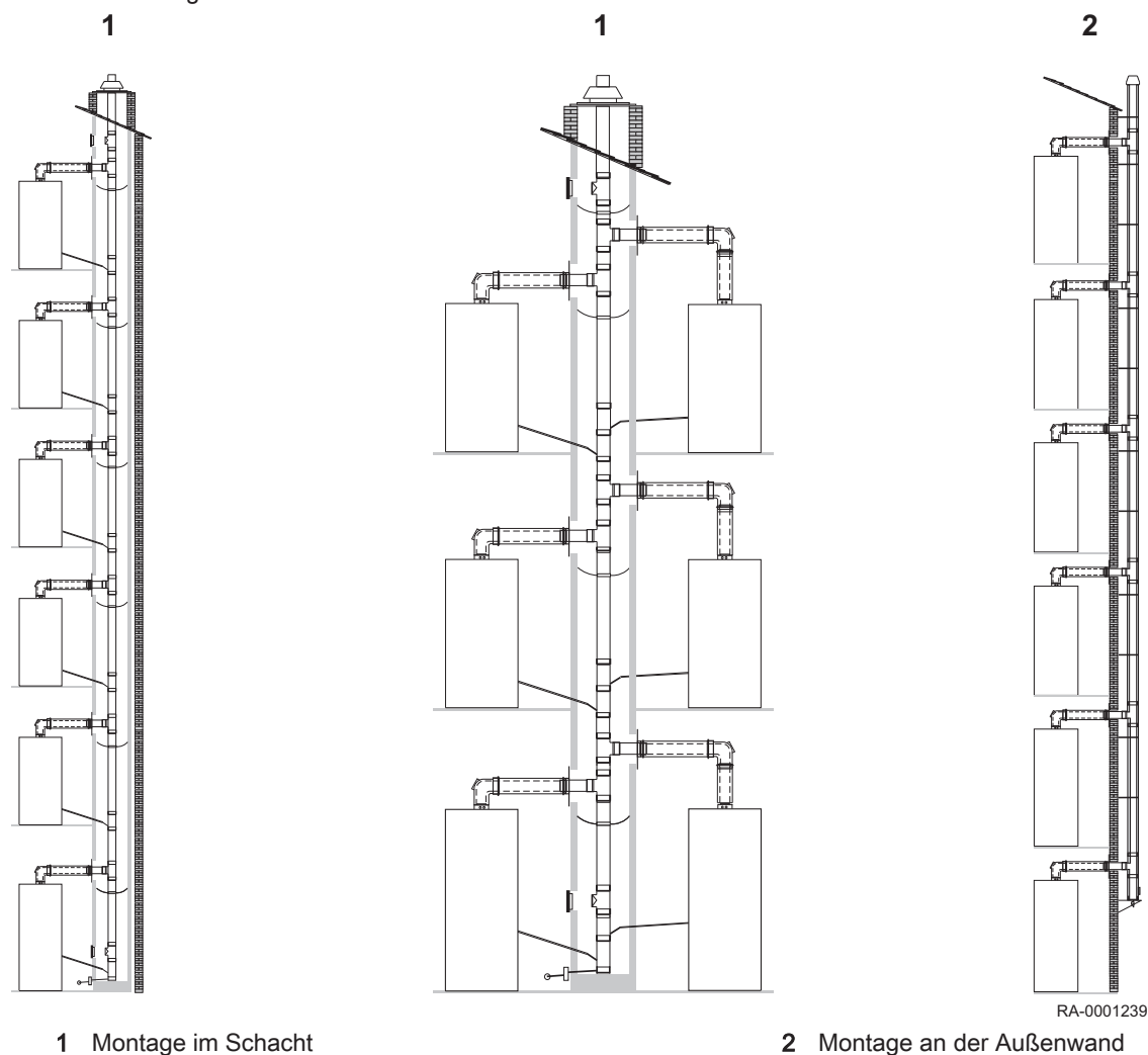
Abb.25 Montagearten
