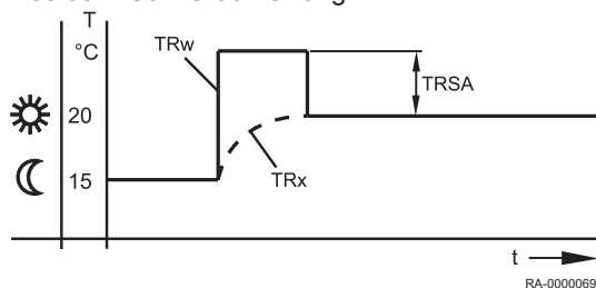
Abb.35 Schnellaufheizung
