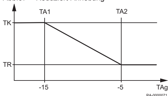
Abb.37 Reduziert-Anhebung
