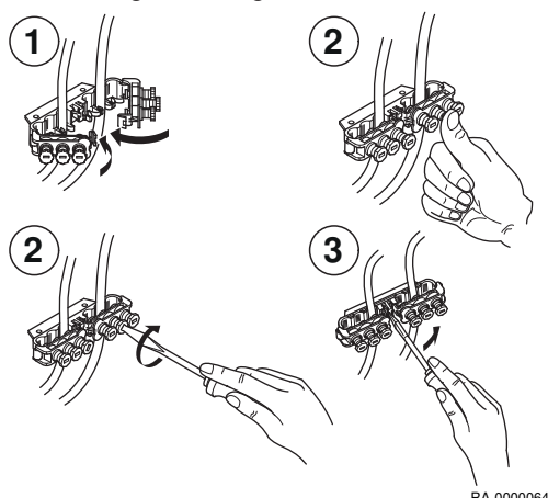
Abb.26 Zugentlastungen
