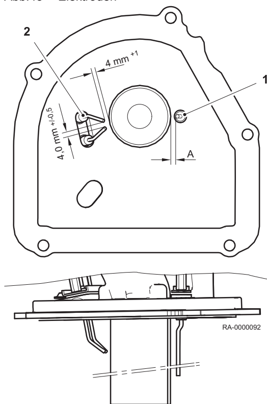
Abb.45 Elektroden
