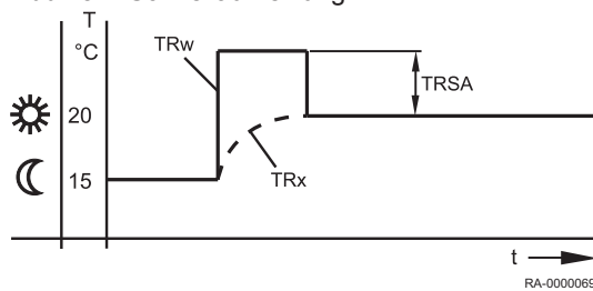
Abb.28 Schnellaufheizung
