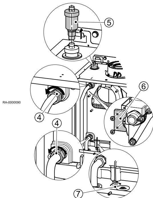
Abb.41 Wärmetauscher ausbauen
