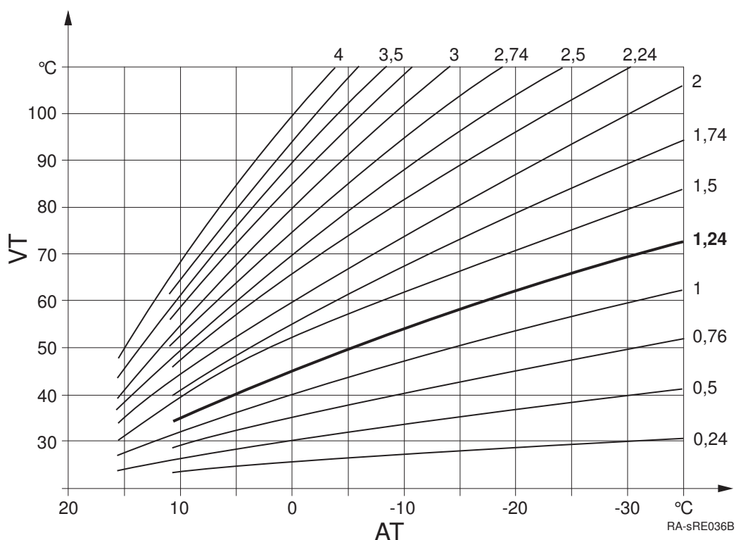
Abb.25 Heizkennlinien-Diagramm
