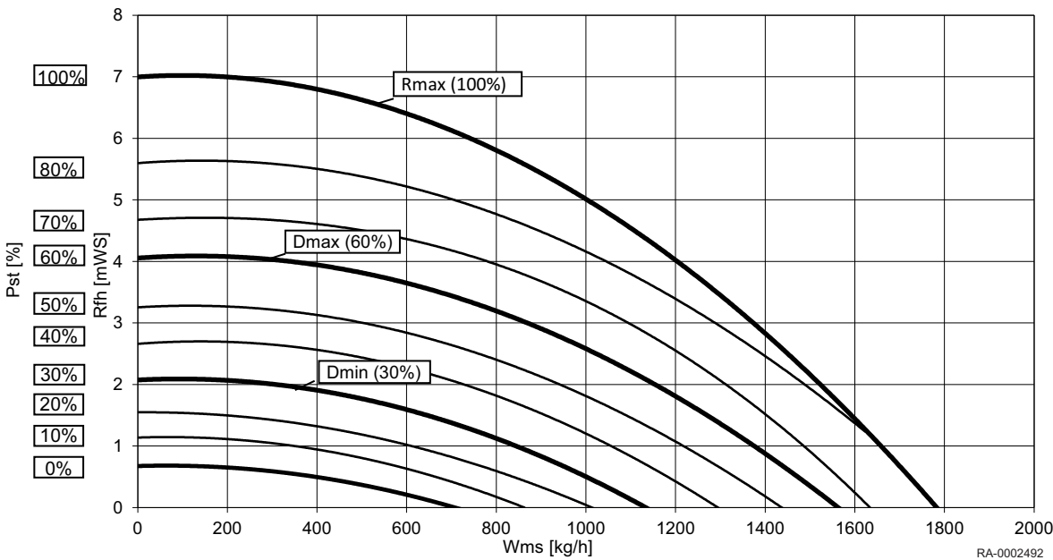
Abb.1 Restförderhöhe BBK EVO 20/22
