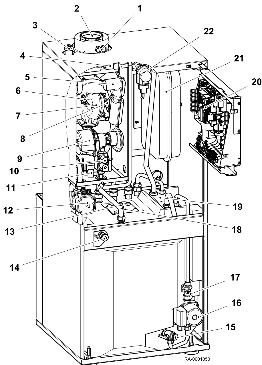
Abb.4 Kesselansicht BBK EVO (dargestellt ohne Vorderwand und Abdeckung der Regelung)
