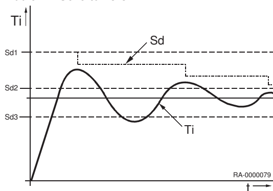
Abb.34 Schaltdifferenz
