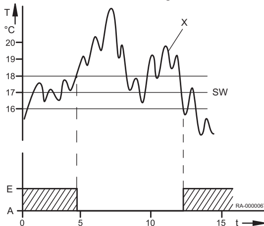
Abb.26 Sommer-/Winterheizgrenze
