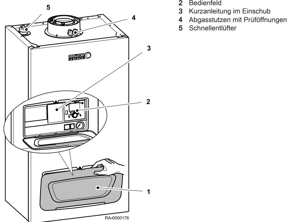
Abb.1 Übersichtszeichnung WGB
