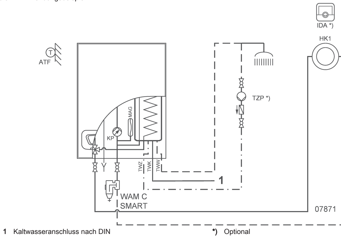
Abb.10 Anschlussplan
