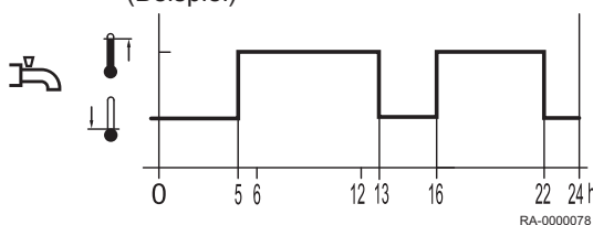
Abb.32 Freigabe nach Zeitprogramm 4 (Beispiel)
