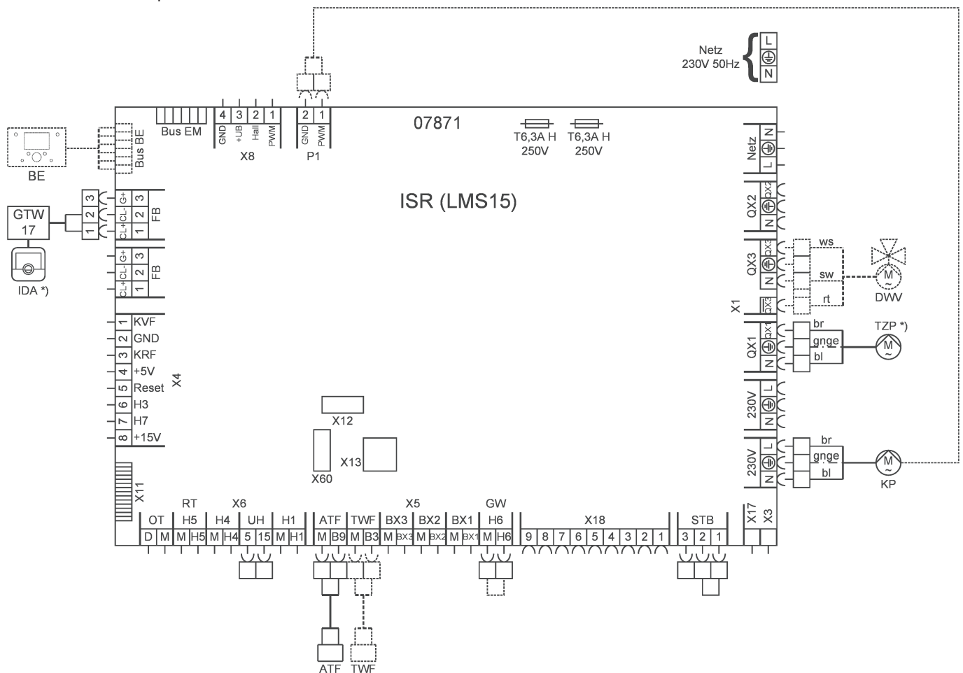
Abb.10 Anschlussplan
