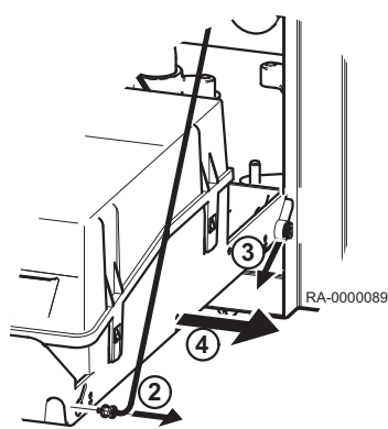
Abb.37 Kesselschaltfeld aushaken
