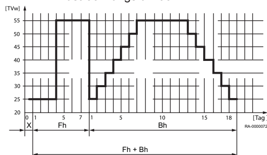
Abb.30 Temperaturprofil bei der Estrich-Austrocknungsfunktion
