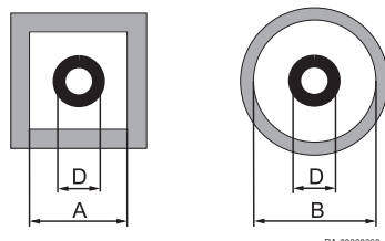
Abb.15 Mindestmaße des Schachtes
