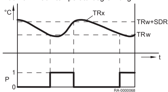
Abb.26 Raumtemperaturbegrenzung
