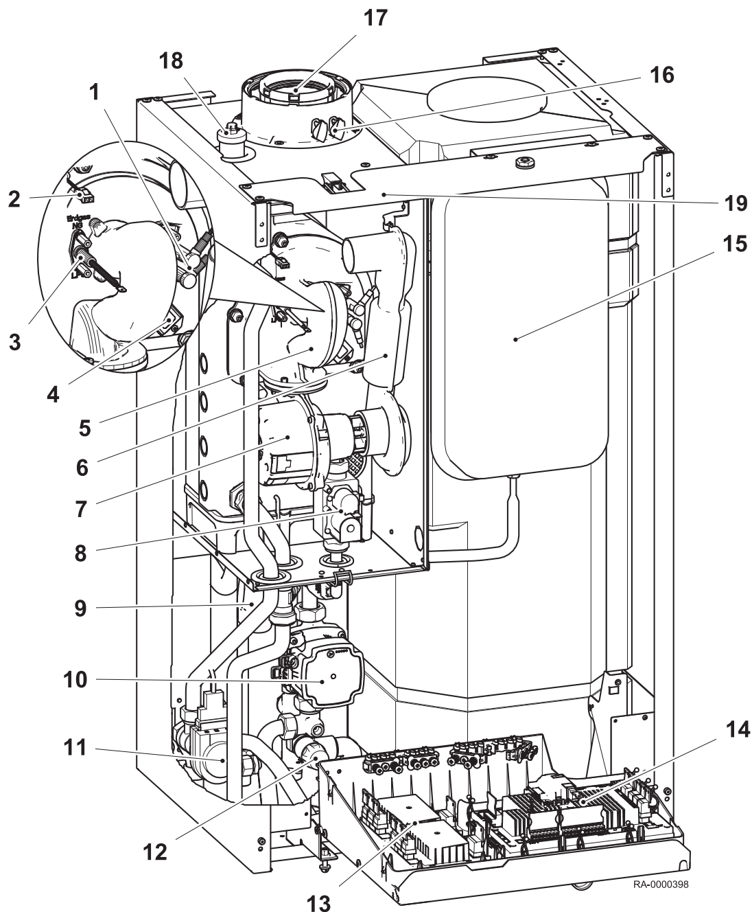
Abb.4 Kesselansicht WGB-K EVO (dargestellt ohne Vorderwand und Abdeckung der Regelung)
