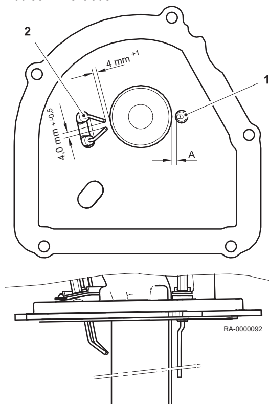
Abb.38 Elektroden
