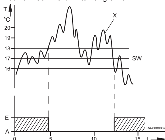
Abb.25 Sommer-/Winterheizgrenze
