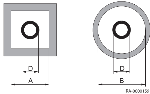
Abb.17 Mindestmaße des Schachtes
