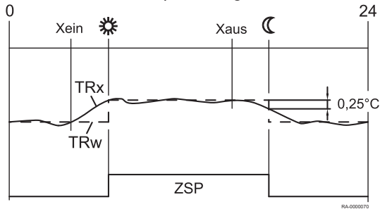
Abb.28 Einschalt- und Ausschaltoptimierung
