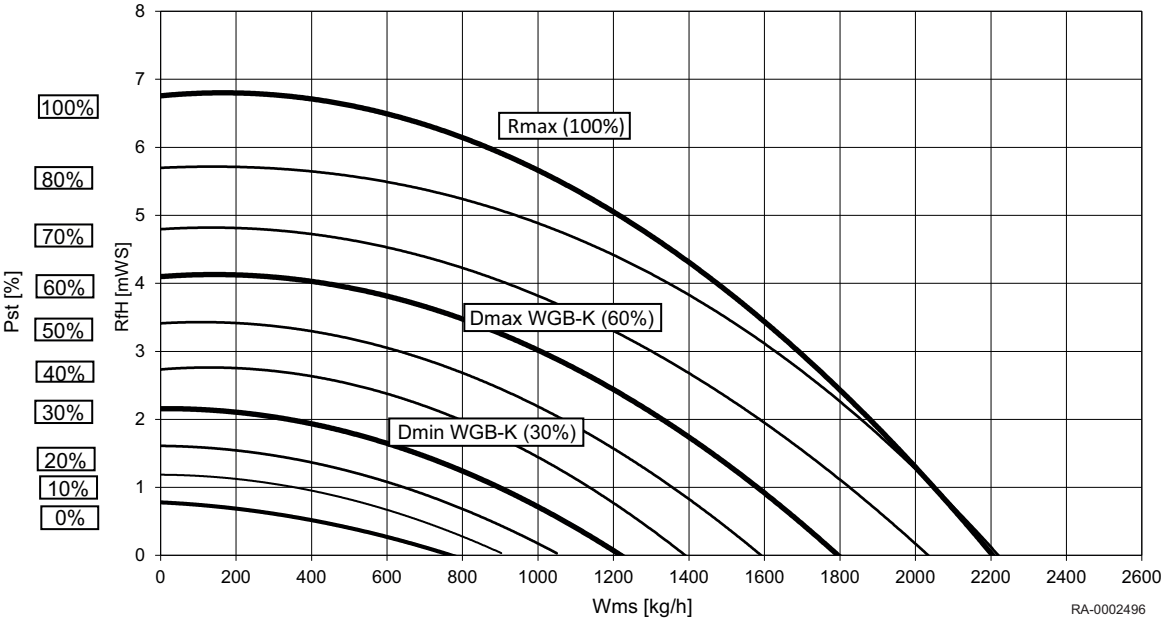
Abb.1 Restförderhöhe WGB-K EVO für Pumpenheizkreis
