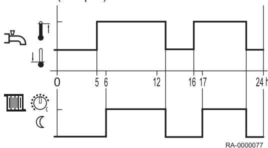
Abb.32 Freigabe nach Zeitprogramm 4 (Beispiel)
