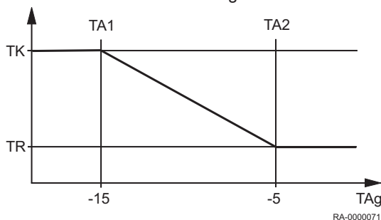
Abb.29 Reduziert-Anhebung
