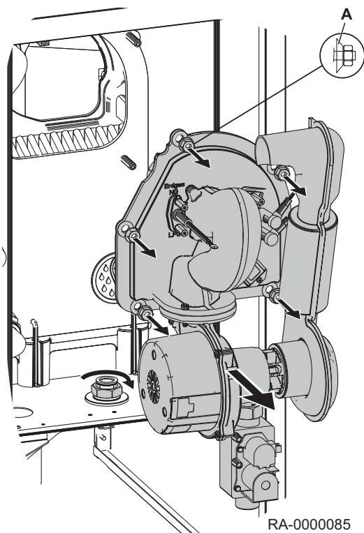
Abb.40 Gasbrenner ausbauen
