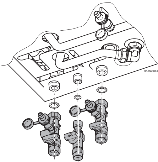
Abb.11 Einbau Absperrventile
