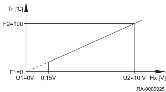
Abb.34 Spannungswert/Funktionswert
