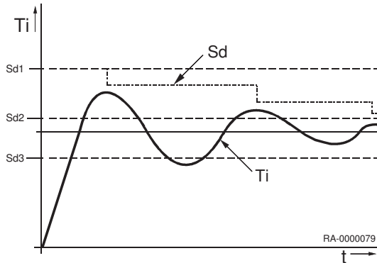
Abb.33 Schaltdifferenz
