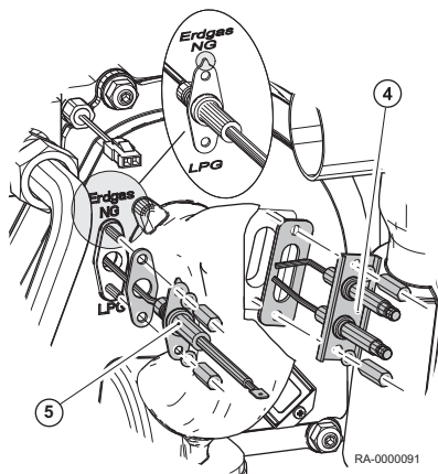
Abb.39 Zünd- und Ionisationselektrode ausbauen
