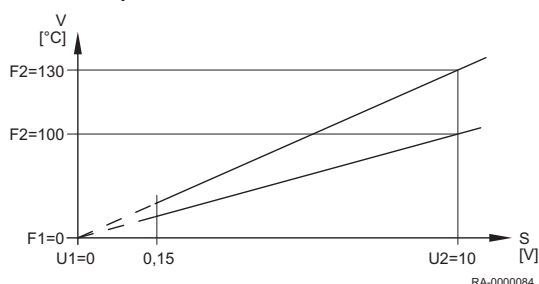
Abb.36 Beispiel für Wärmeanforderung 10 V
