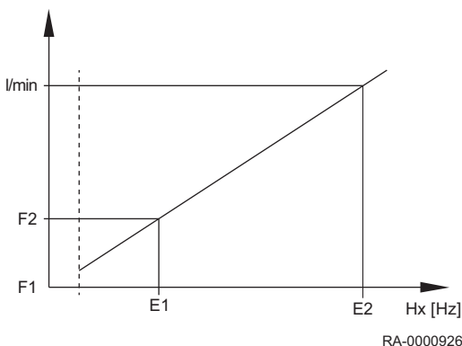
Abb.35 Beispiel für zwei unterschiedliche Fühlerkennlinien
