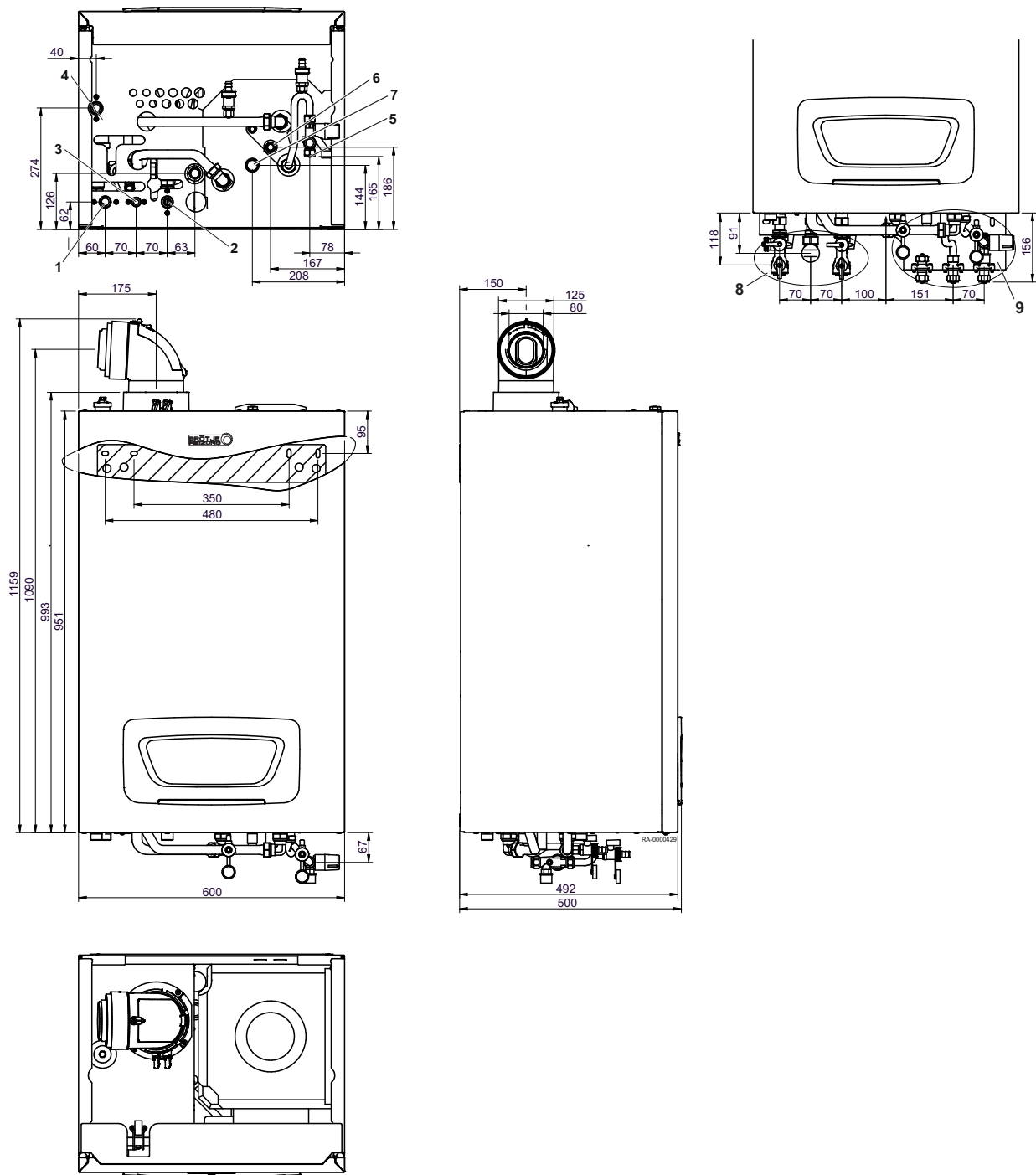
Abb.2 Abmessungen und Anschlüsse WGB-K EVO
