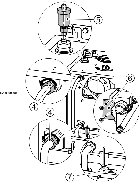
Abb.41 Wärmetauscher ausbauen
